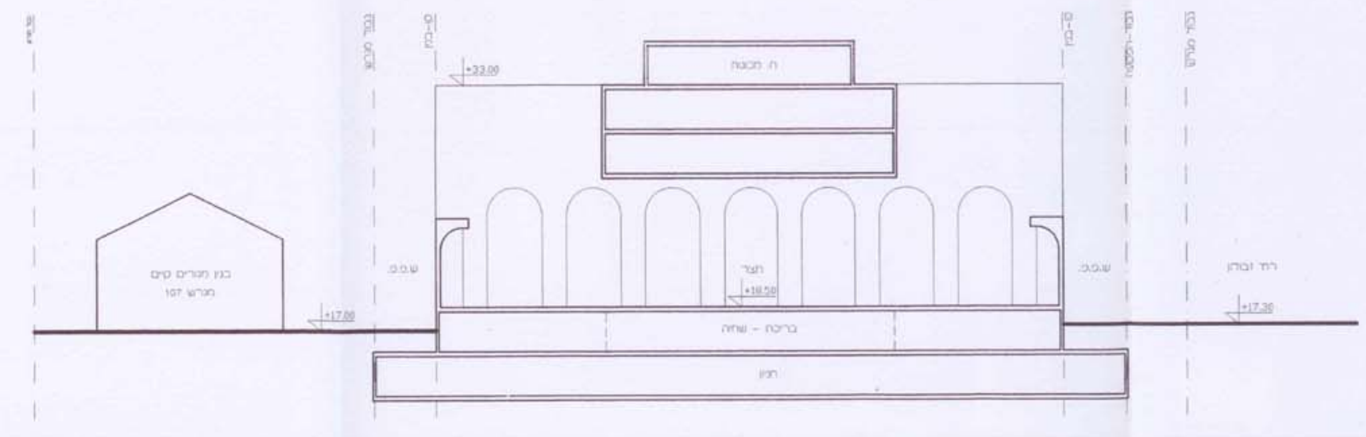
חצר ב-ב צפון-דרום ק.מ. 1:250
