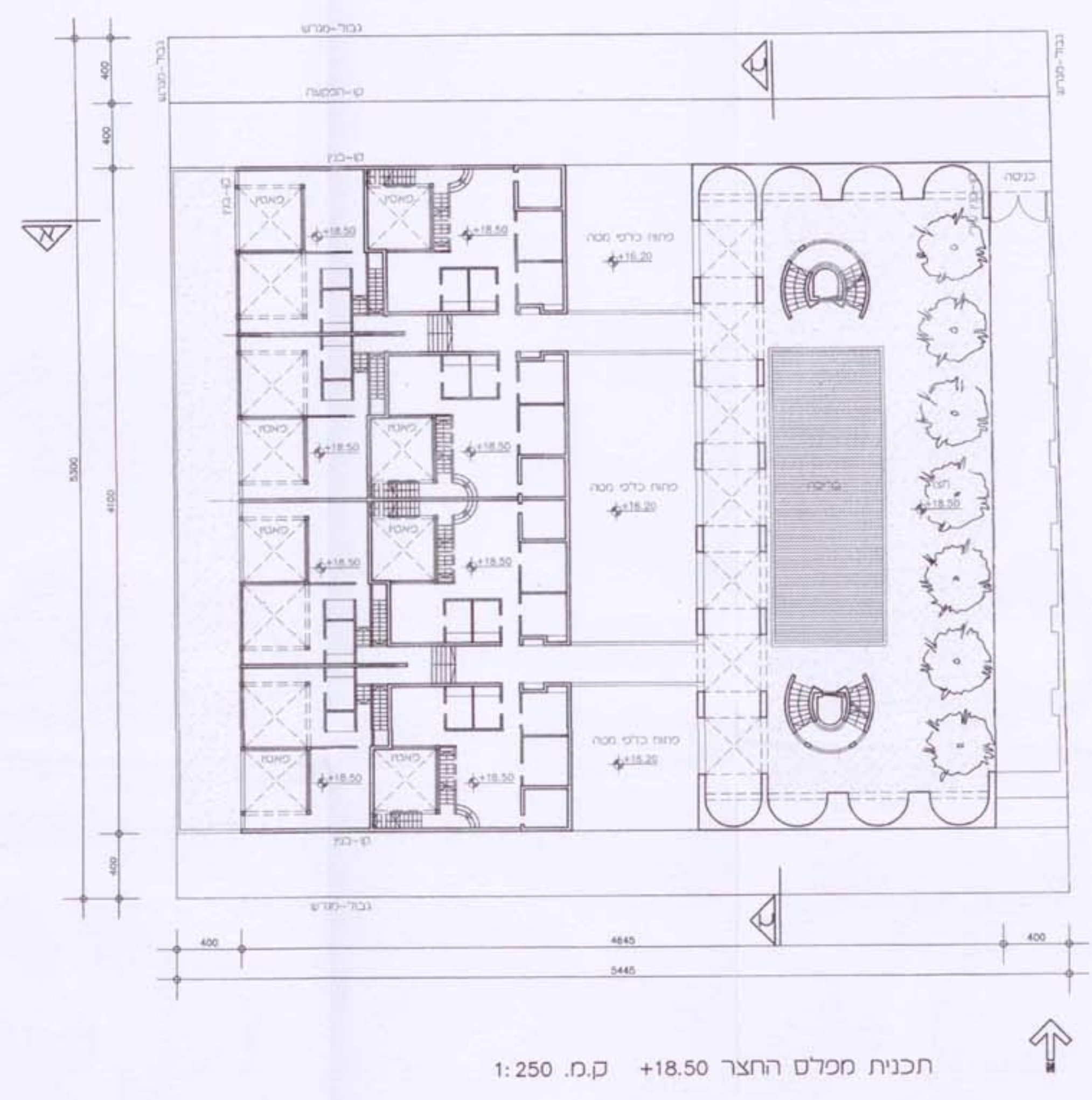
תכנית מכלס החצר +18.50 ק.מ. 1:250
