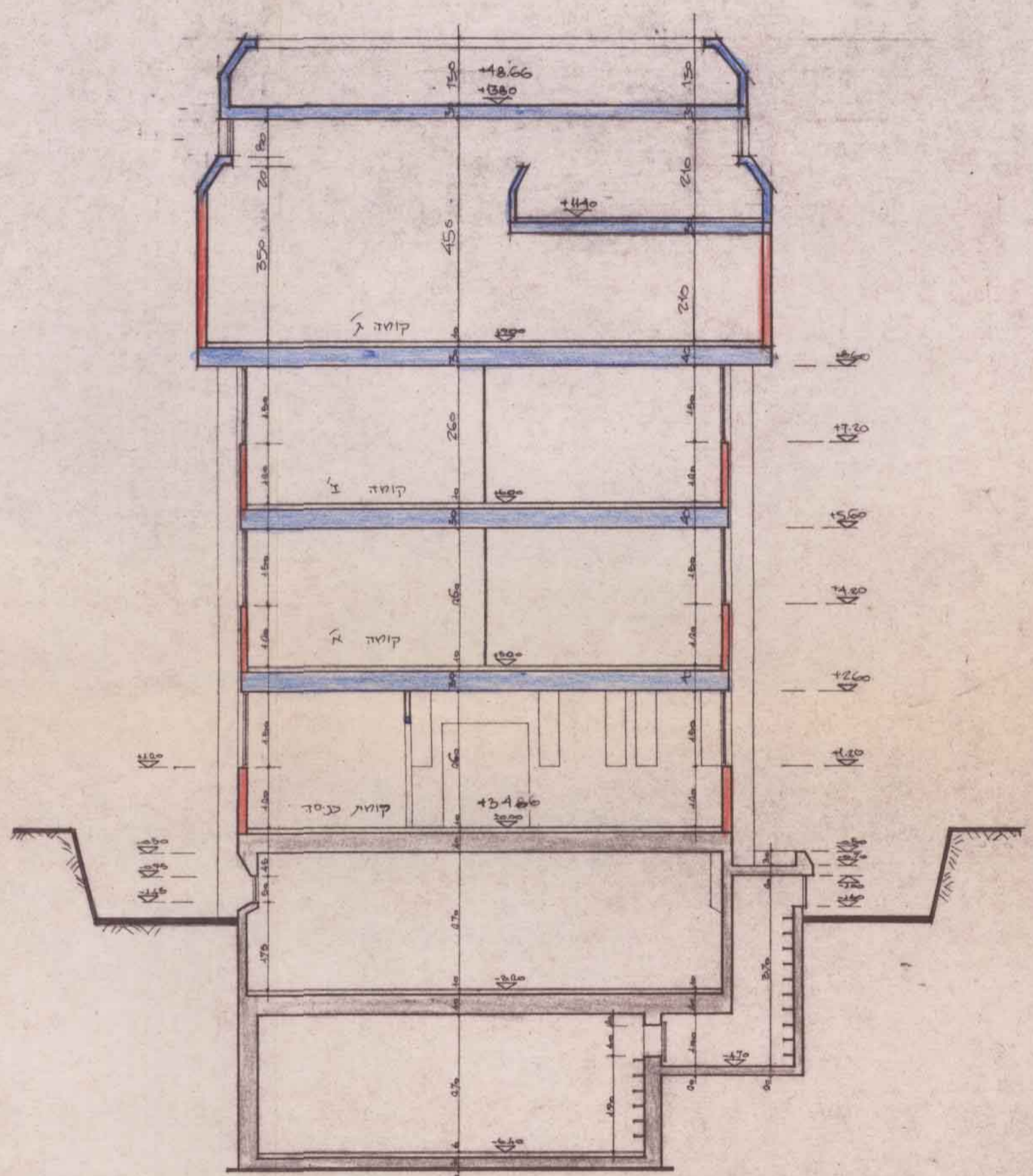
צנף ב-ב
