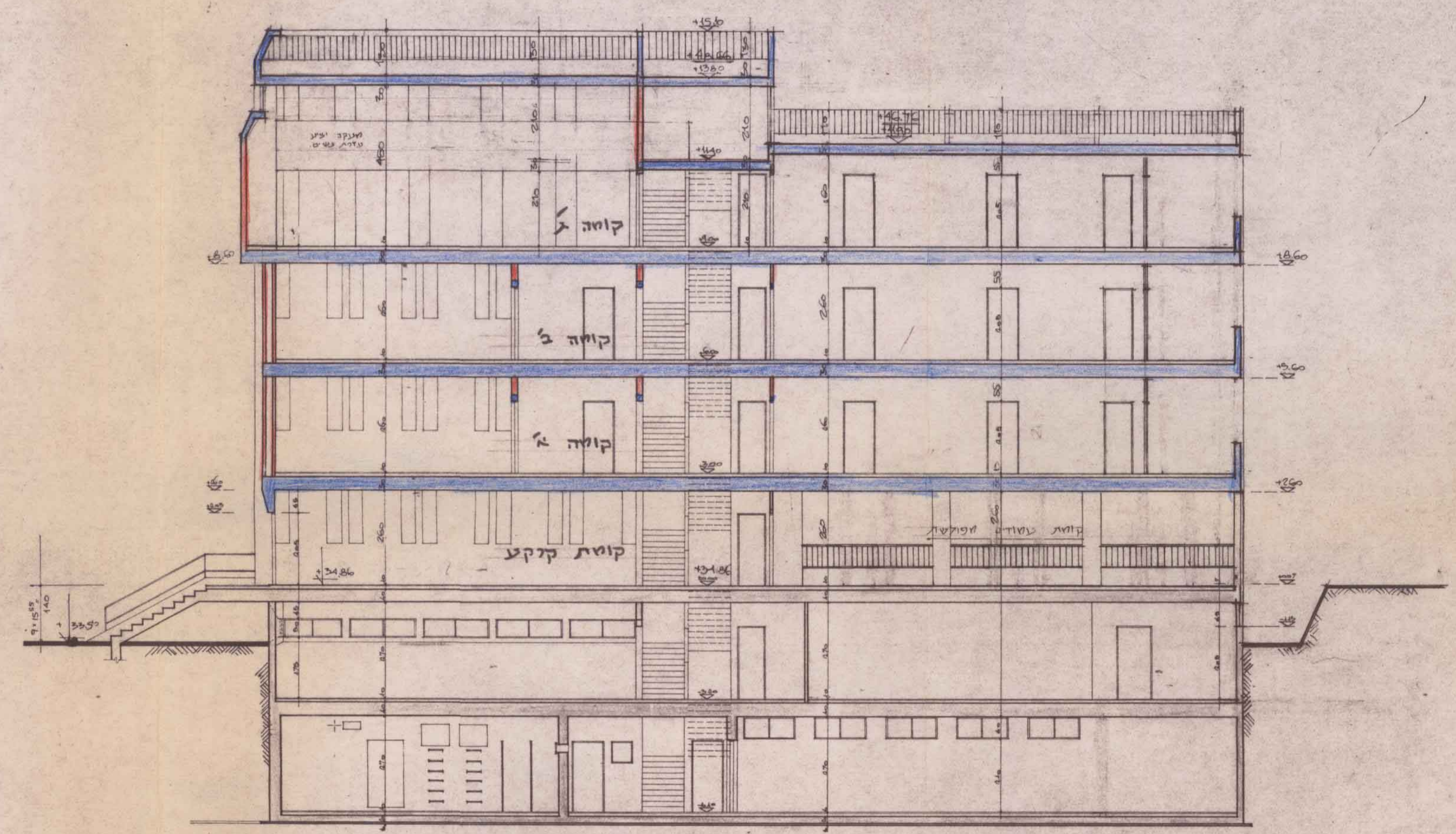
צנף ג-ג 1:100
