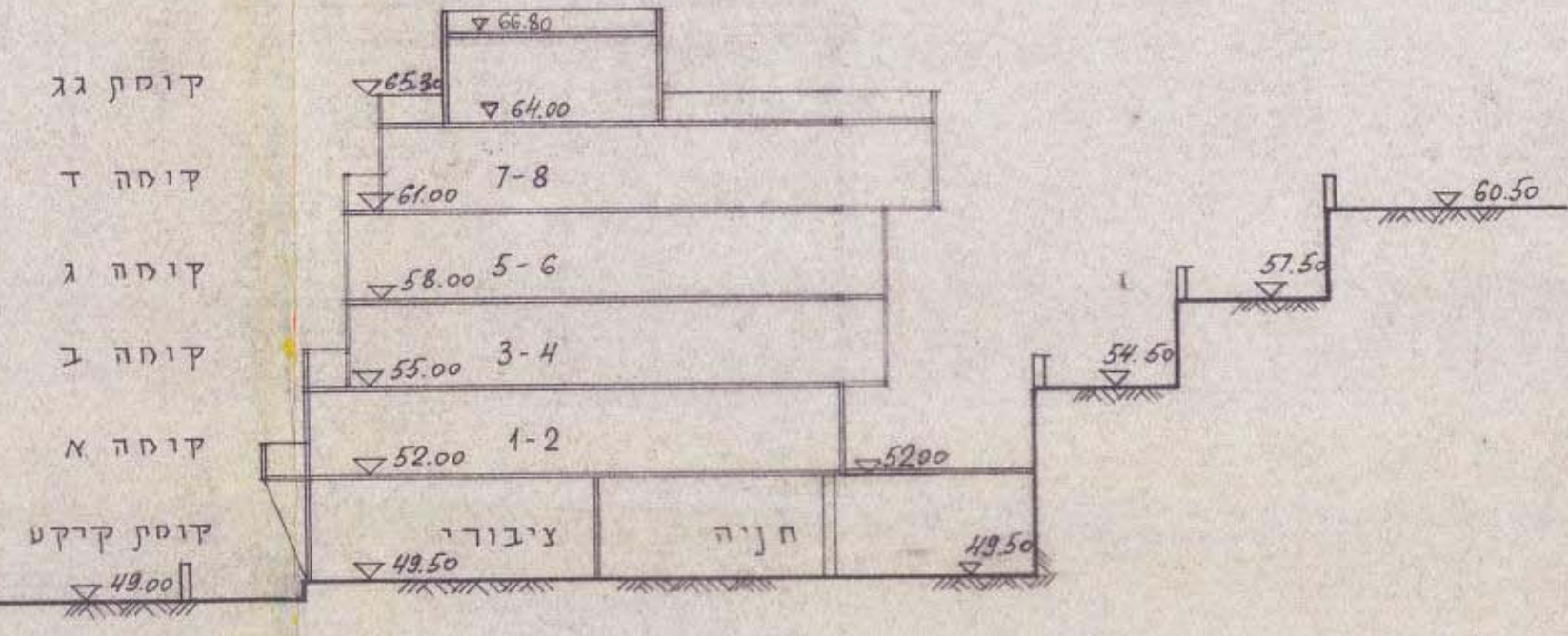
חתך א-א חלקה 239
