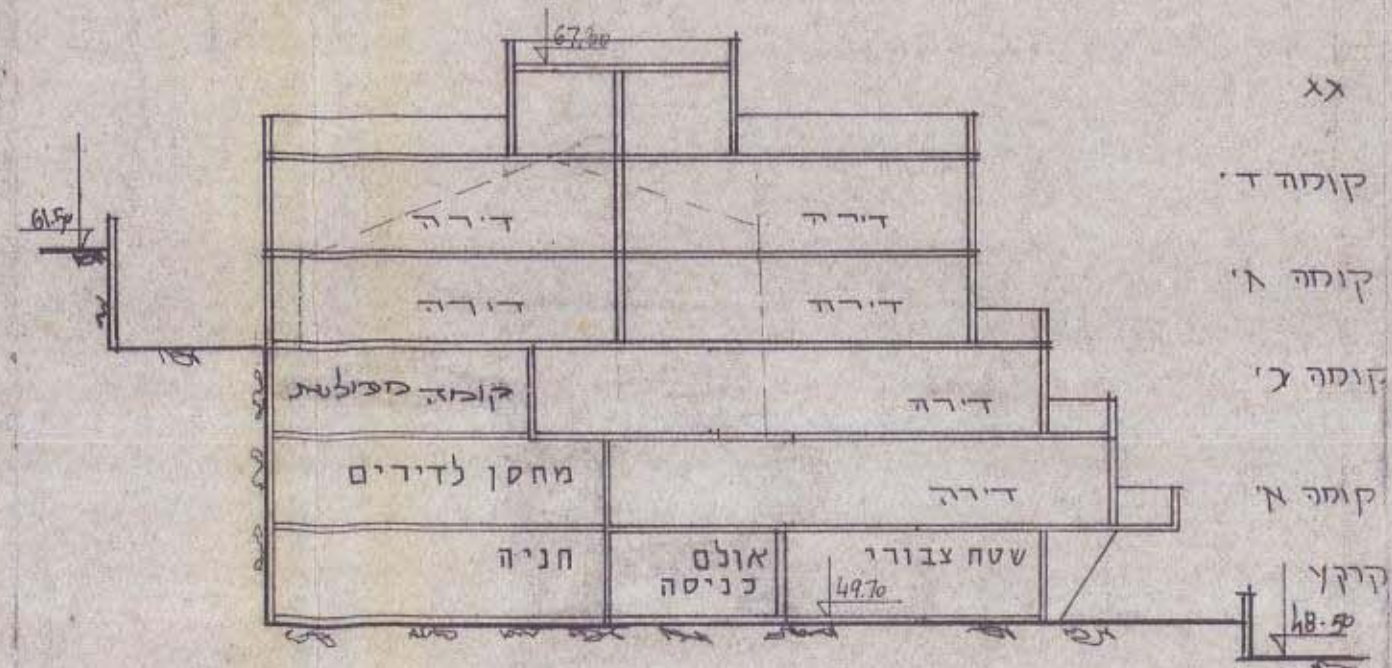
חתך ב-ב חלקה 236
