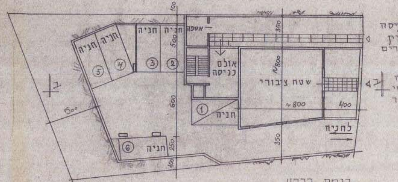
קומה קרקע חלקה 236
