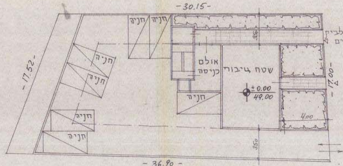
תוכנית קו סדה קרקע חלקה 238
