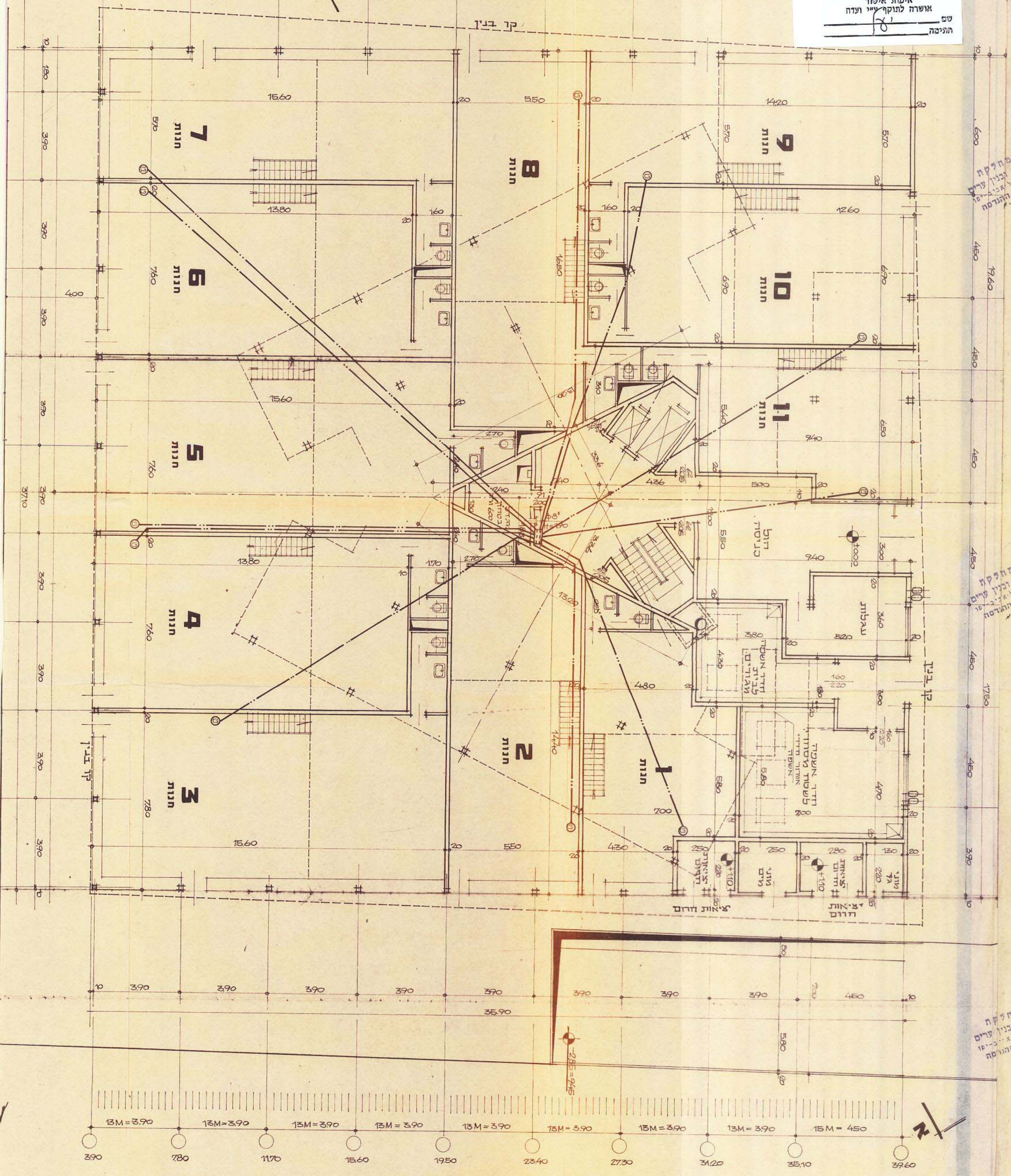
תכנית קומת קרקע - ק.מ. 1:100
