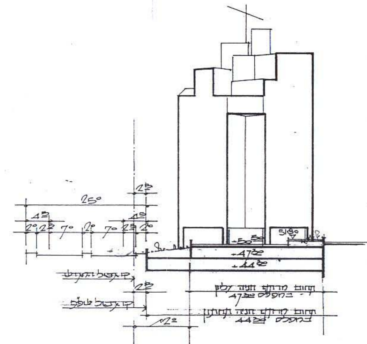
חתך ד-ד
