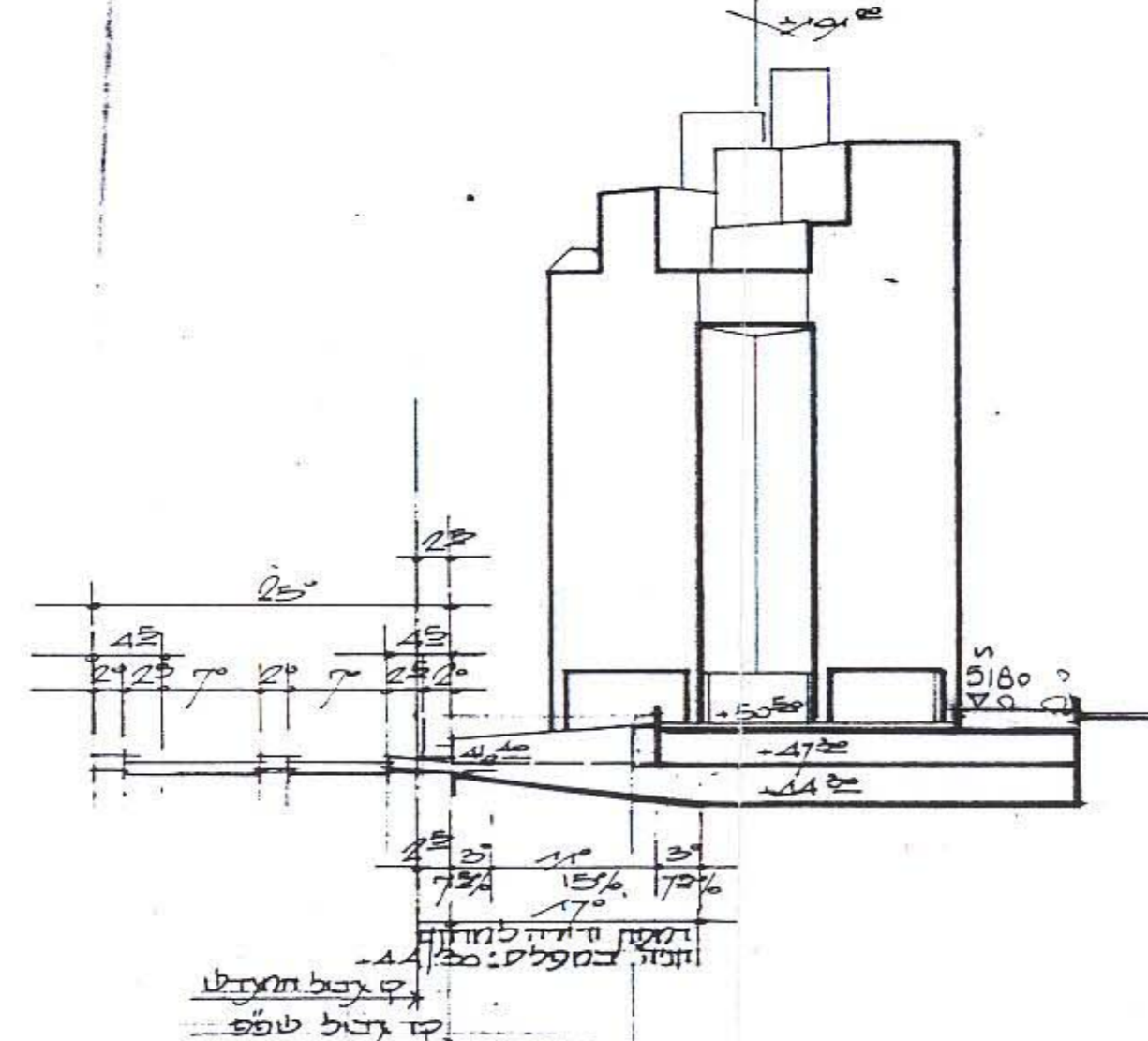
חתך ג-ג
