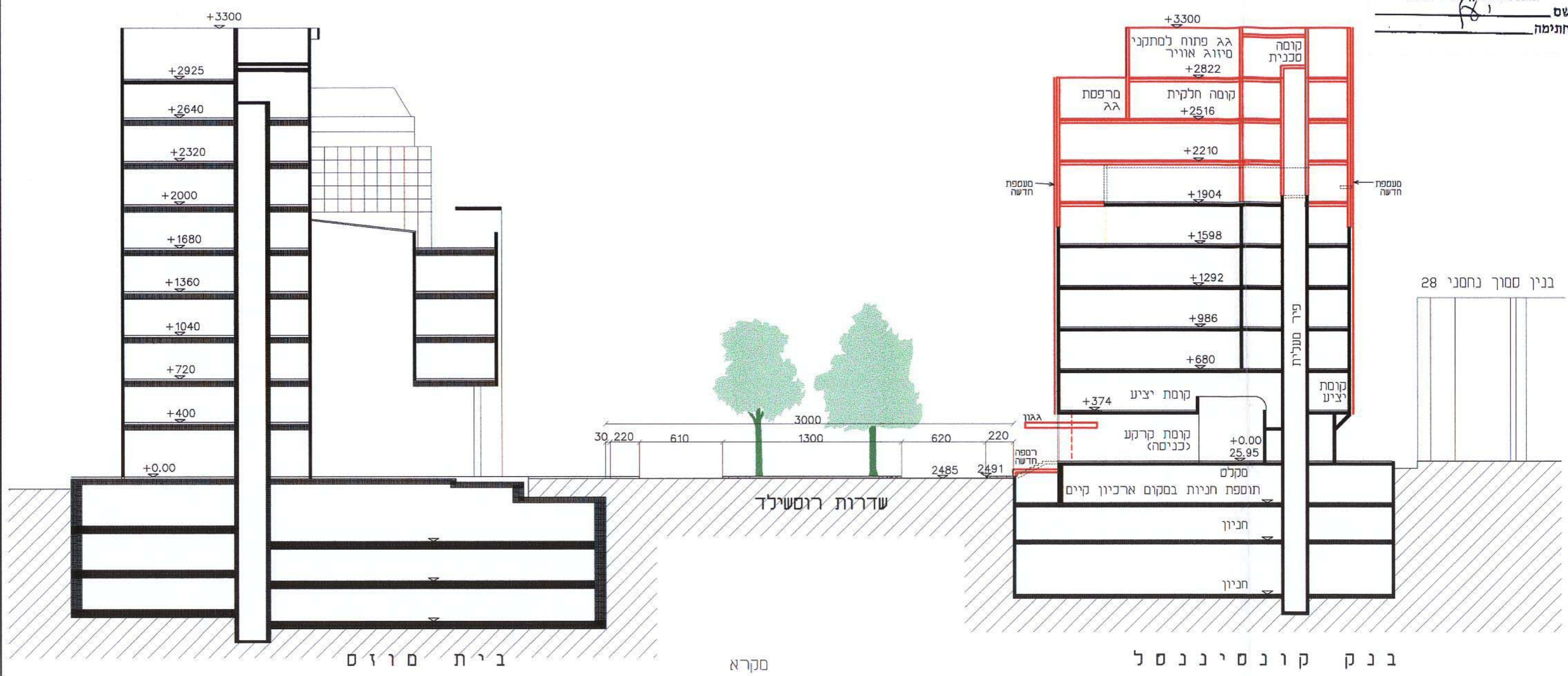
ניספח בינוי - חתך ק.מ. 1:250
