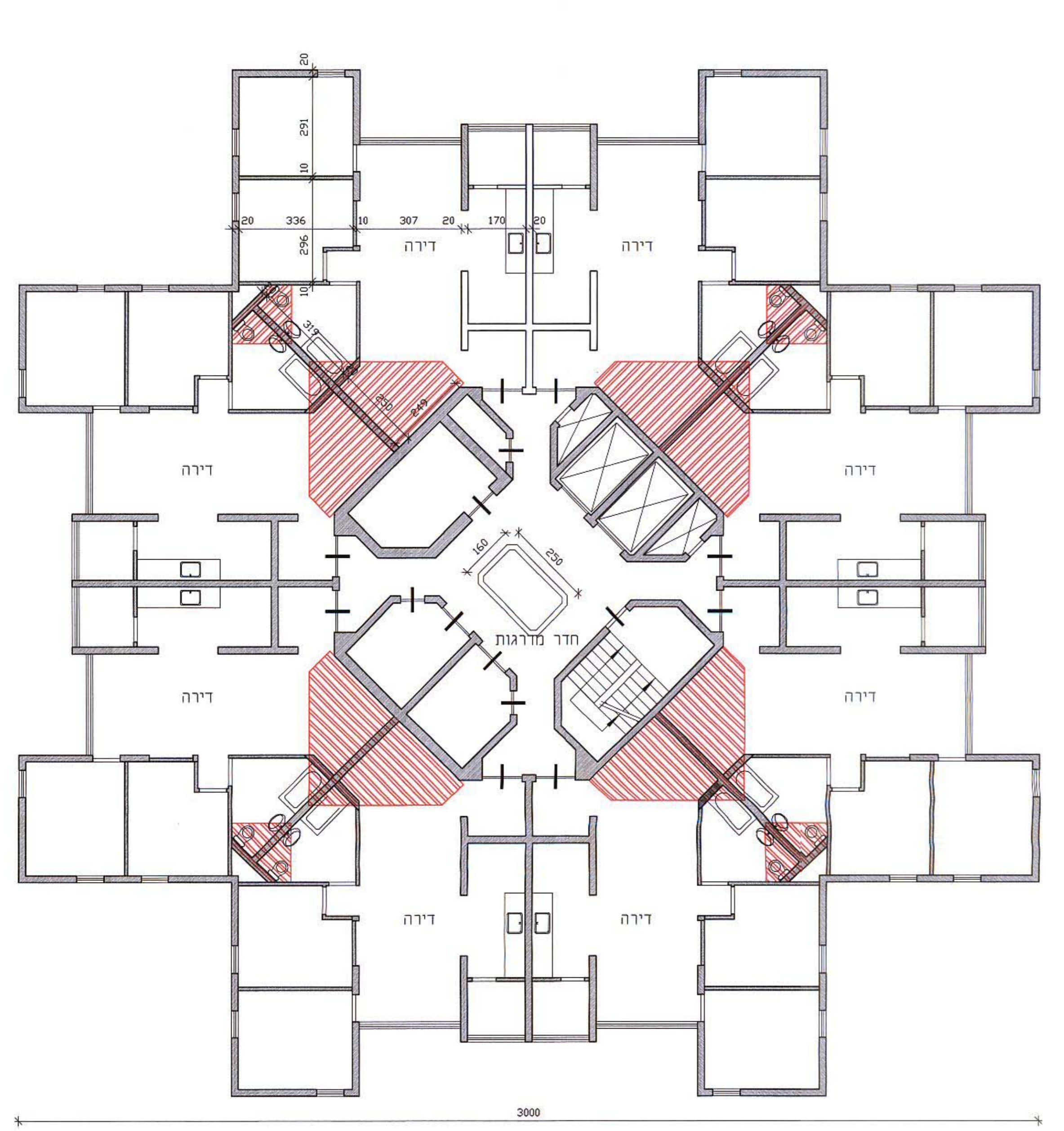
תכנית קומה טיפוסית
