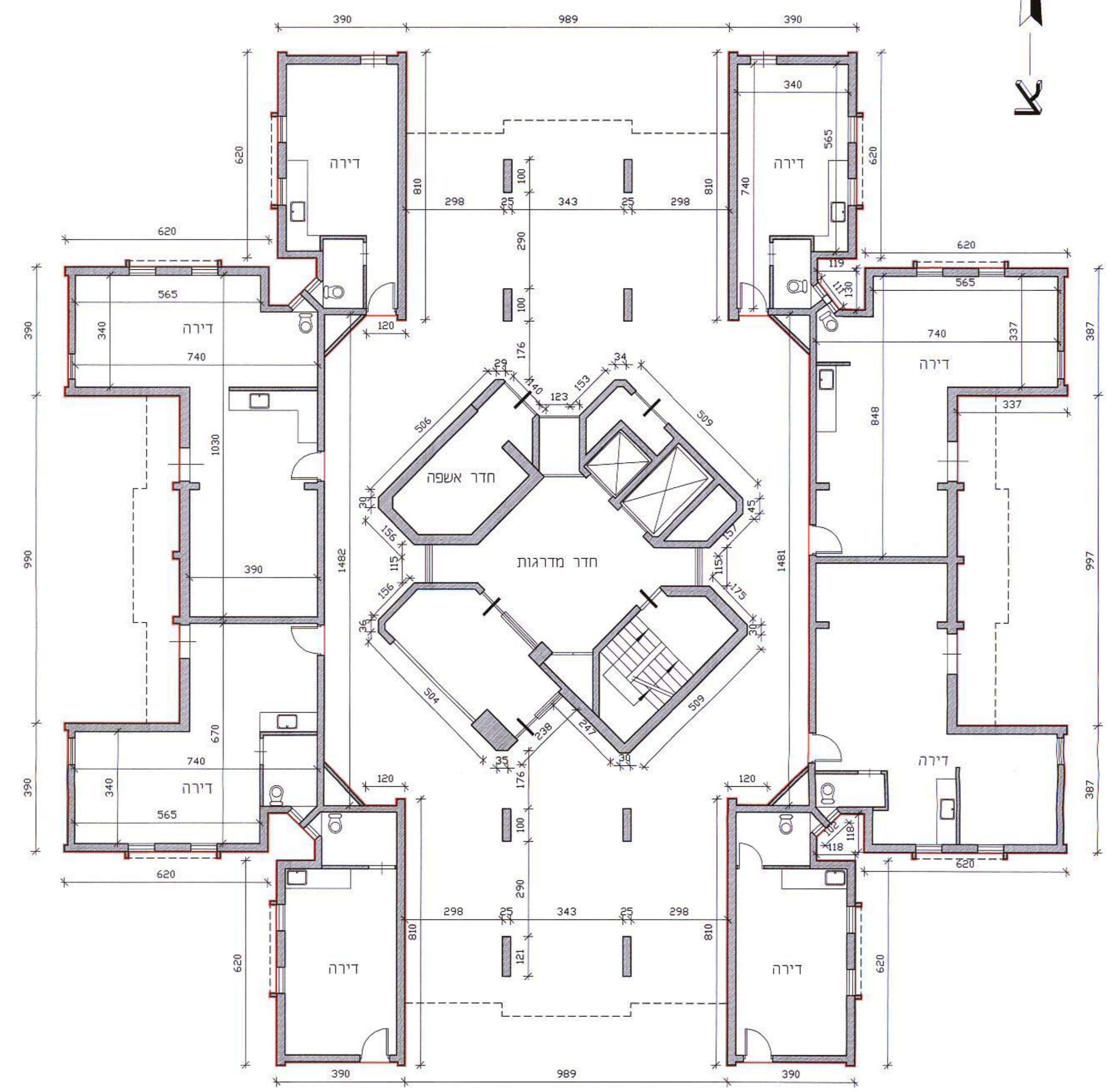
תכנית קומת קרקע
