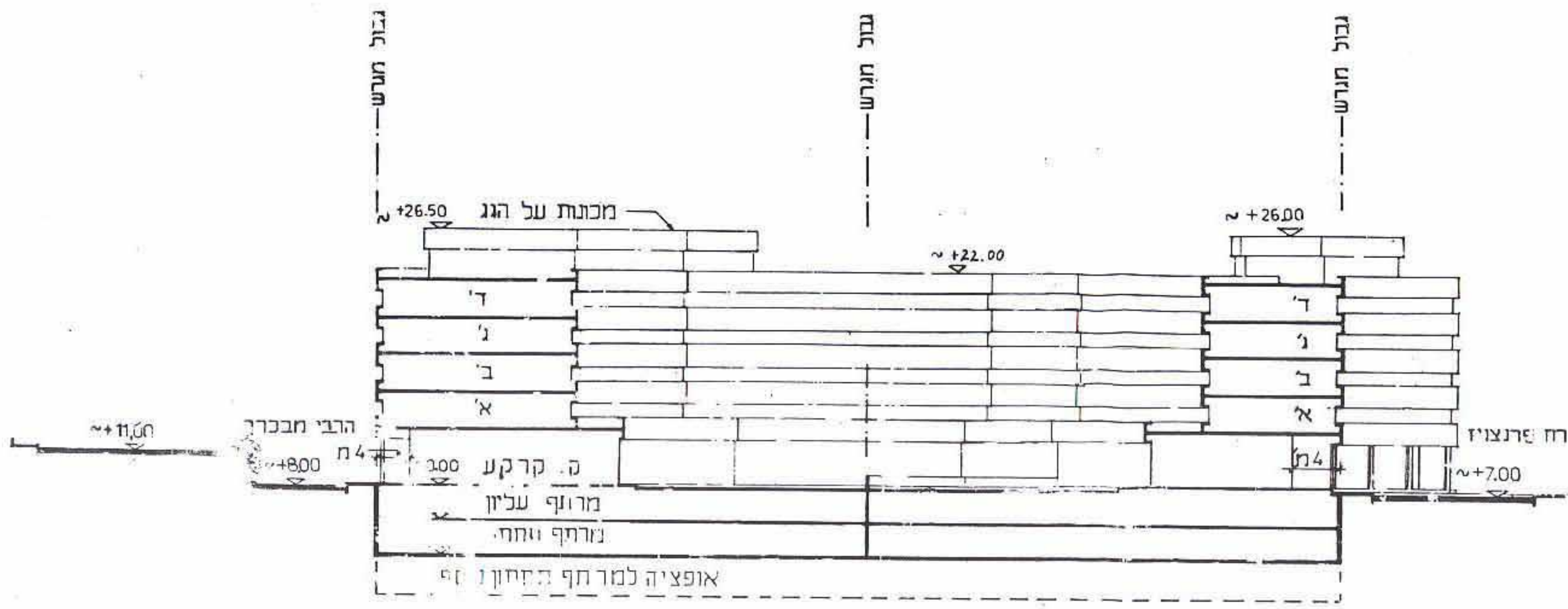
חתך א-א 1:500
