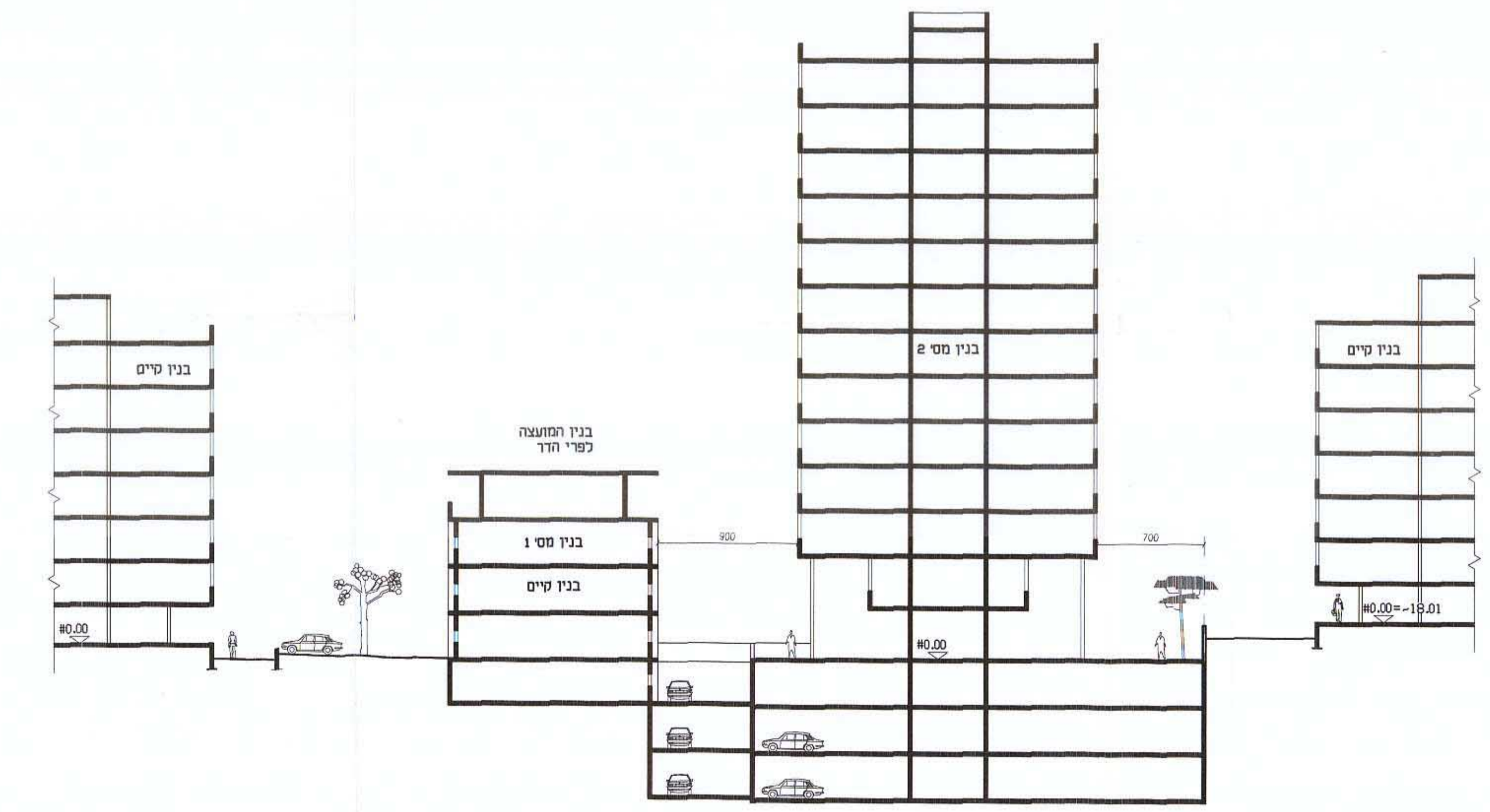
חותך 2-2 ק"מ 1:250
