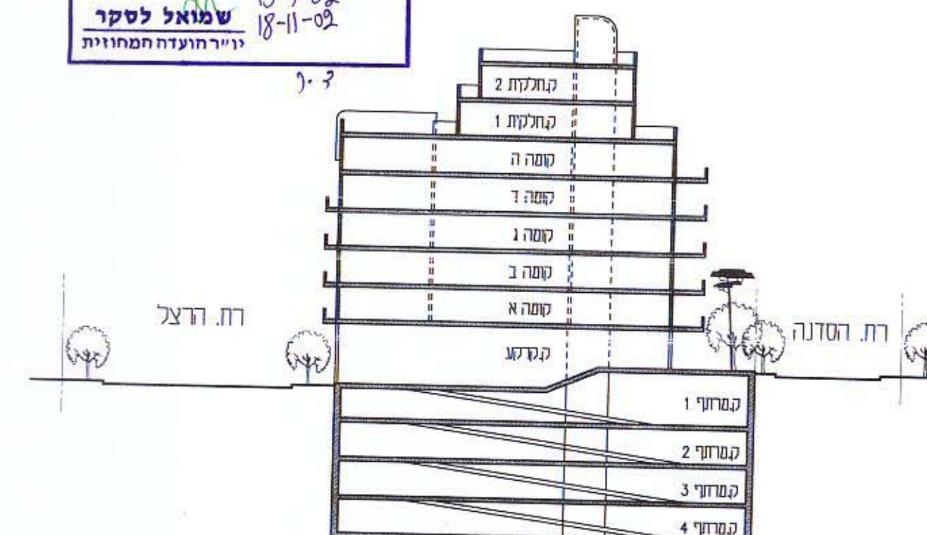
חתך רוחב - בין רחובות הרצל והסדנה 1:500
