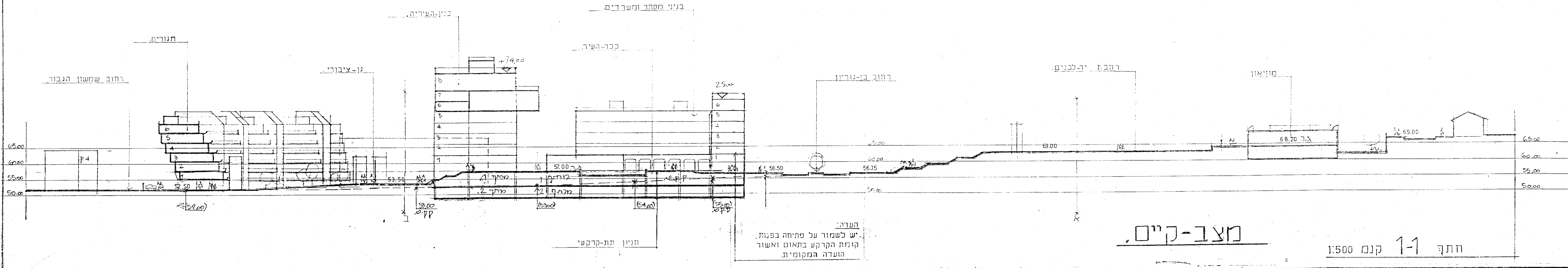
חתך 22 קנמ 1:500
