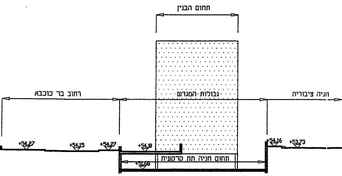
חתך לרוחב רחוב בר-כוכבא ק.מ. 1:250
