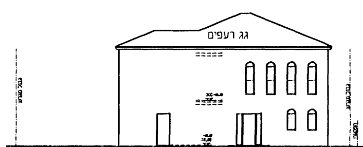
חזית מערבית קנימ 1:250
