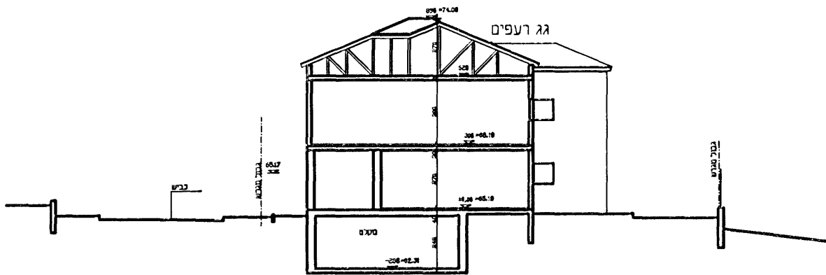
חתך ב-ב קנימ 1:250
