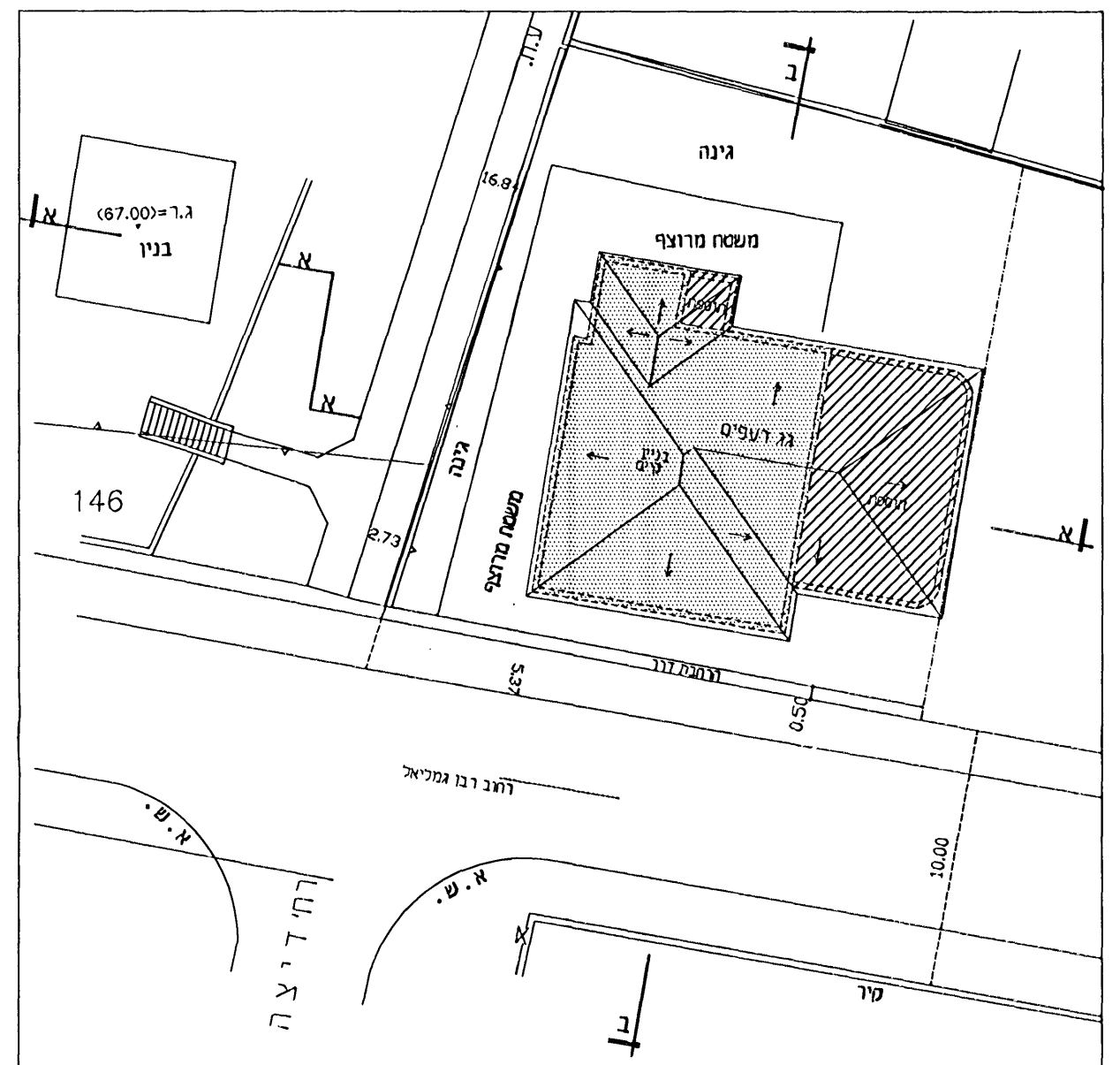
תכנית גגות קנימ 1:250
