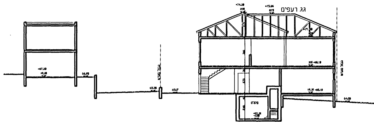
חתך א-א קנימ 1:250
