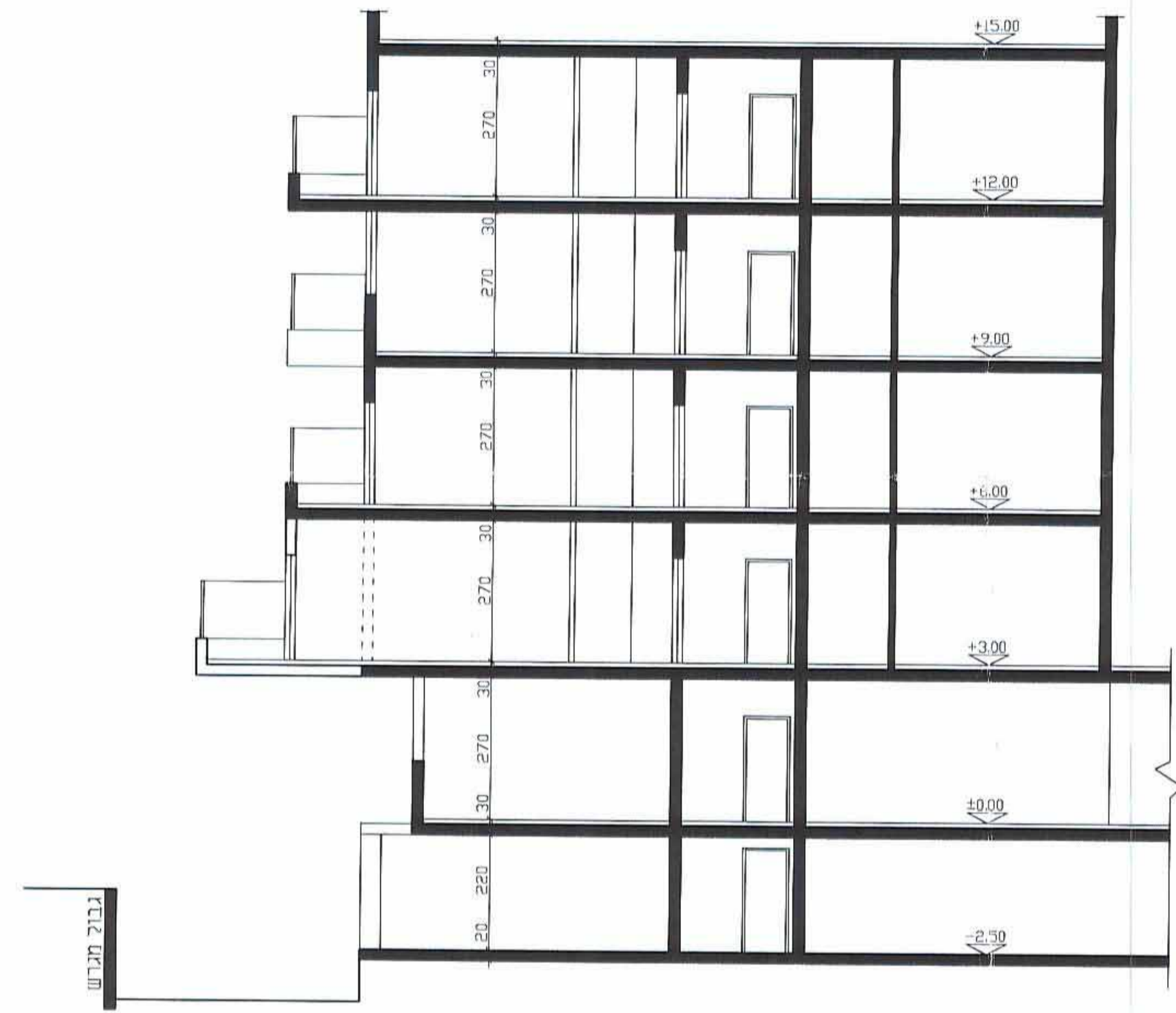
תכנית חתך א-א 1:100
