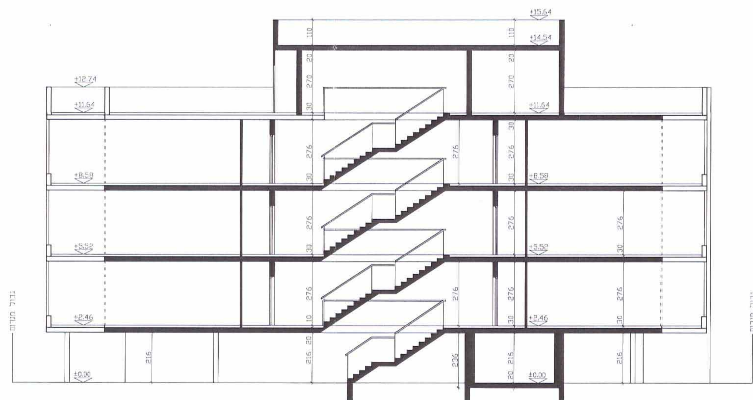
חתך א'-א' ק"נ 1:100
