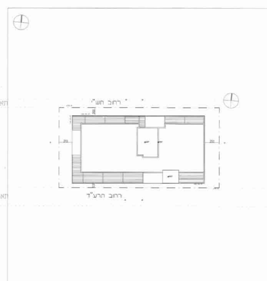
תכנית קומת גג עליזון 1:250
