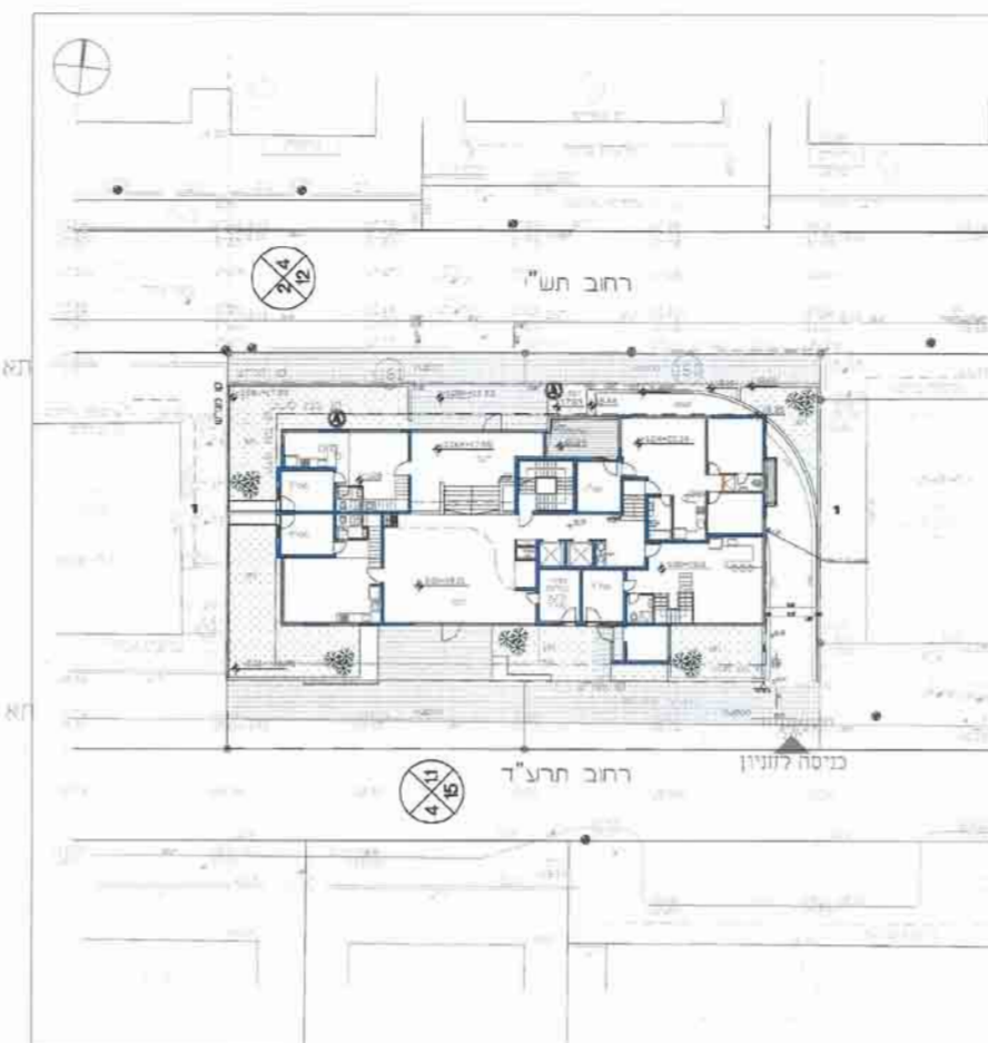
תכנית קומת קרקע 1:250
