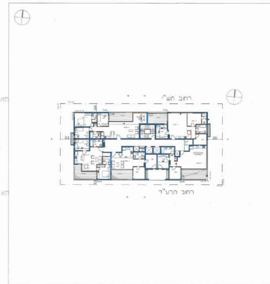
תכנית קומה 2-8 1:250
