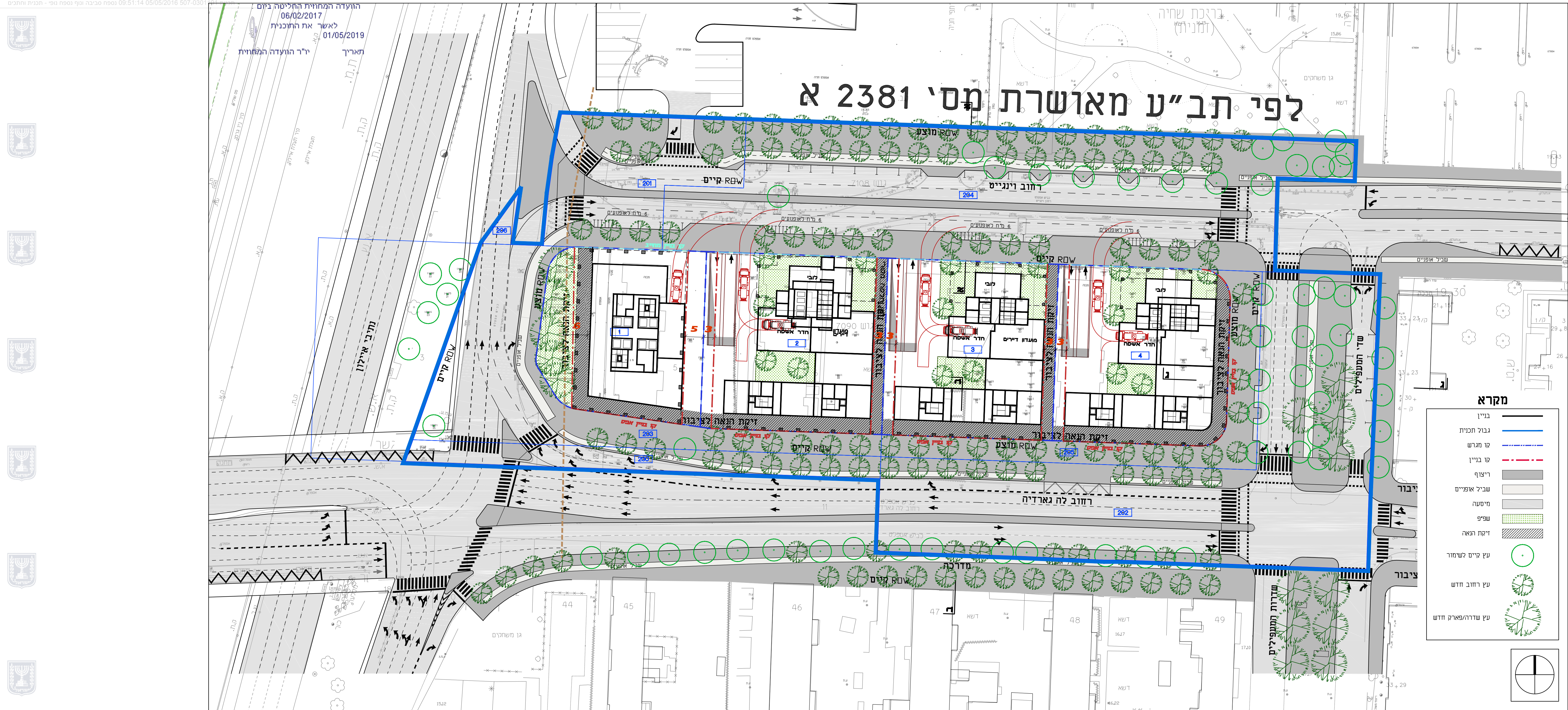
תכנית פיתוח נופי - קנ"מ 1:500
