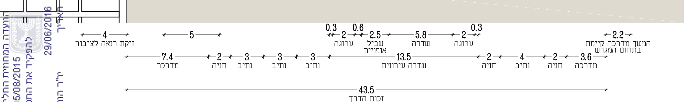
חתך אופייני ג-ג - רחוב המעפילים קנ"מ 1:200
