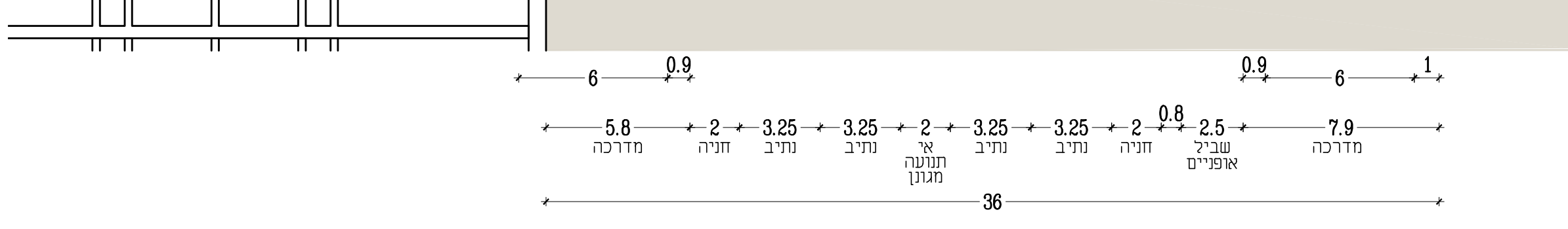
חתך אופייני א-א - רחוב וינגייט קנ"מ 1:200
