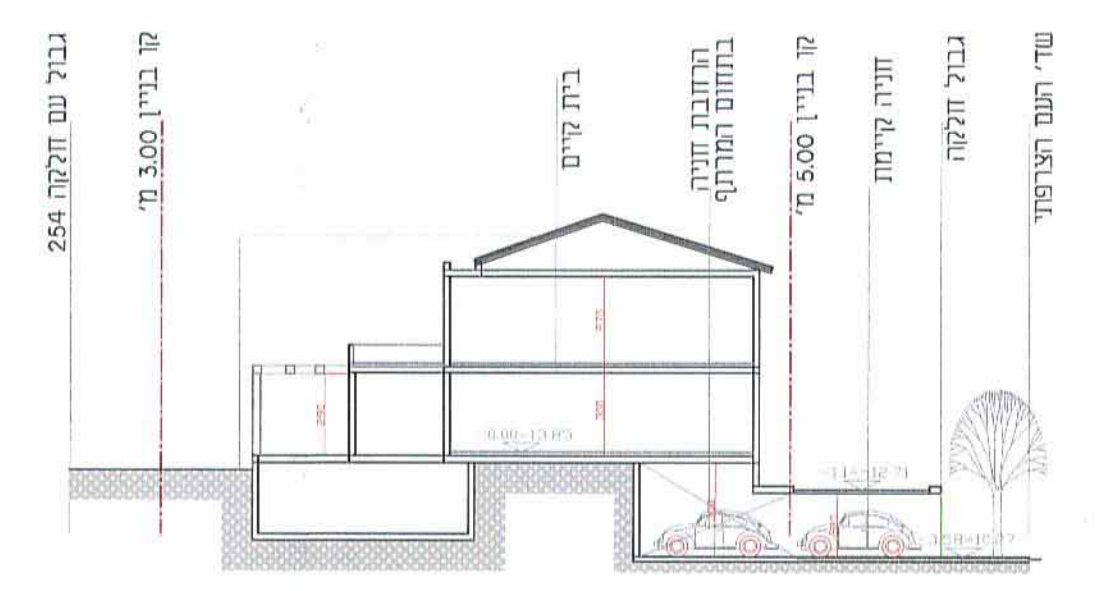
חותך א-א קני"מ 1:250
