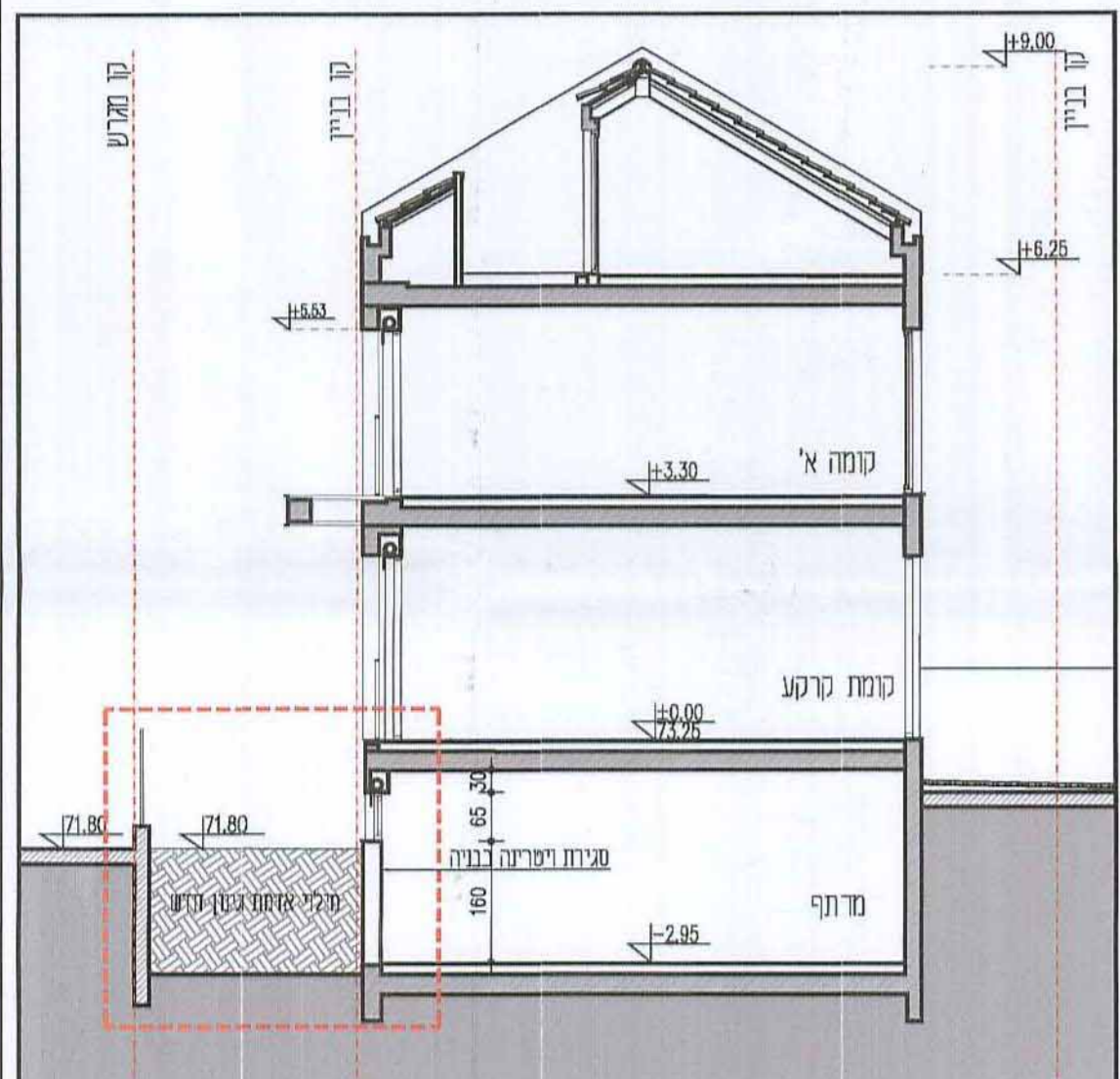
חתך עקרוני קנ"מ 1:100
