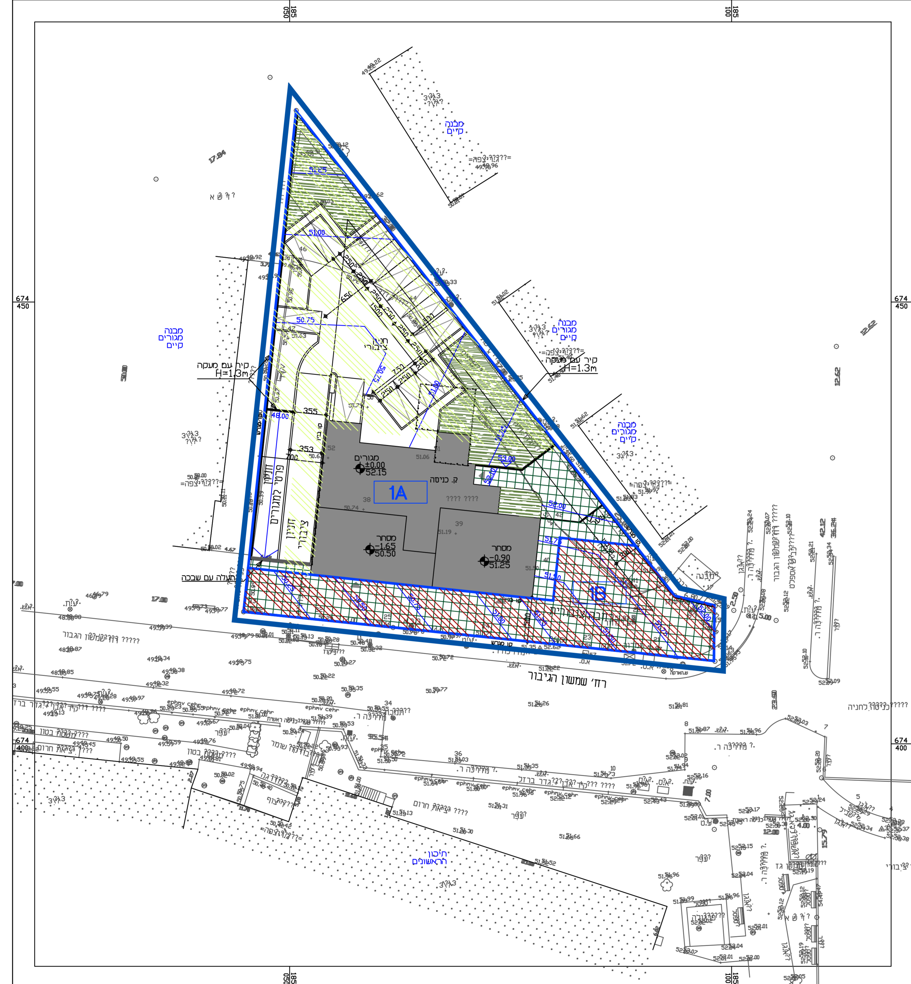
תכנית קומות קרקע קנ"מ 1:250
