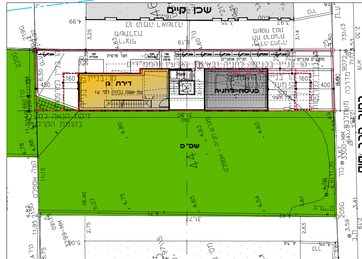
תכנית העמדה (קומת קרקע) 1:250
