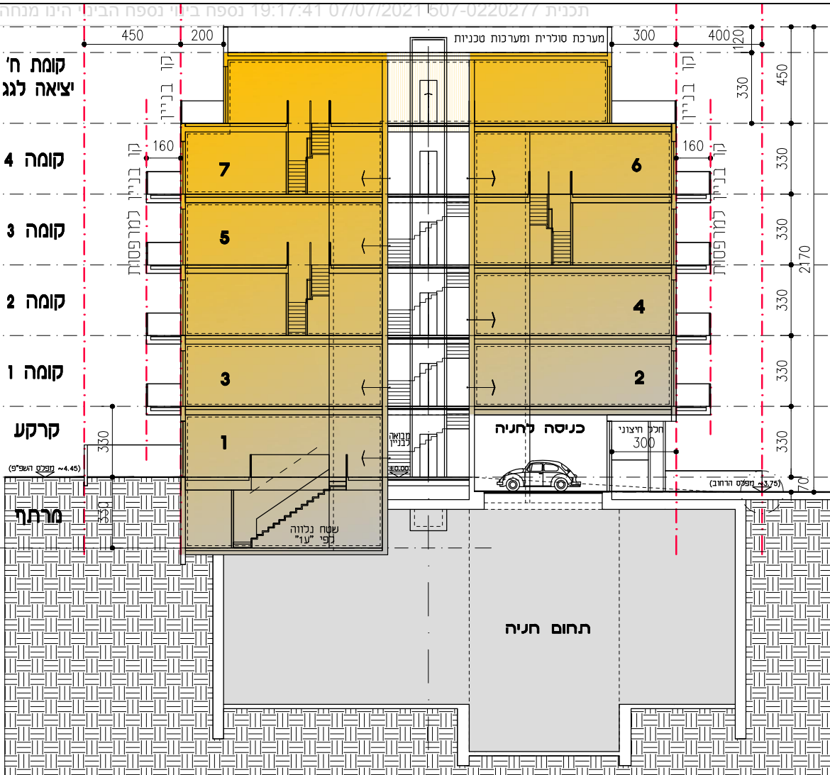
חתך עקרוני 1:250
