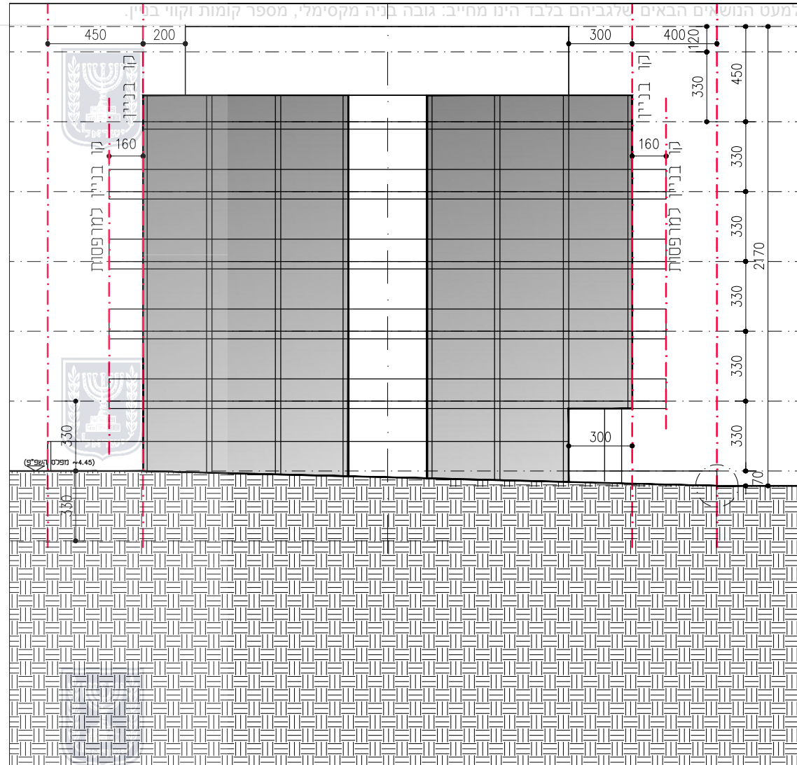
חזית עקרונית למערב - קיר דקורטיבי לשפ"פ 1:250
