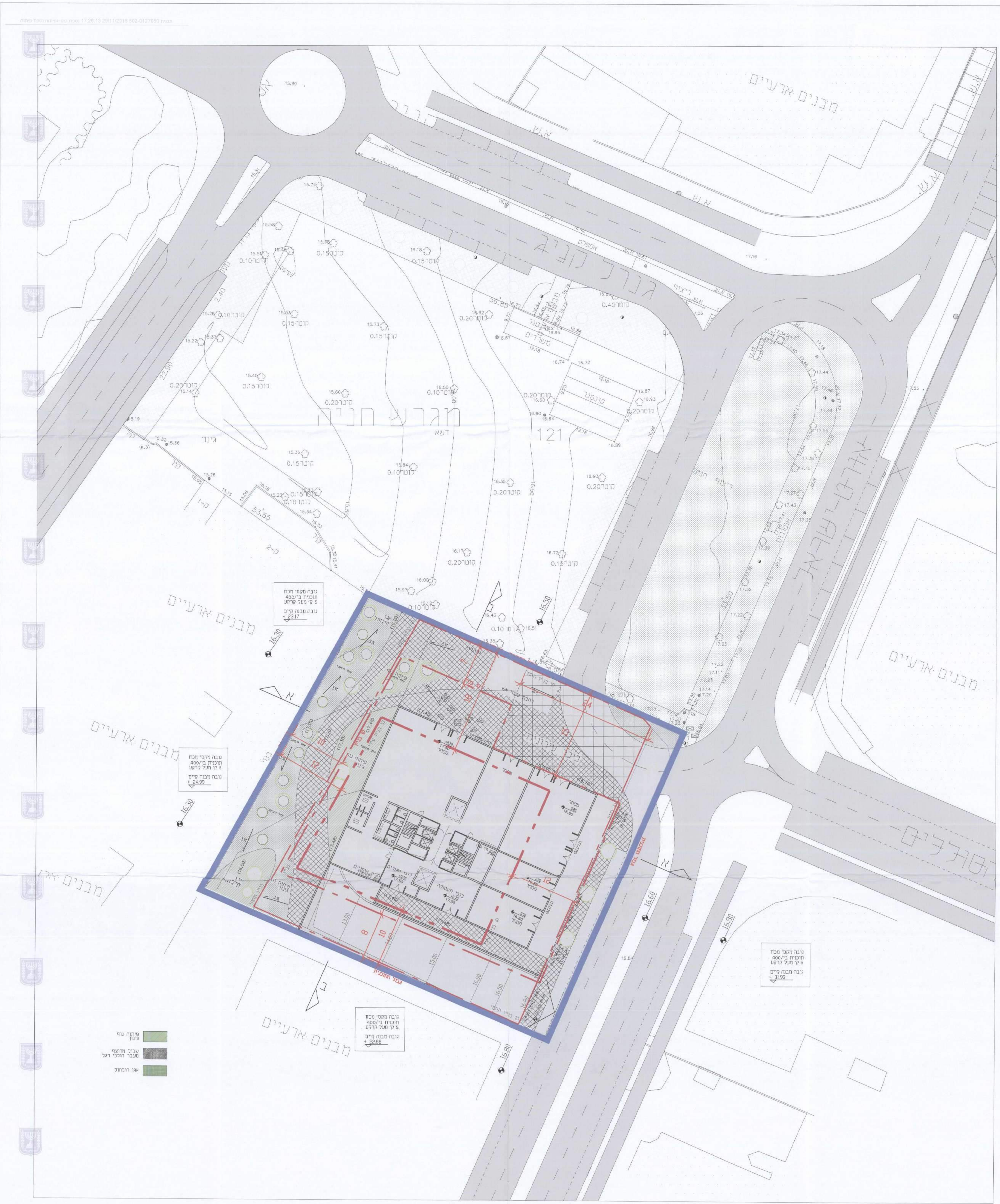
תוכנית פיתוח קומת קרקע 1:250
