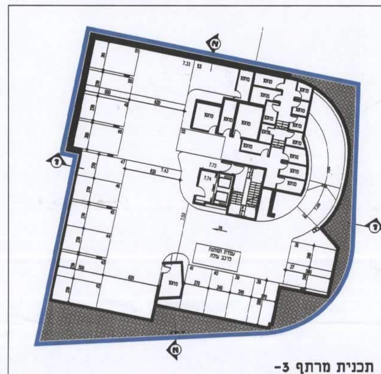
תכנית מרתף 3-3
