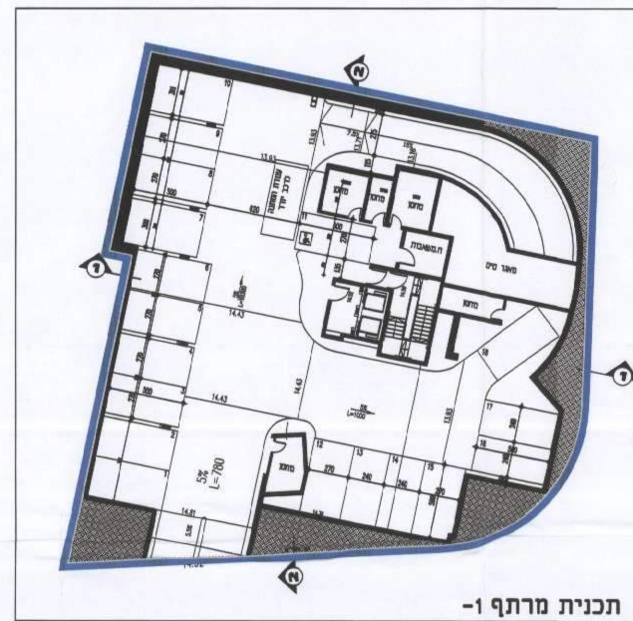
תכנית מרתף 1-1
