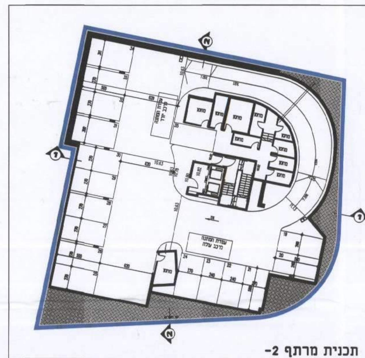
תכנית מרתף 2-2
