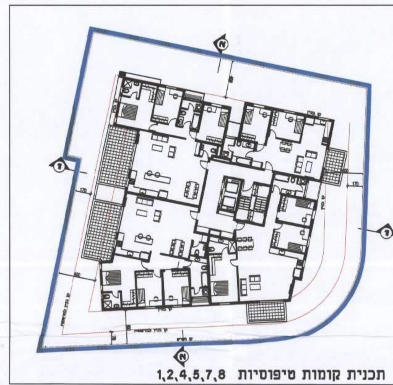
תכנית קומות טיפוסיות 1,2,4,5,7,8
