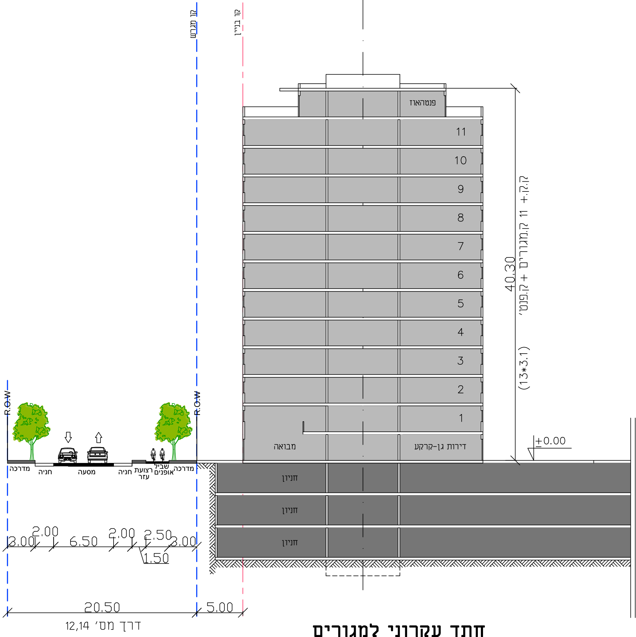
חתך עקרוני למגורים דרכים מסי 12,14 ק.מ. 1:250
