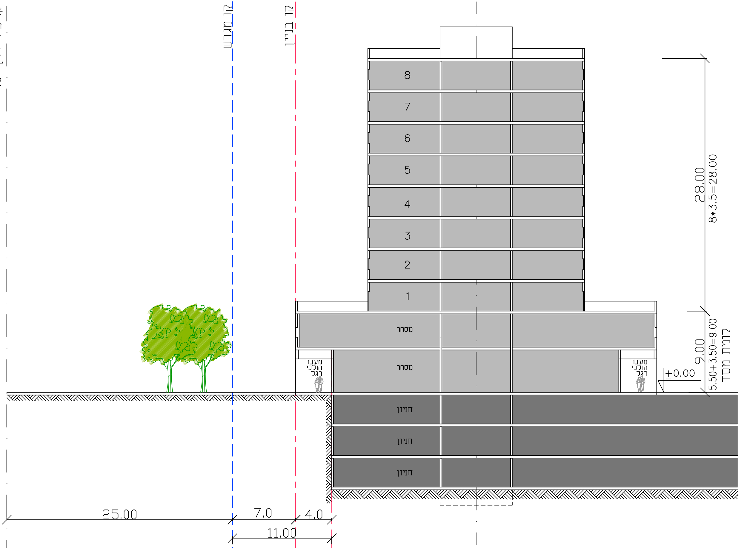
חתך עקרוני למבנה מסחר ותעסוקה עם חפיפה לדרך 461 ק.מ. 1:250
