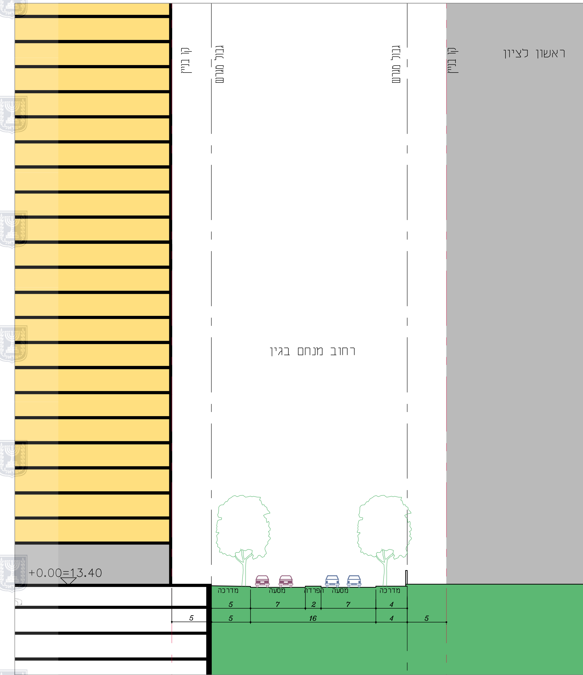
חתך ב-ב קנה מידה 1:250
