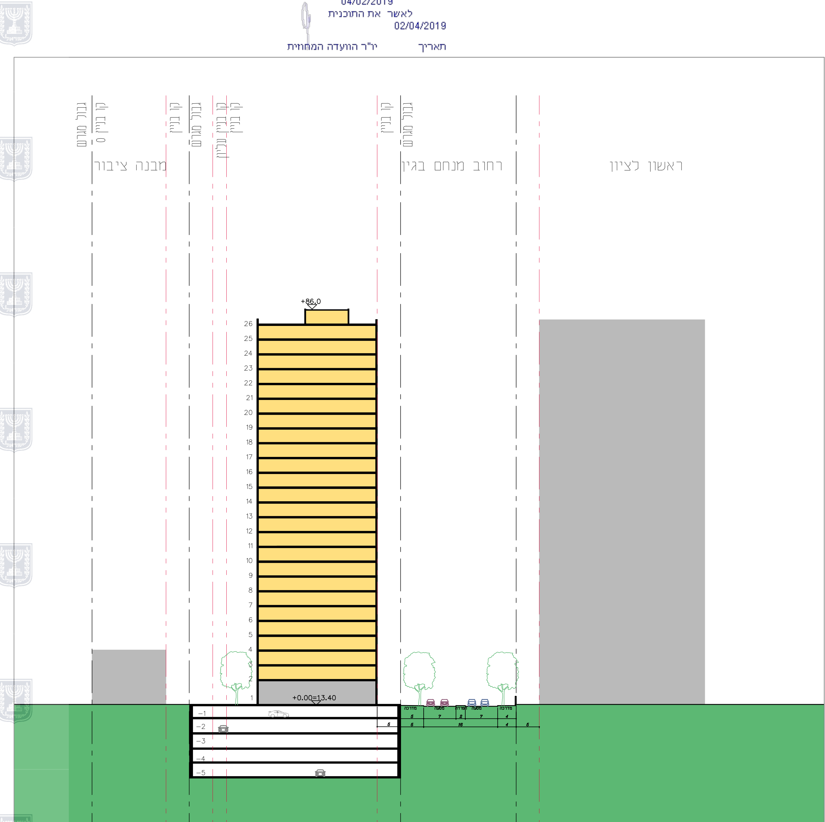
חתך ב-ב קנה מידה 1:500
