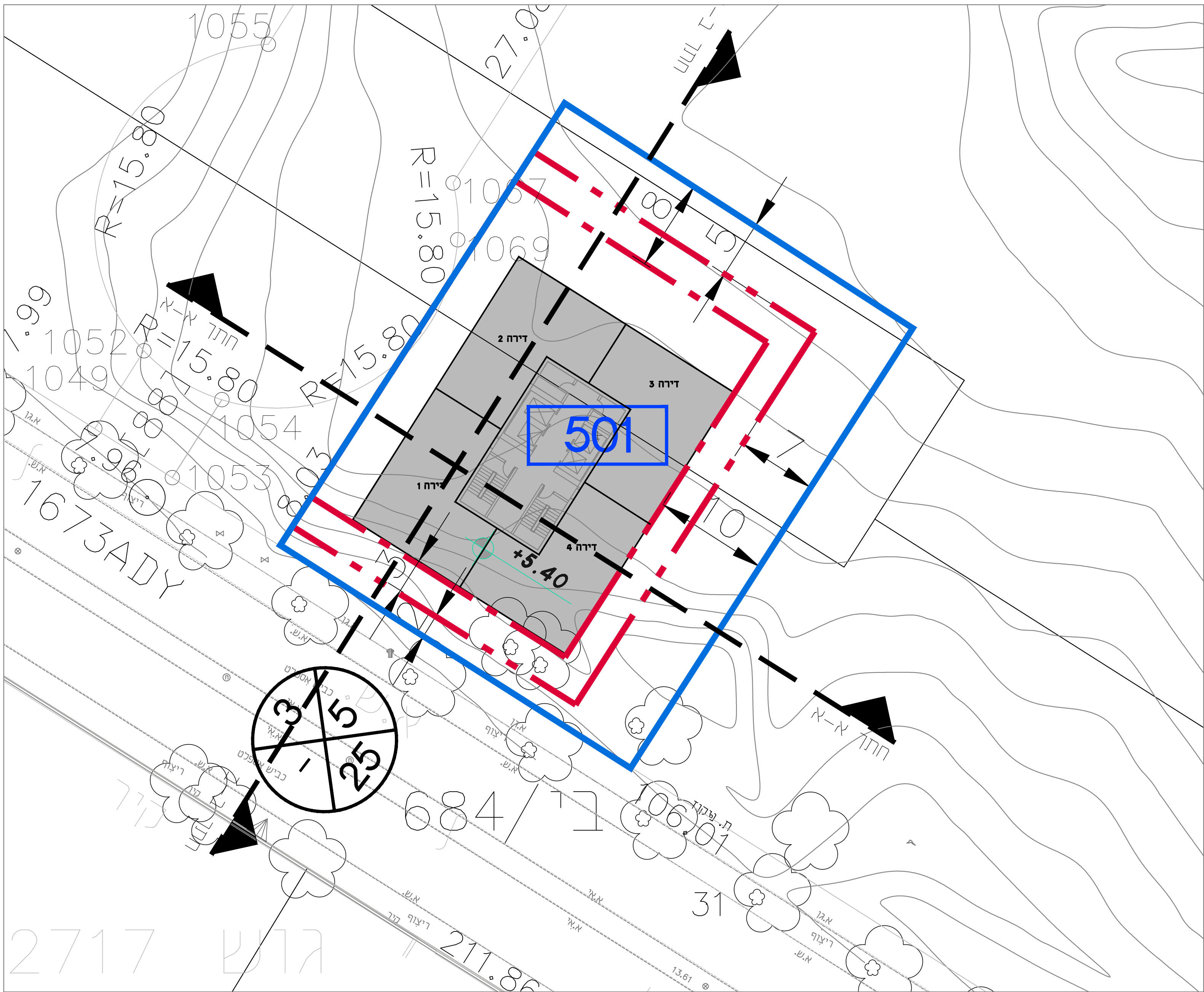
תכנית קומת מגורים טיפוסית קנ"מ 1:250
