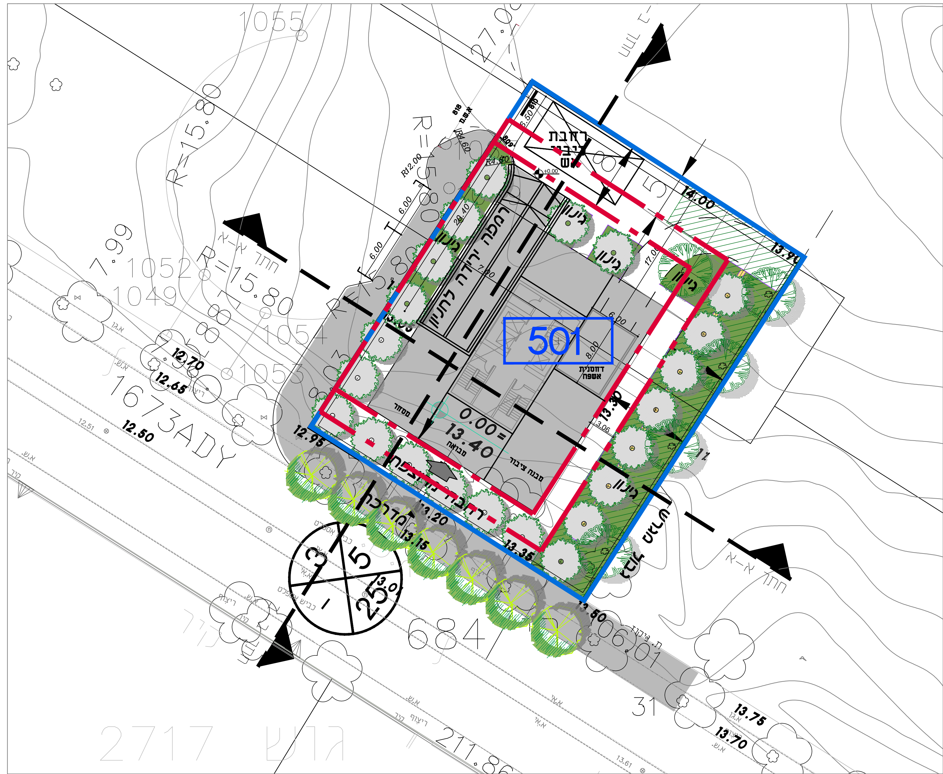
תכנית קומת קרקע קנ"מ 1:250
