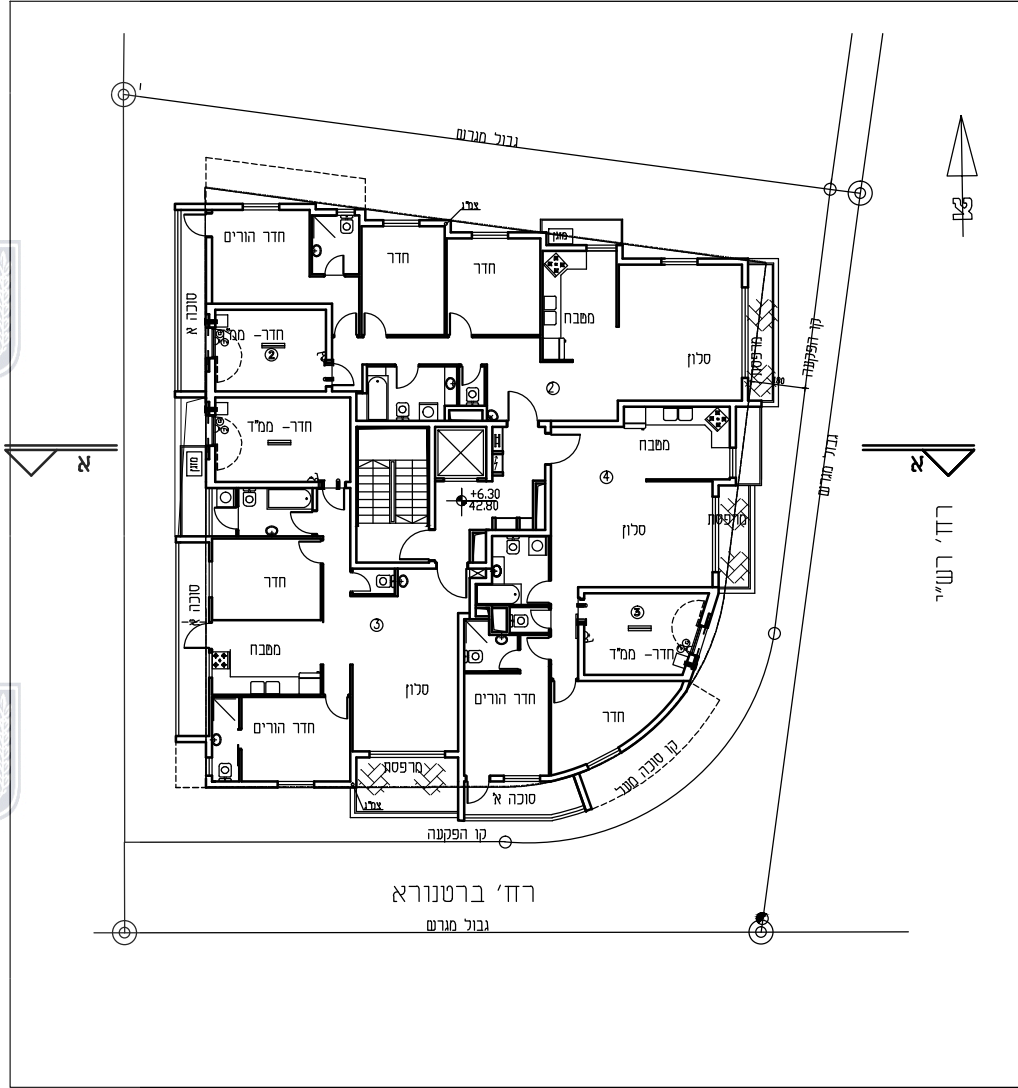
קומה א' ק"מ 1:250
