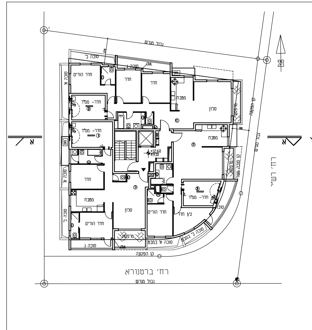
קומה ו' ק"מ 1:250
