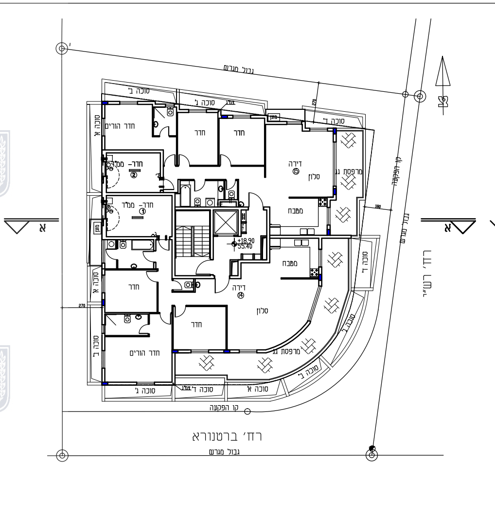
קומת ג' ק"מ 1:250
