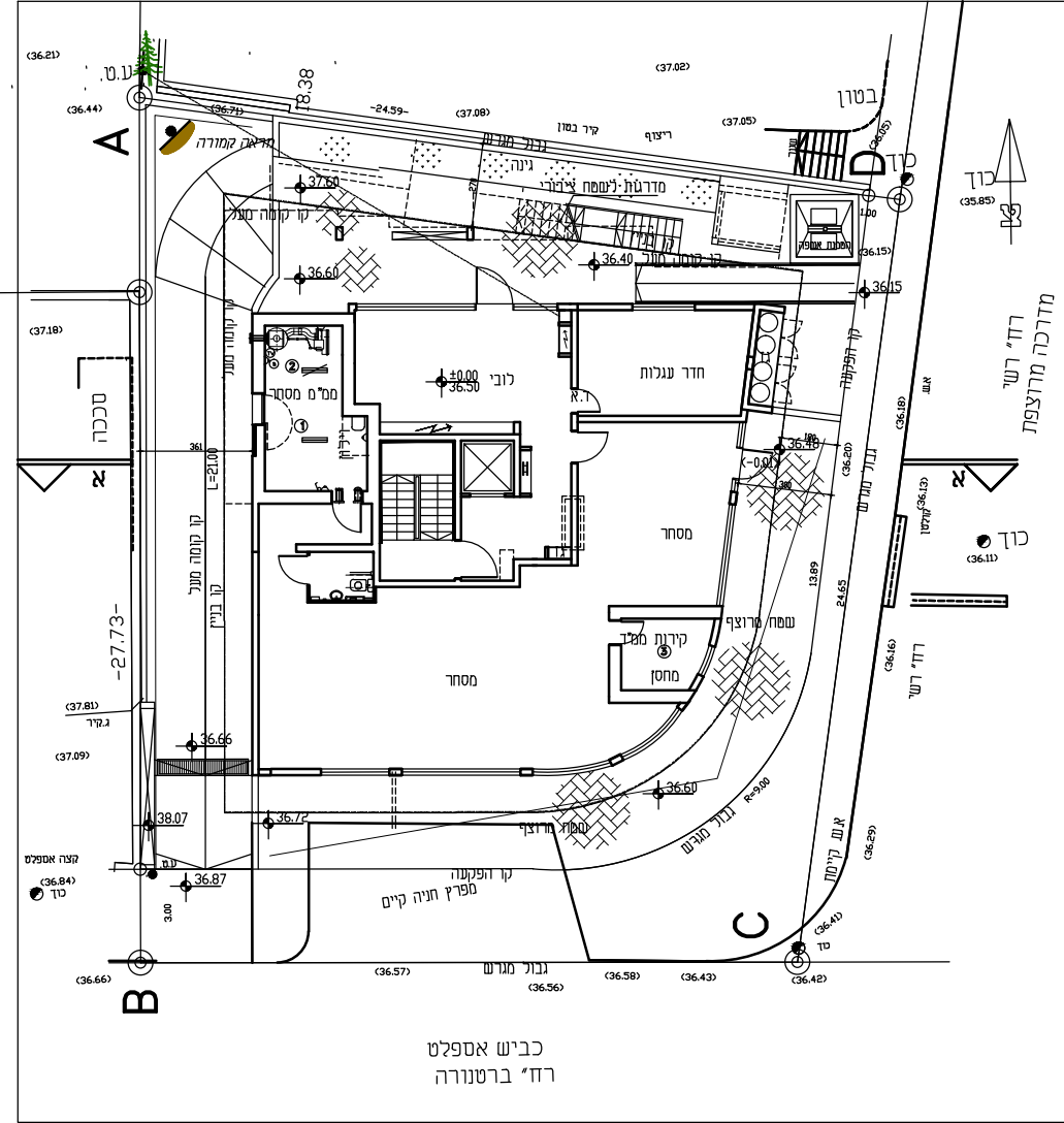
קומת קרקע ק"מ 1:250
