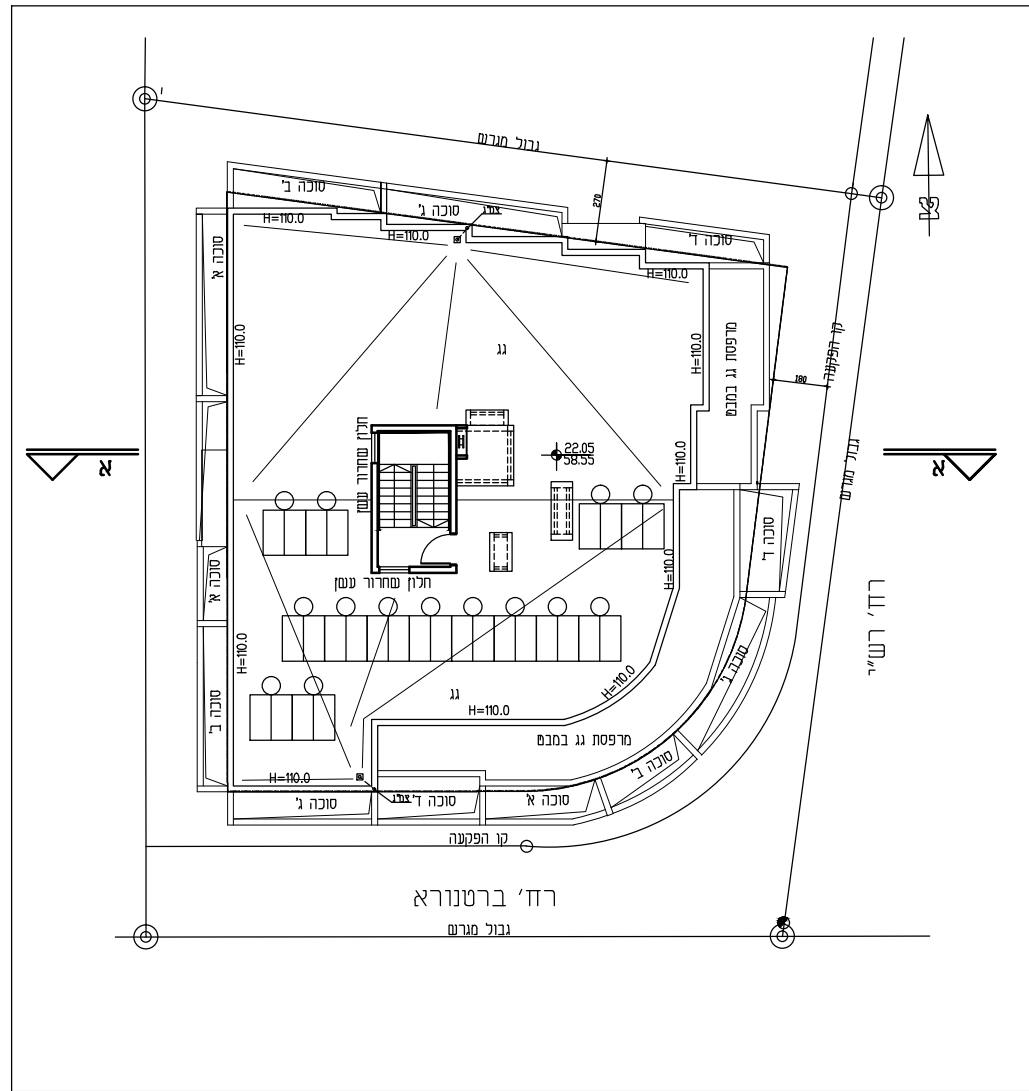
גג עליזן ק"מ 1:250
