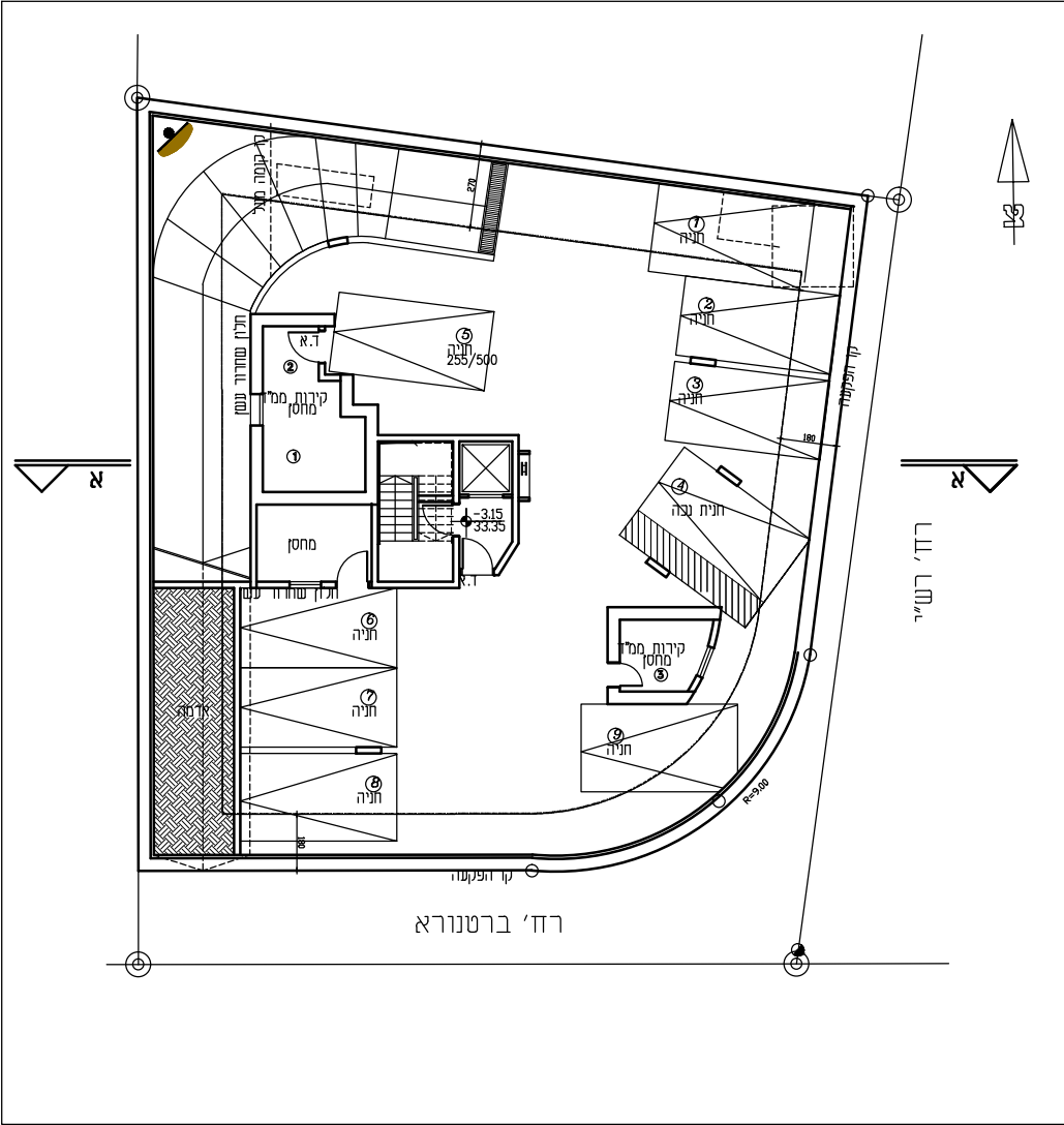
קומת מרתף ק"מ 1:250
