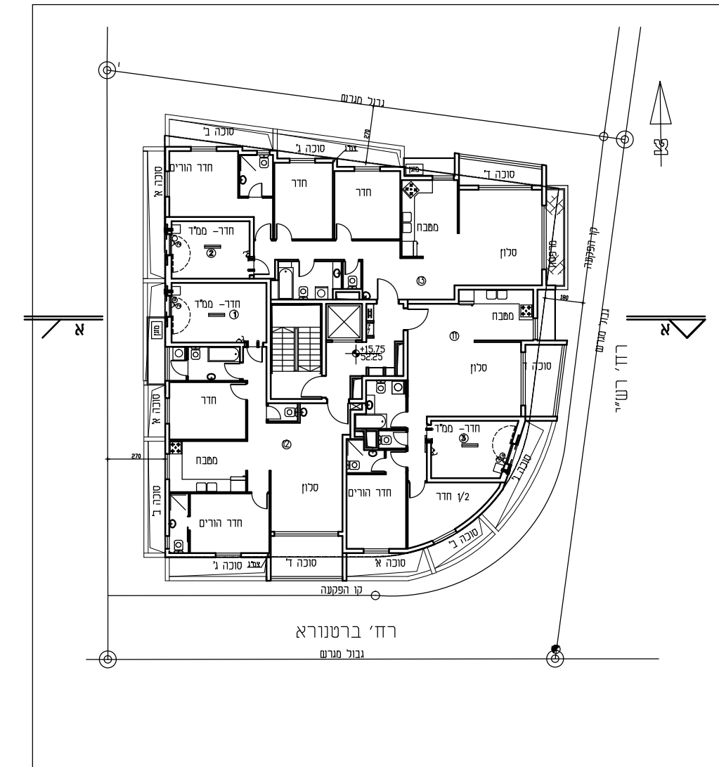
קומה ד' ק"מ 1:250
