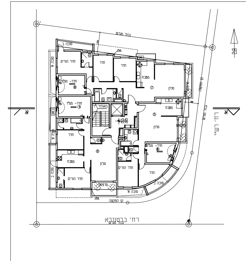
קומה ז' ק"מ 1:250
