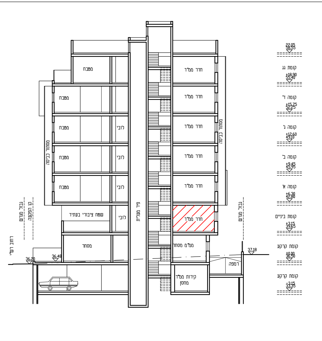
תחת א-א ק"מ 1:250
