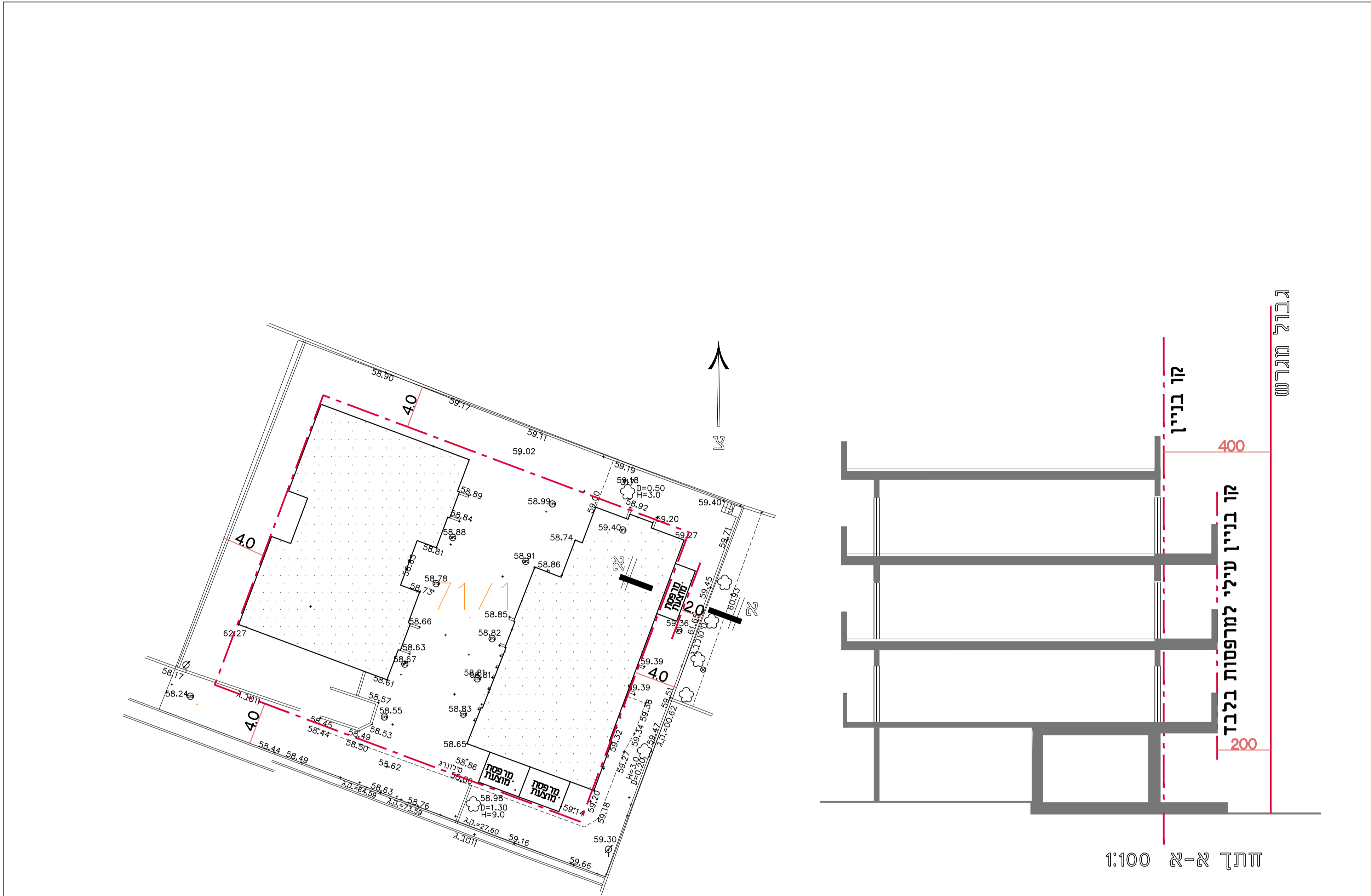
תרשים מגרש 1:250
