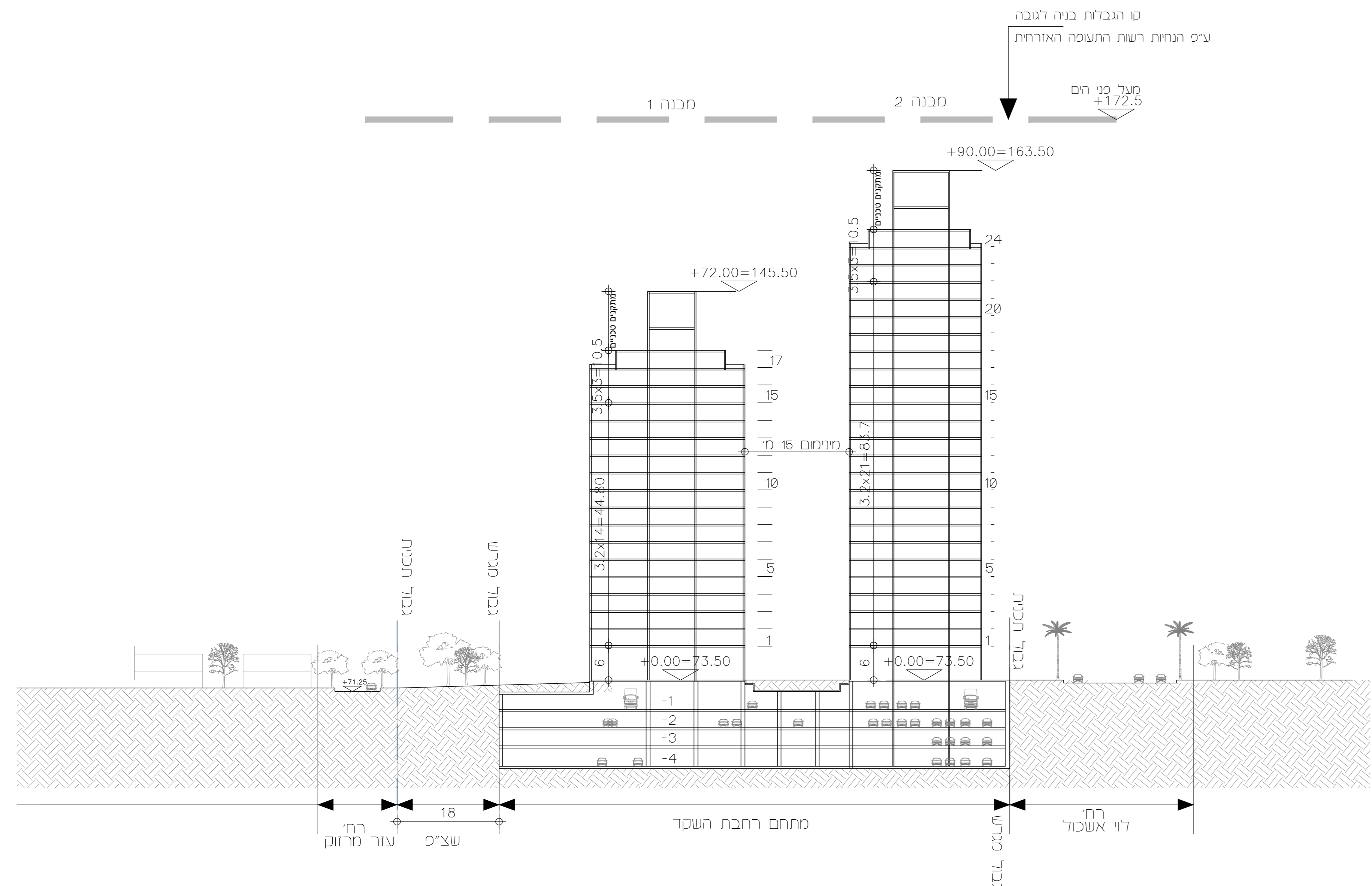
חתך א-א 1:1000
