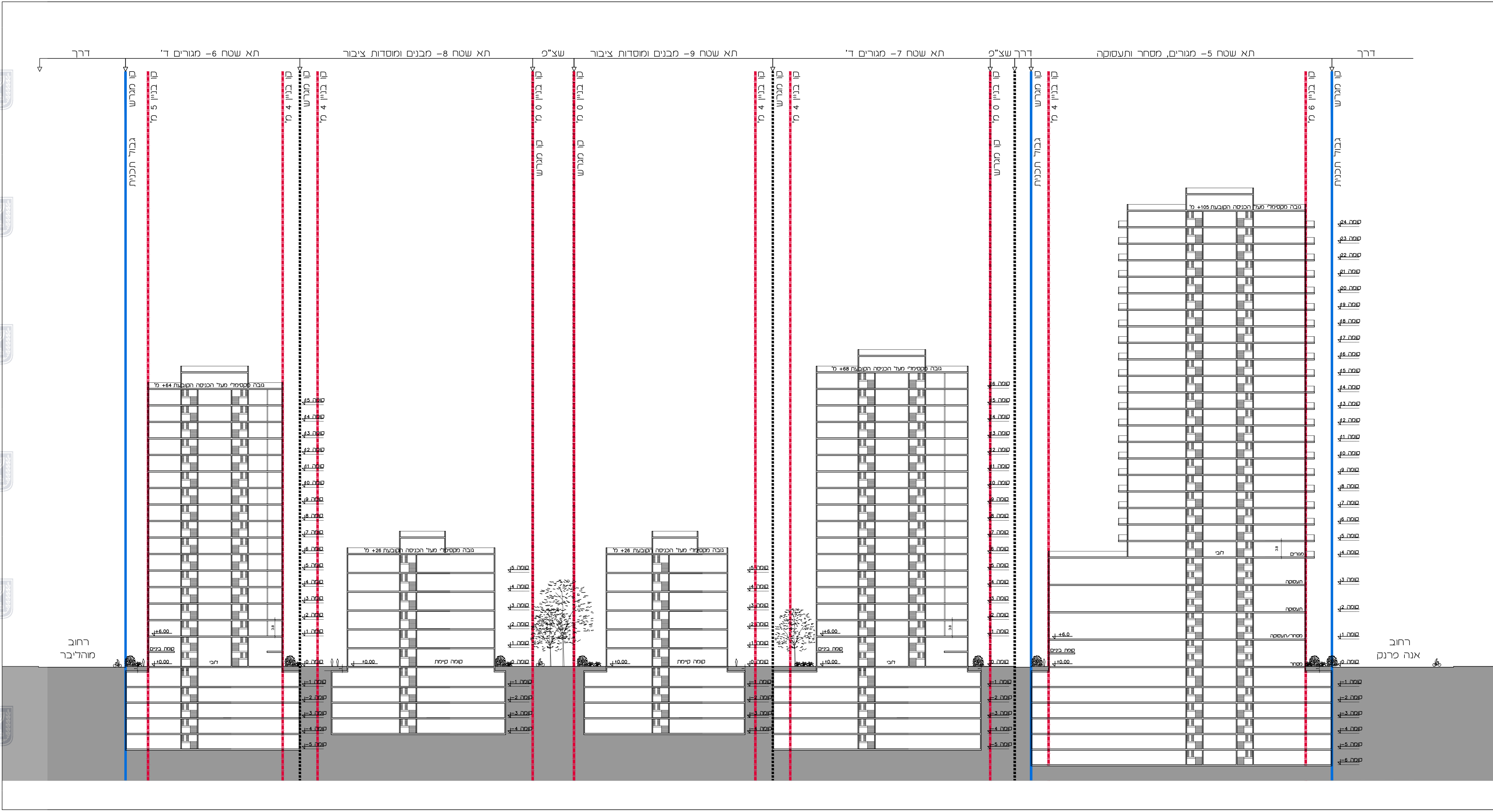
חתך אורך 1-1:500
