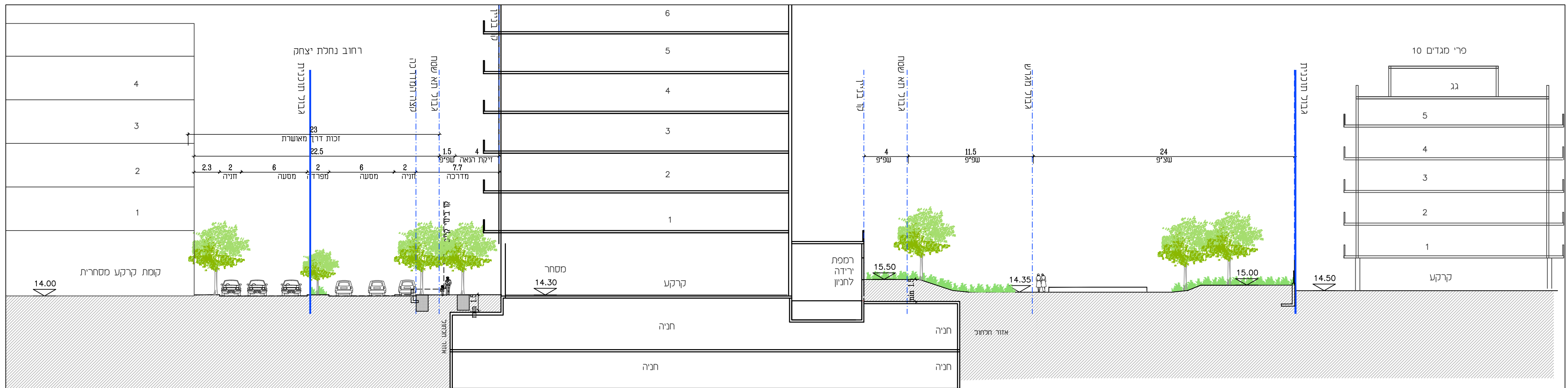
חתך א-א קנ"מ 1:250
