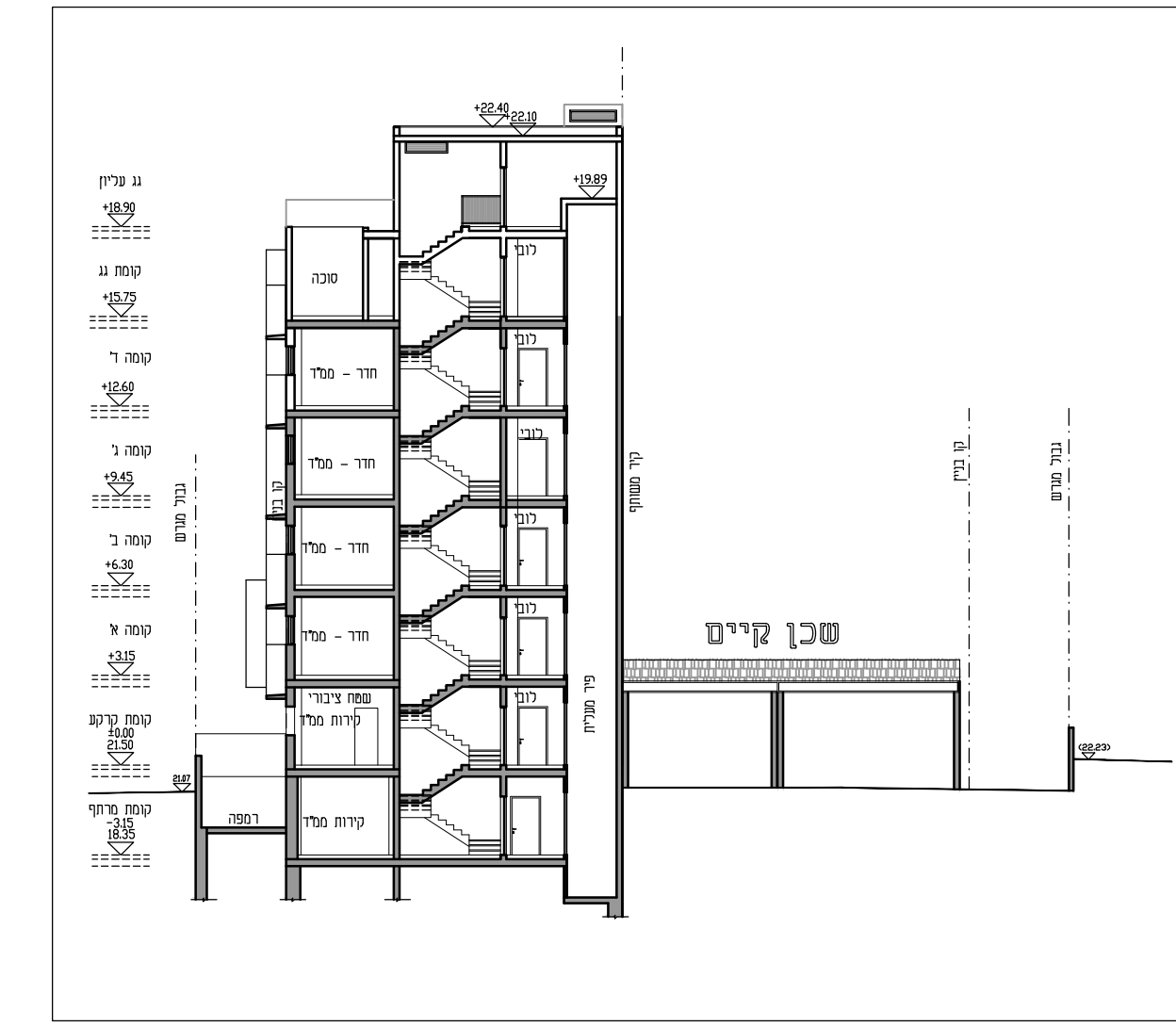
תתך ב-ב' קני"מ 1:250
