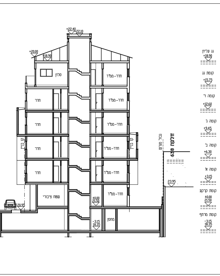
תתך א-א קני"מ 1:250
