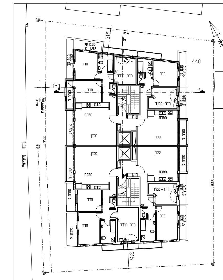
קופת ג' קני"מ 1:250
