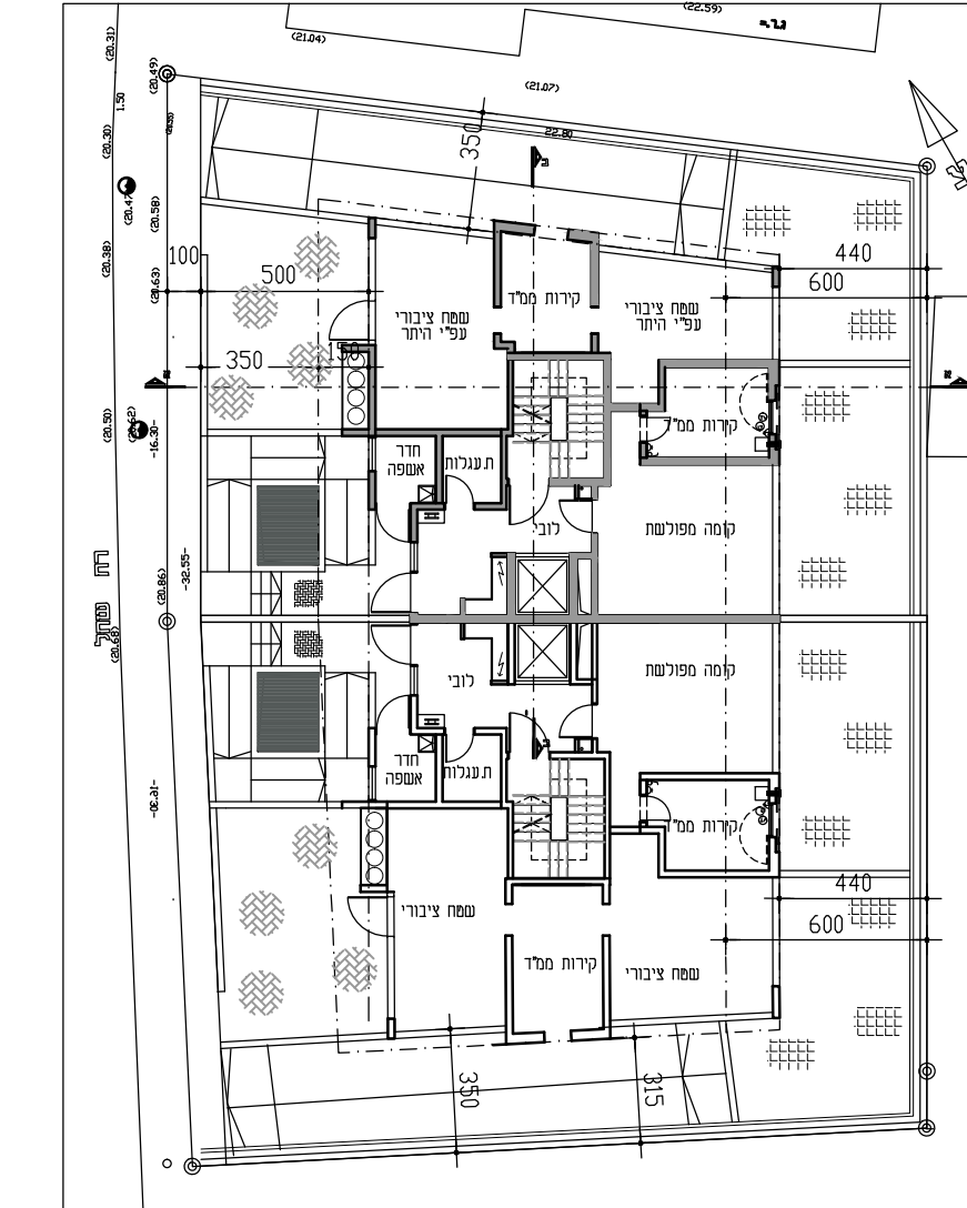
קופת קרקע קני"מ 1:250
