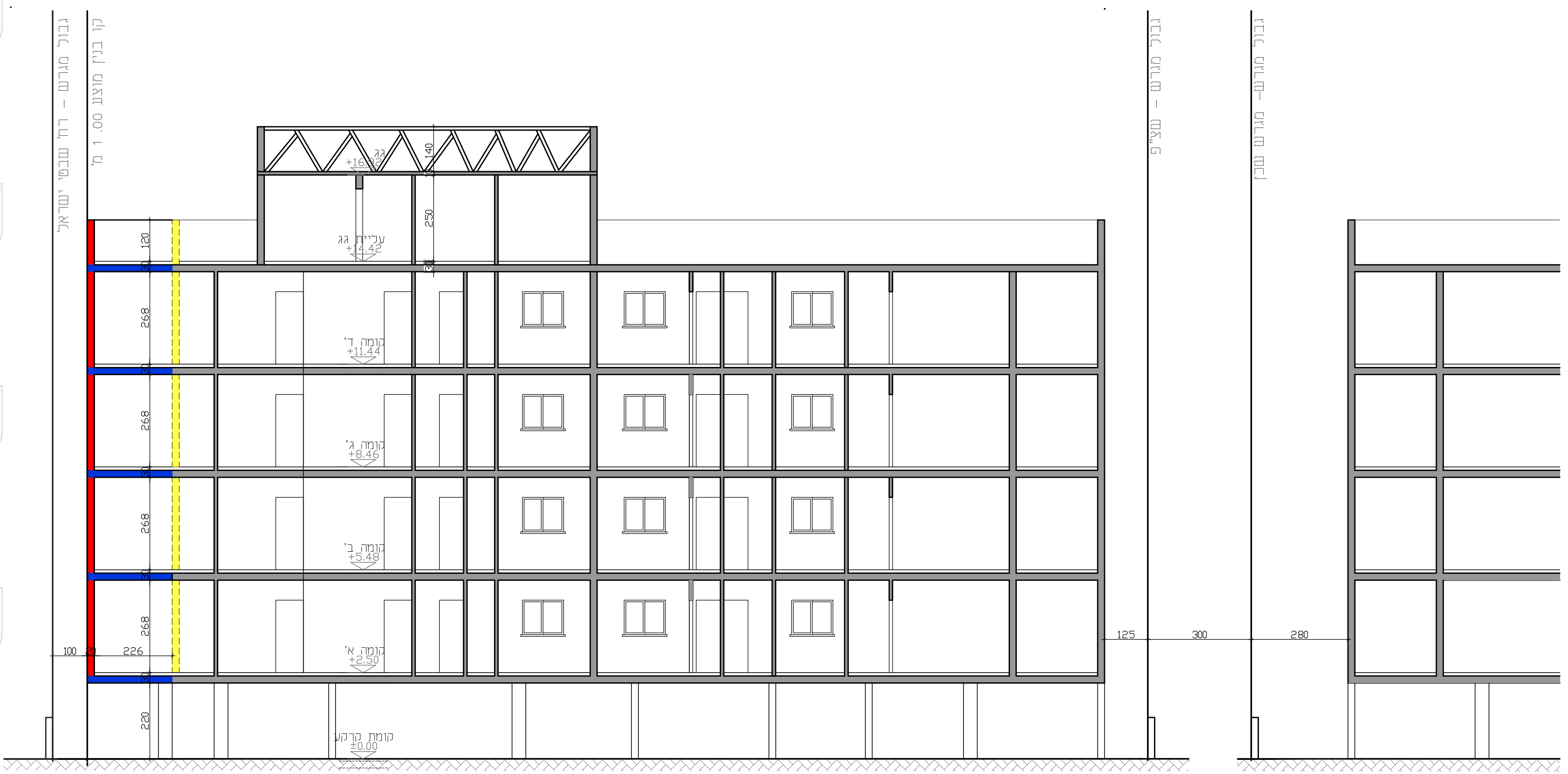
חתך א' א קל"מ 1:100
