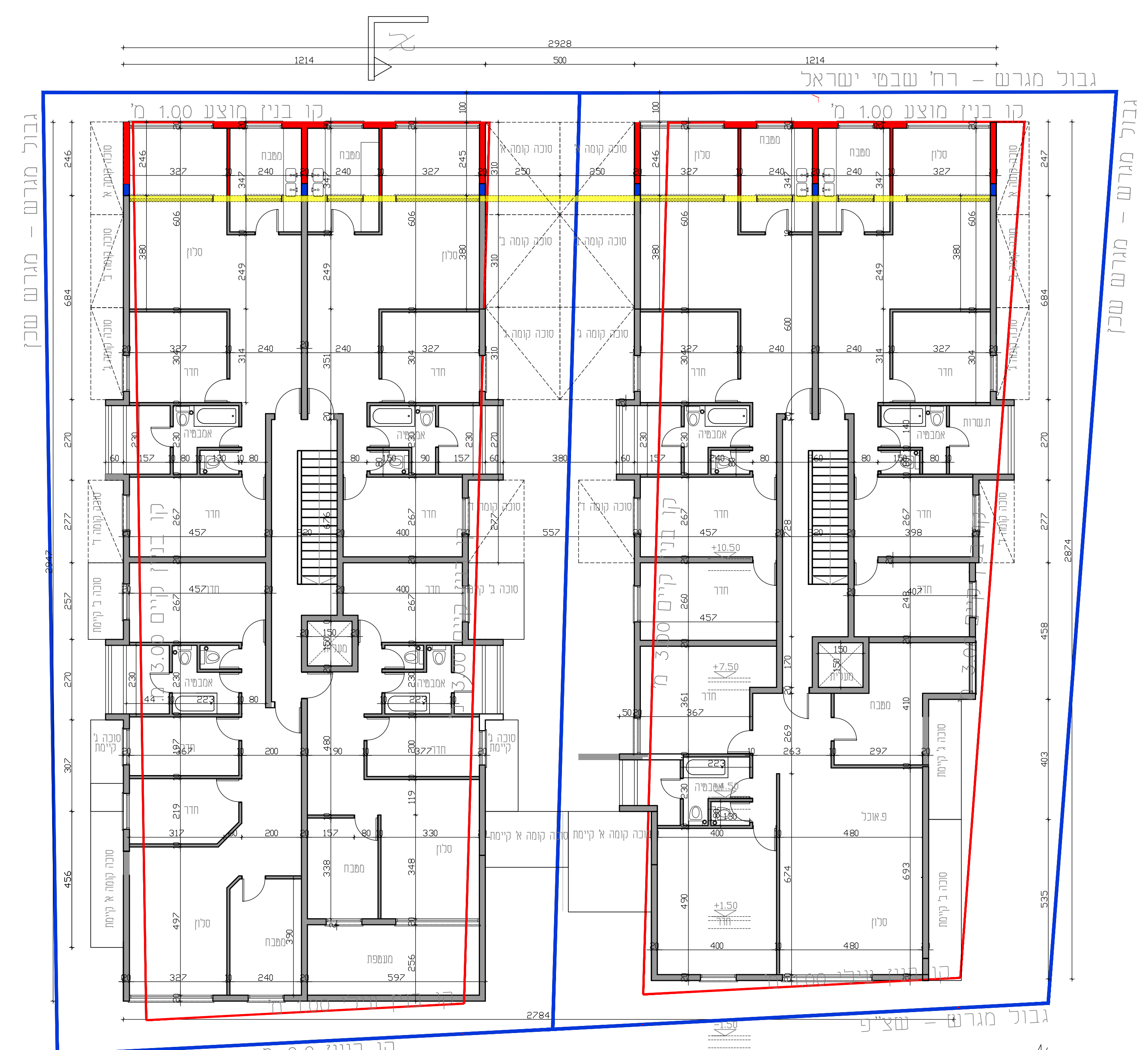
תוכנית קומה טיפוסית
