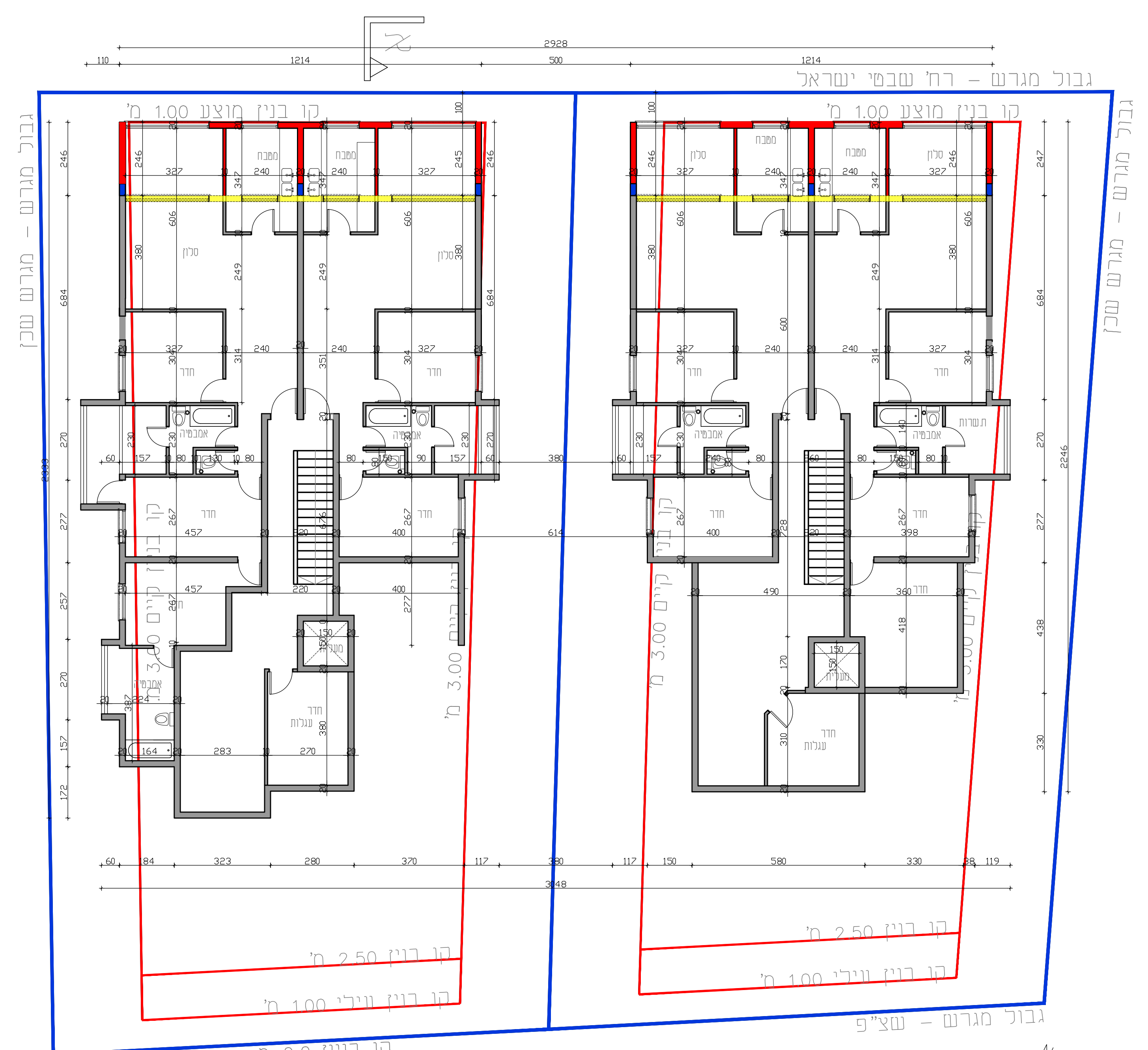
תוכנית קומת קרקע
