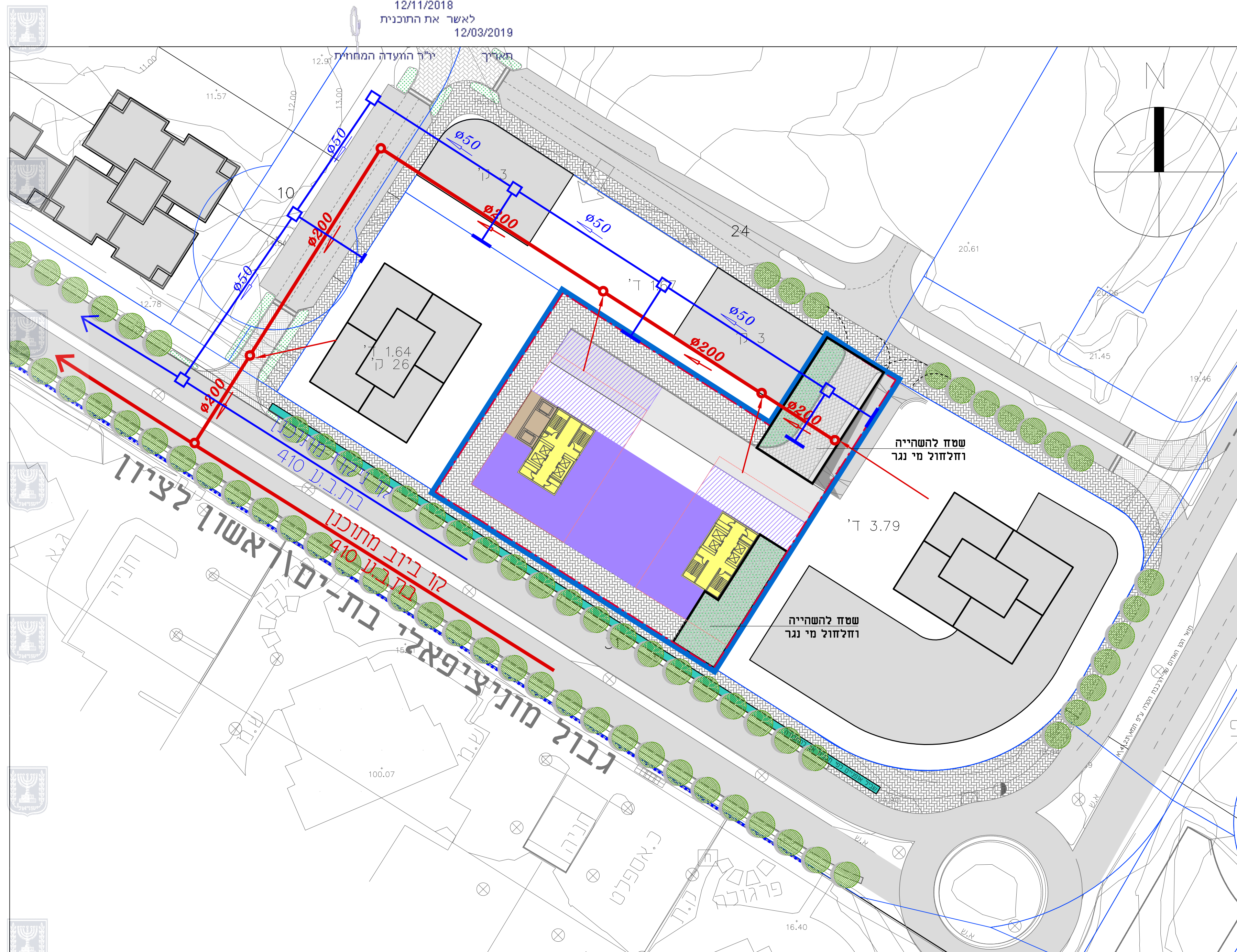
קומת קרקע - מפלס רחוב צפוני 1:500
