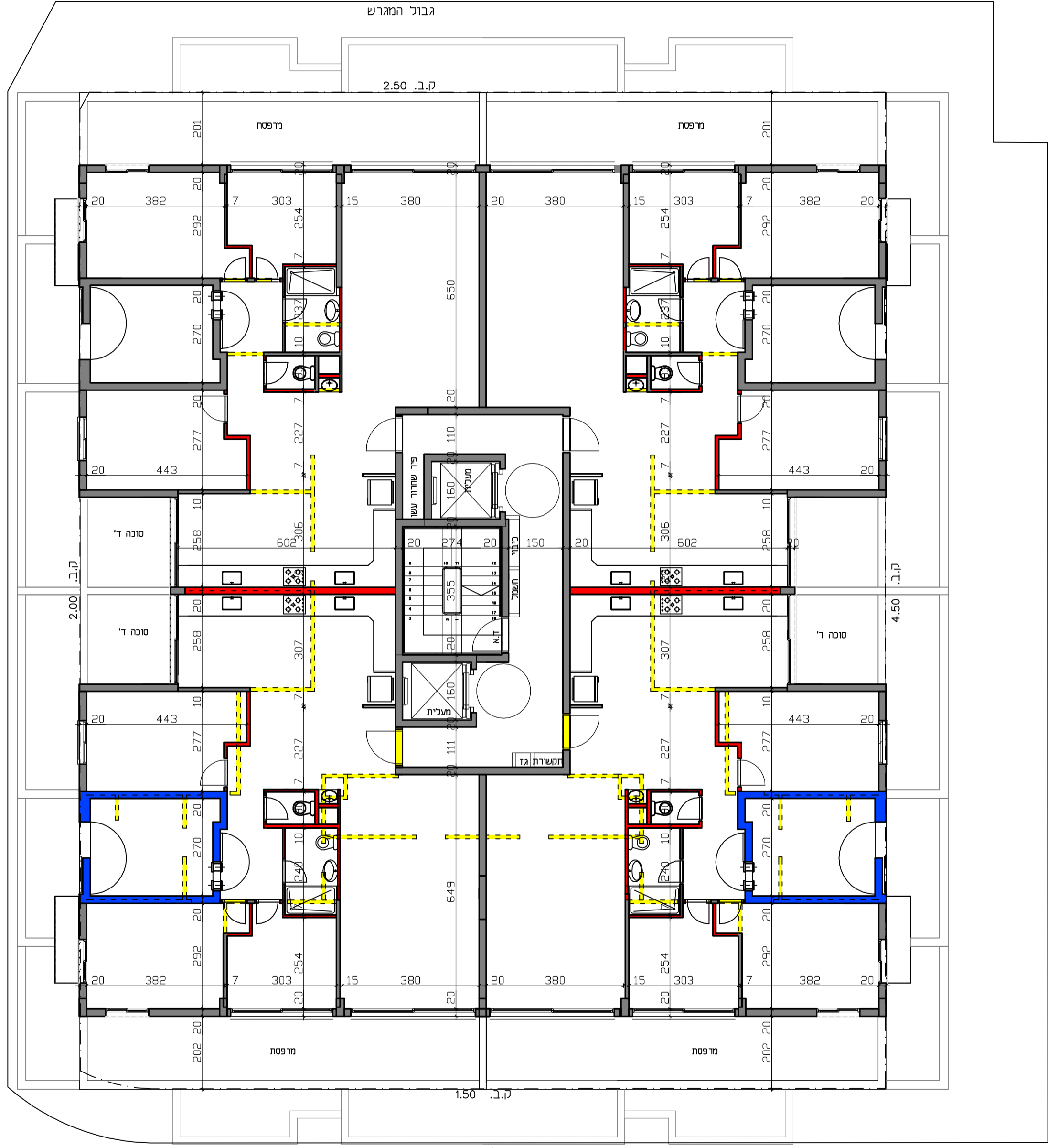
תכנית קומת הגג ק.פ. 1:50
