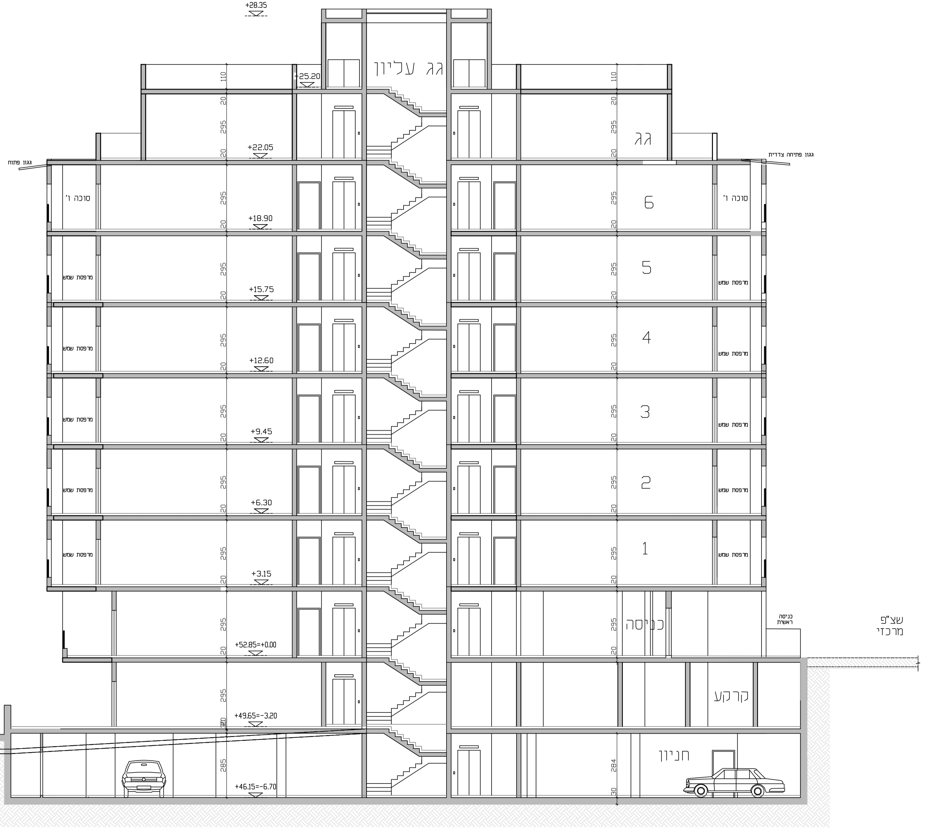
חתך ב-ב ק"פ 1:100
