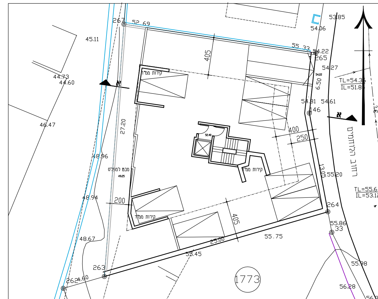
קומת חניה קנ"מ 1:250
