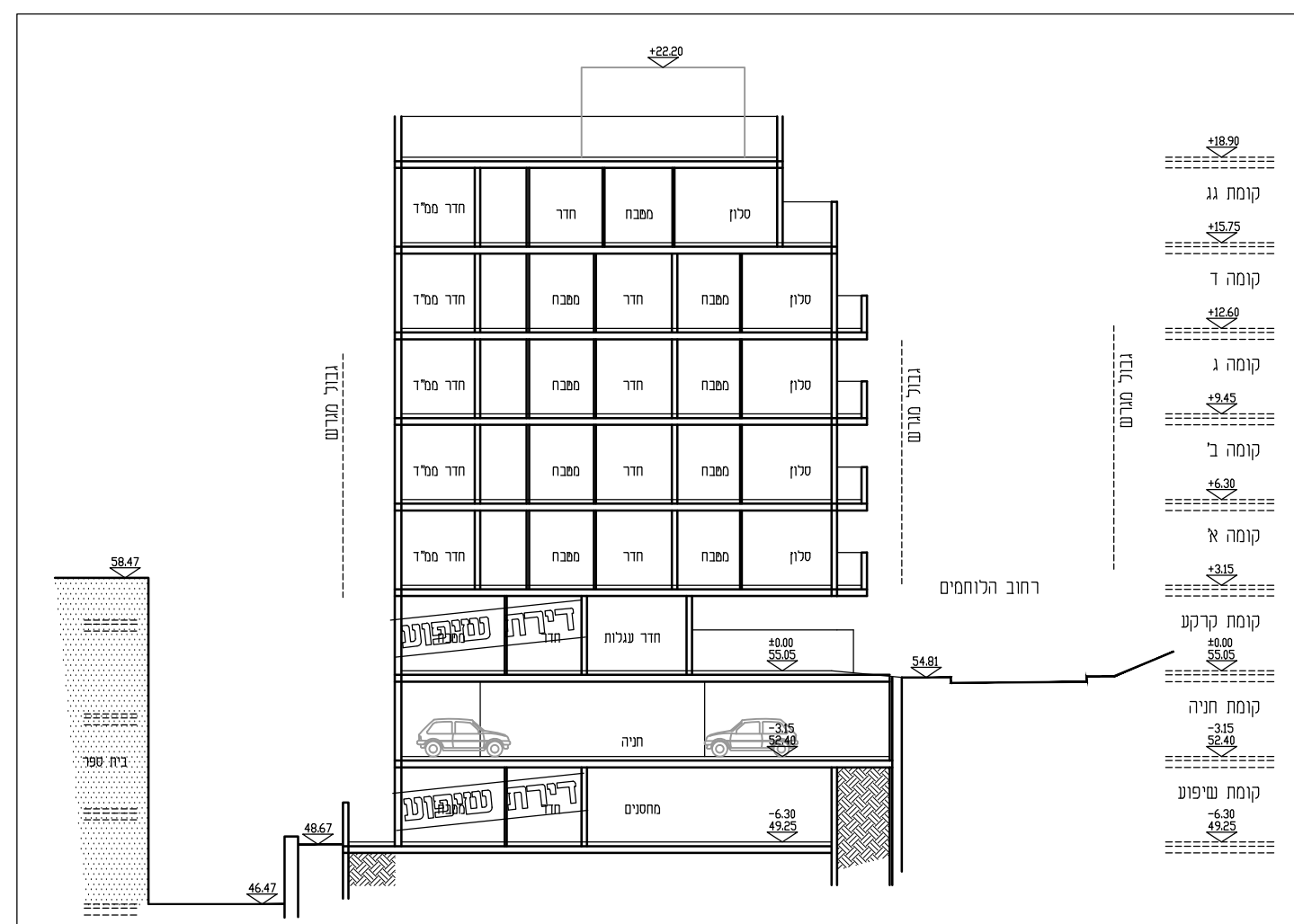
תתך א-א קנ"מ 1:250
