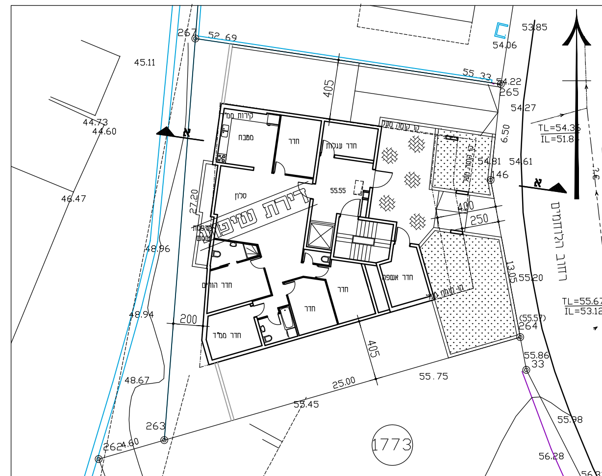
קומת קרקע קנ"מ 1:250
