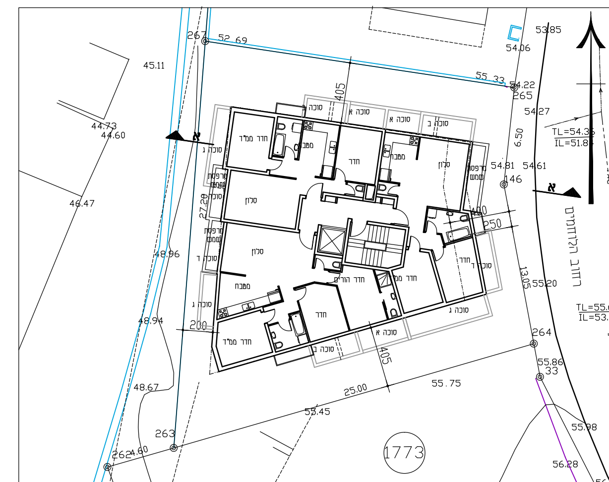
קומה שיפוטית קנ"מ 1:250
