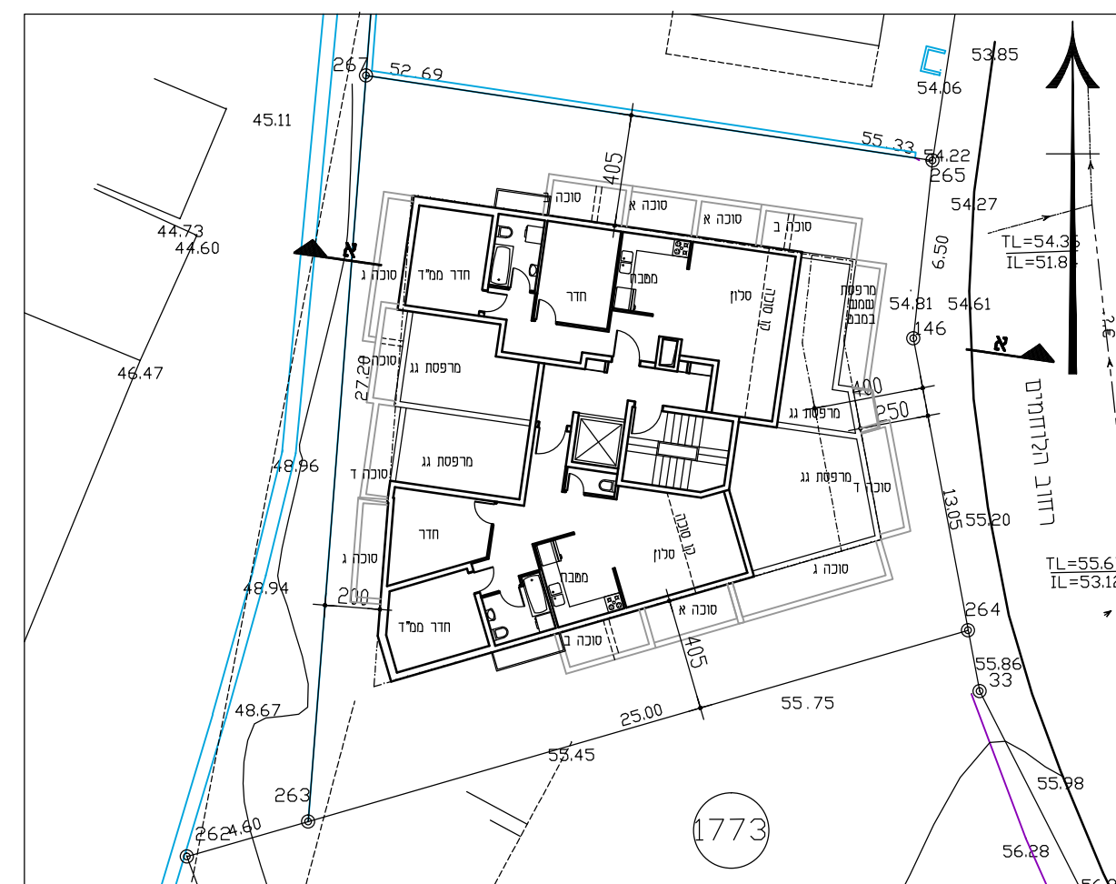
קומת גג קנ"מ 1:250
