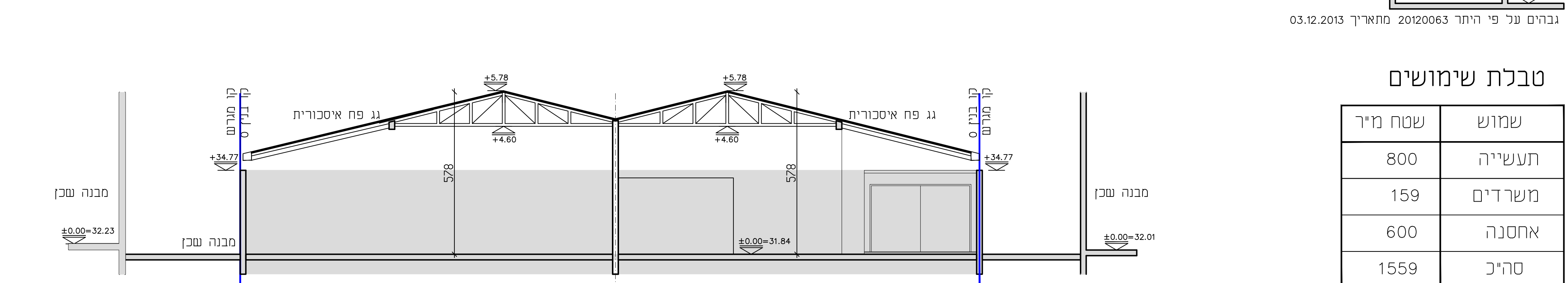
חותך 2 - 2 ק.מ. 1:100
