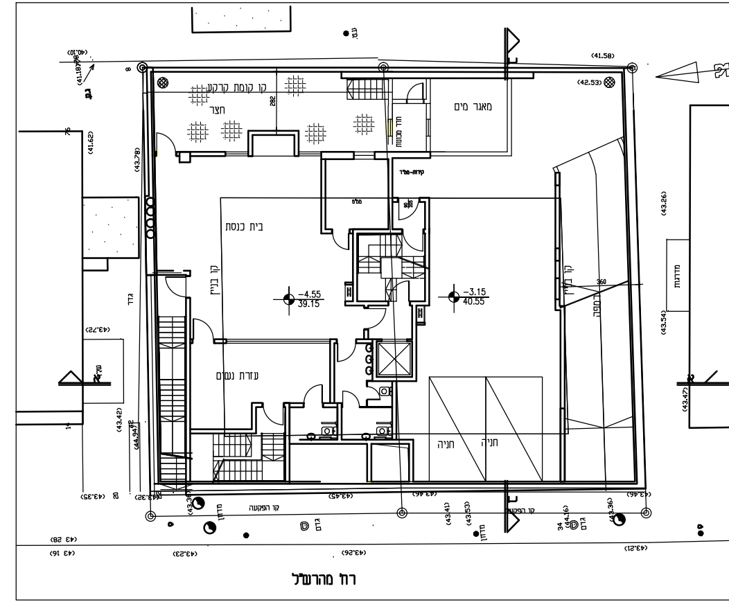
קומת מרתף ק"מ 1:250
