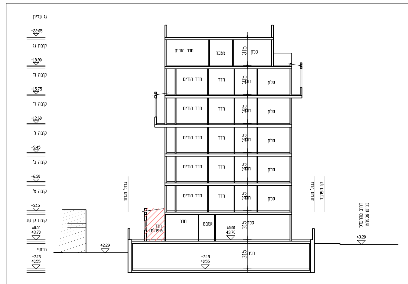
חתך ב-ב ק"מ 1:250
