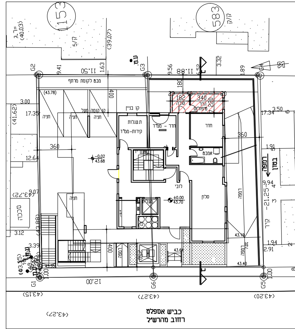
קומת קרקע ק"מ 1:250
