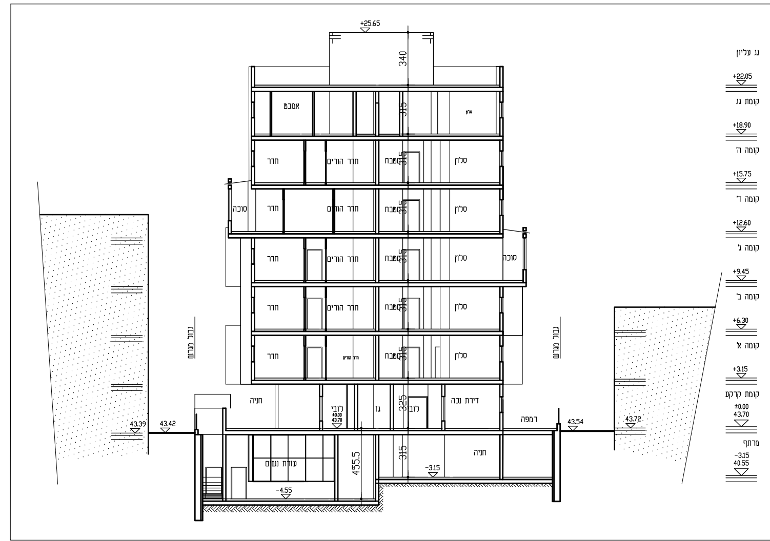
חתך א-א ק"מ 1:250
