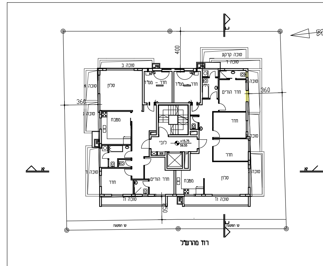
קומת א-ה ק"מ 1:250
