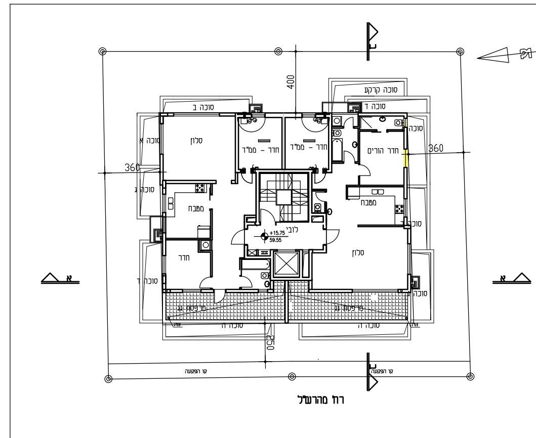
קומת גג ק"מ 1:250
