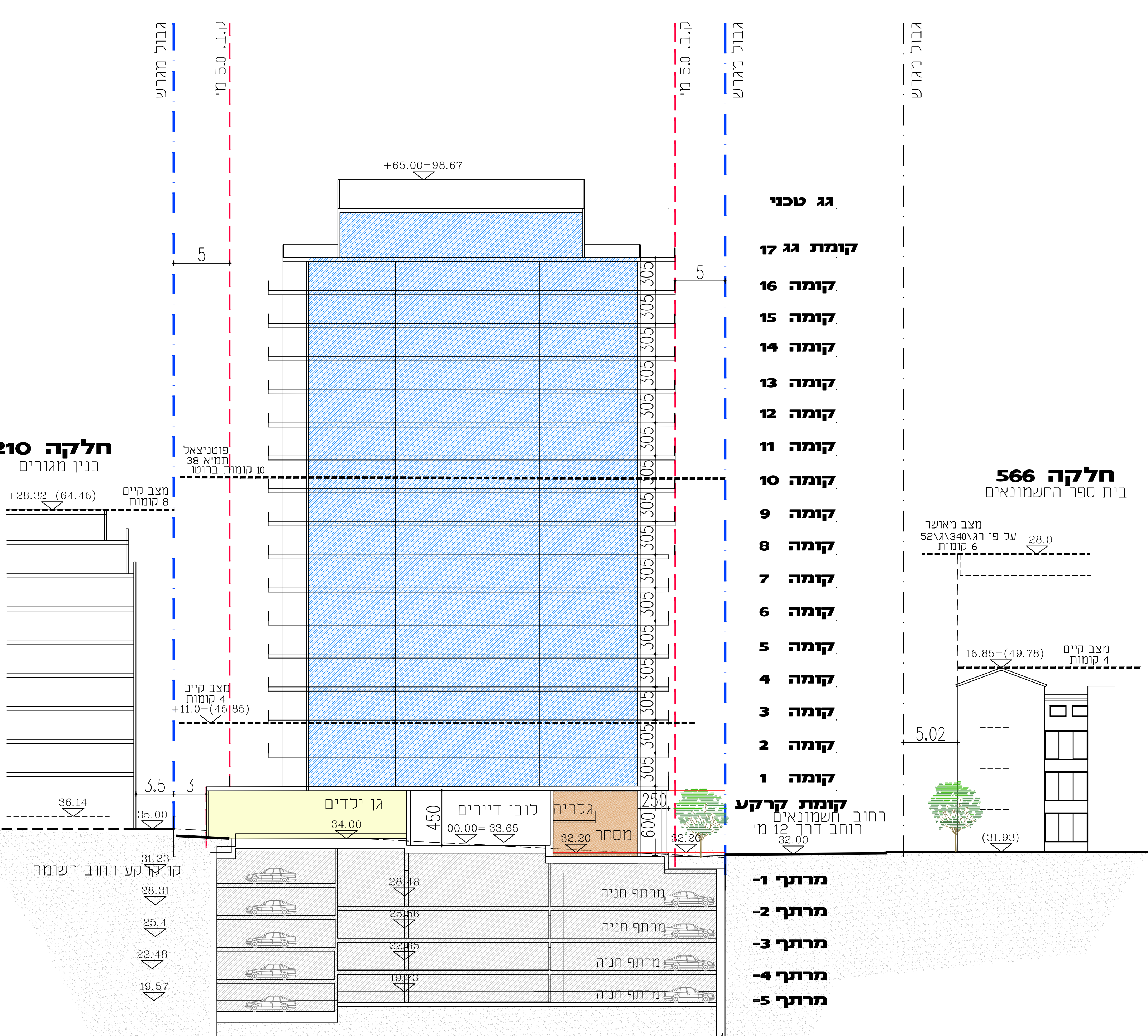
חתך א-א קני"מ 1 : 250
