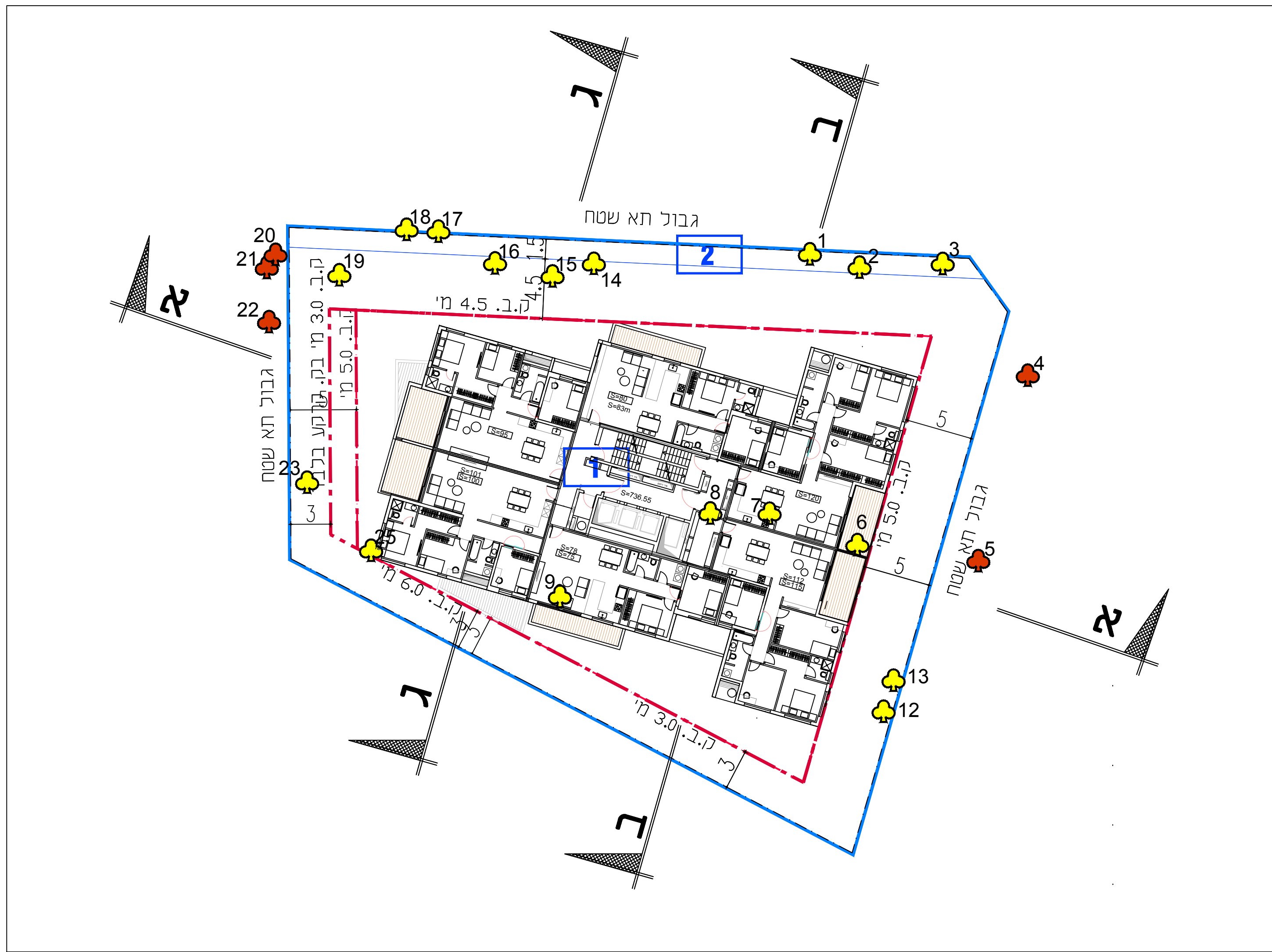
תכנית קומה טיפוסית קני"מ 1 : 250
