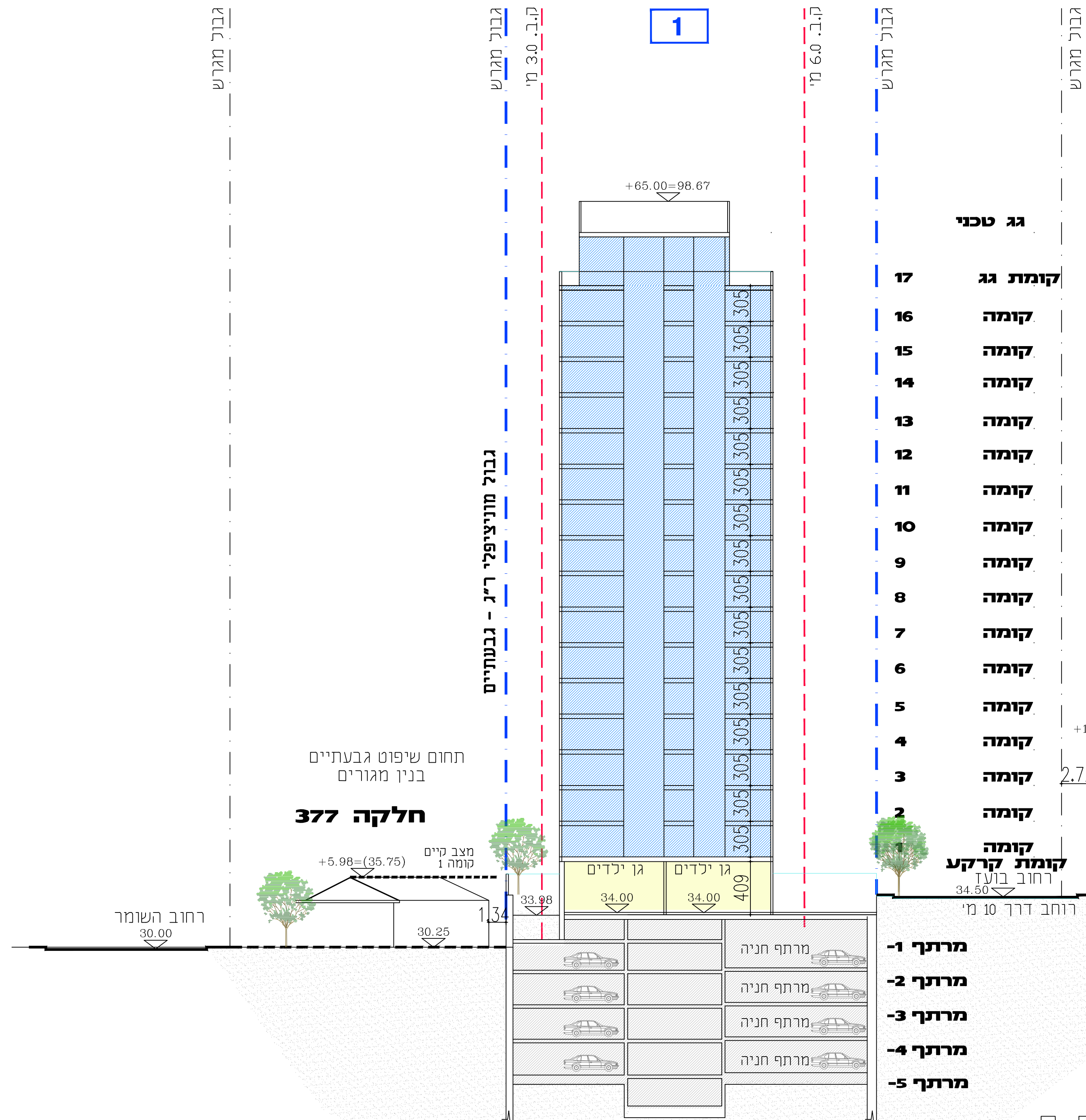
חתך ג-ג קני"מ 1 : 250
