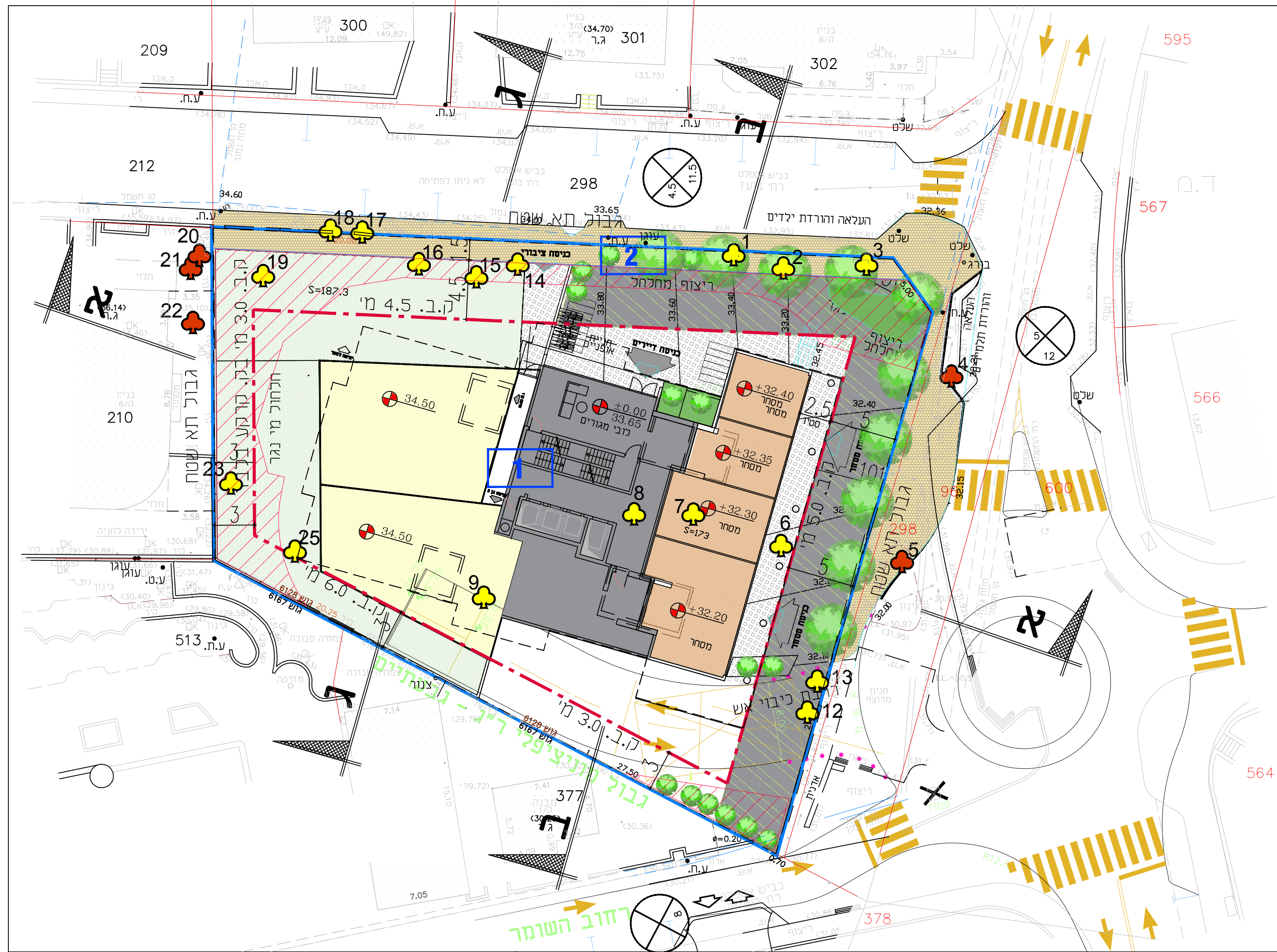
תכנית קומת ארקע קני"מ 1 : 250
