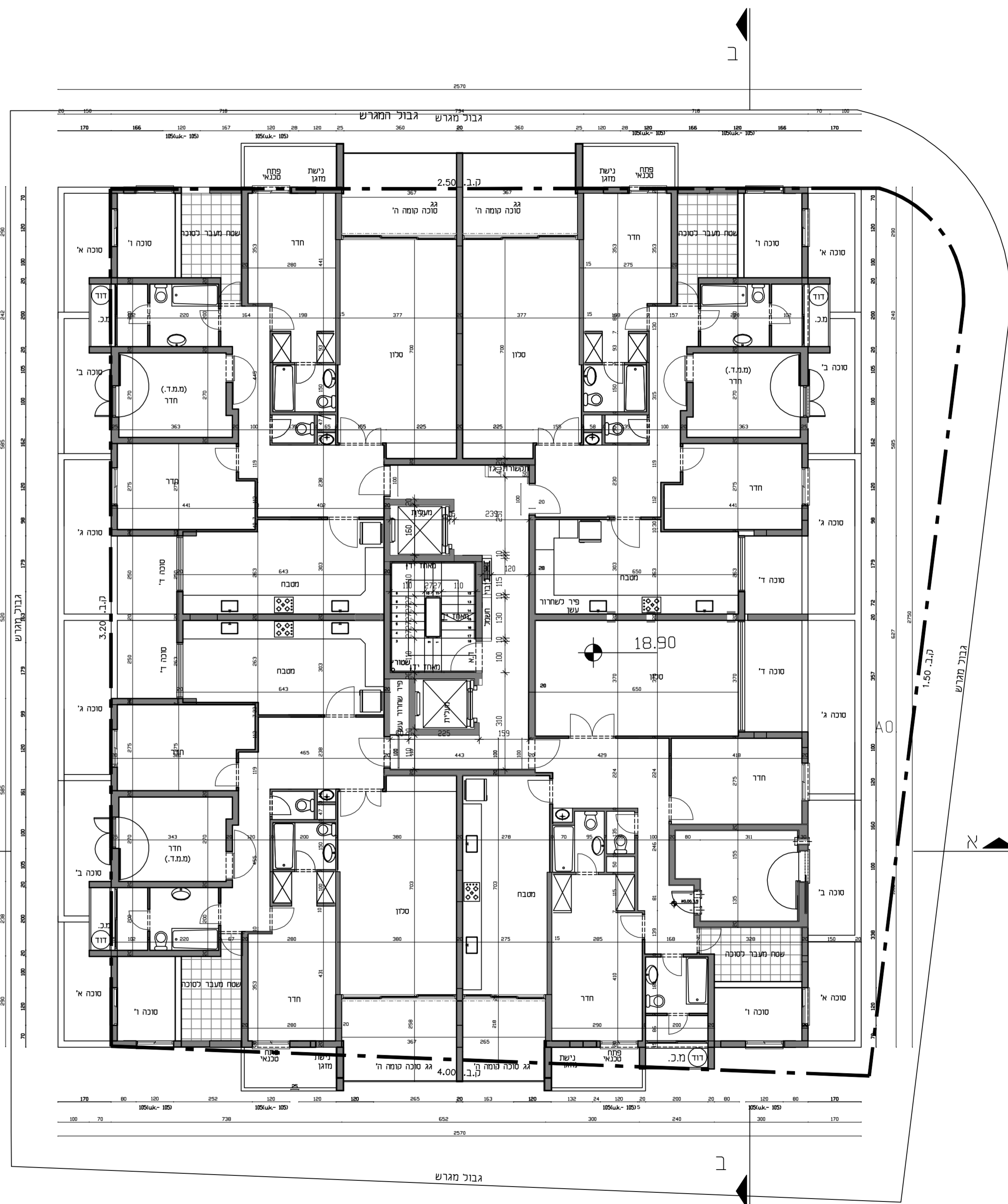
תכנית קוֹדֵת א' . ק . ד . 1 : 100
