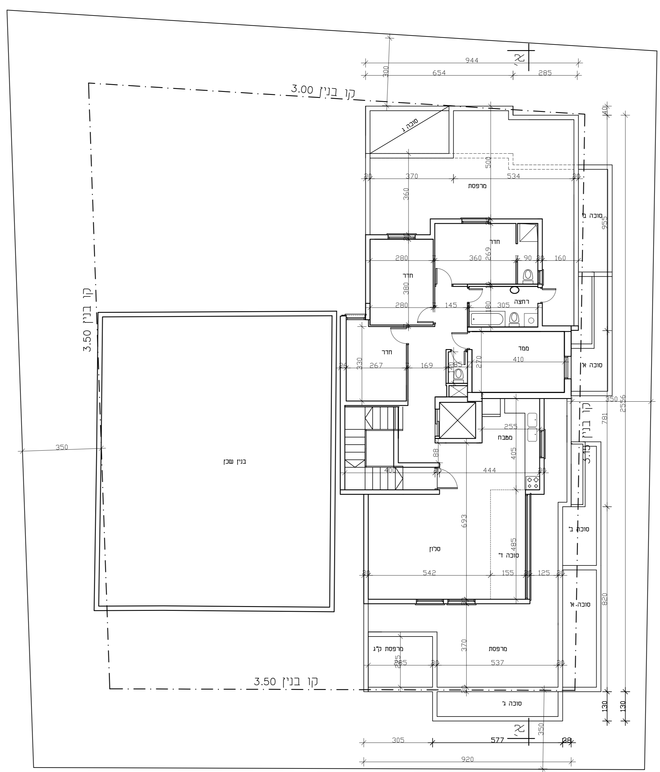
תוכנית קומת הגג ק.ג.מ. 1:100
