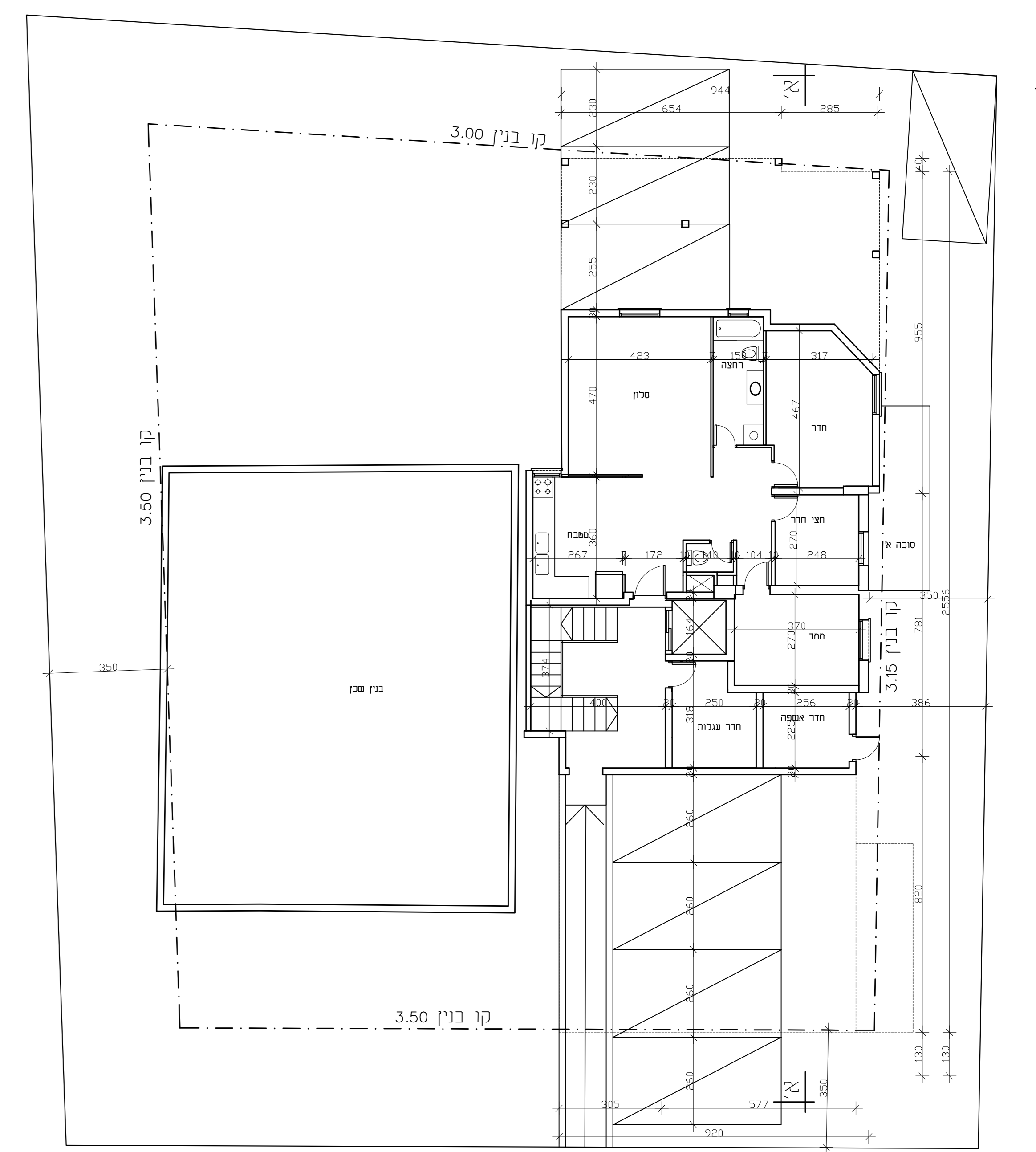
תוכנית קומת ביטה ק.ג.מ. 1:100
