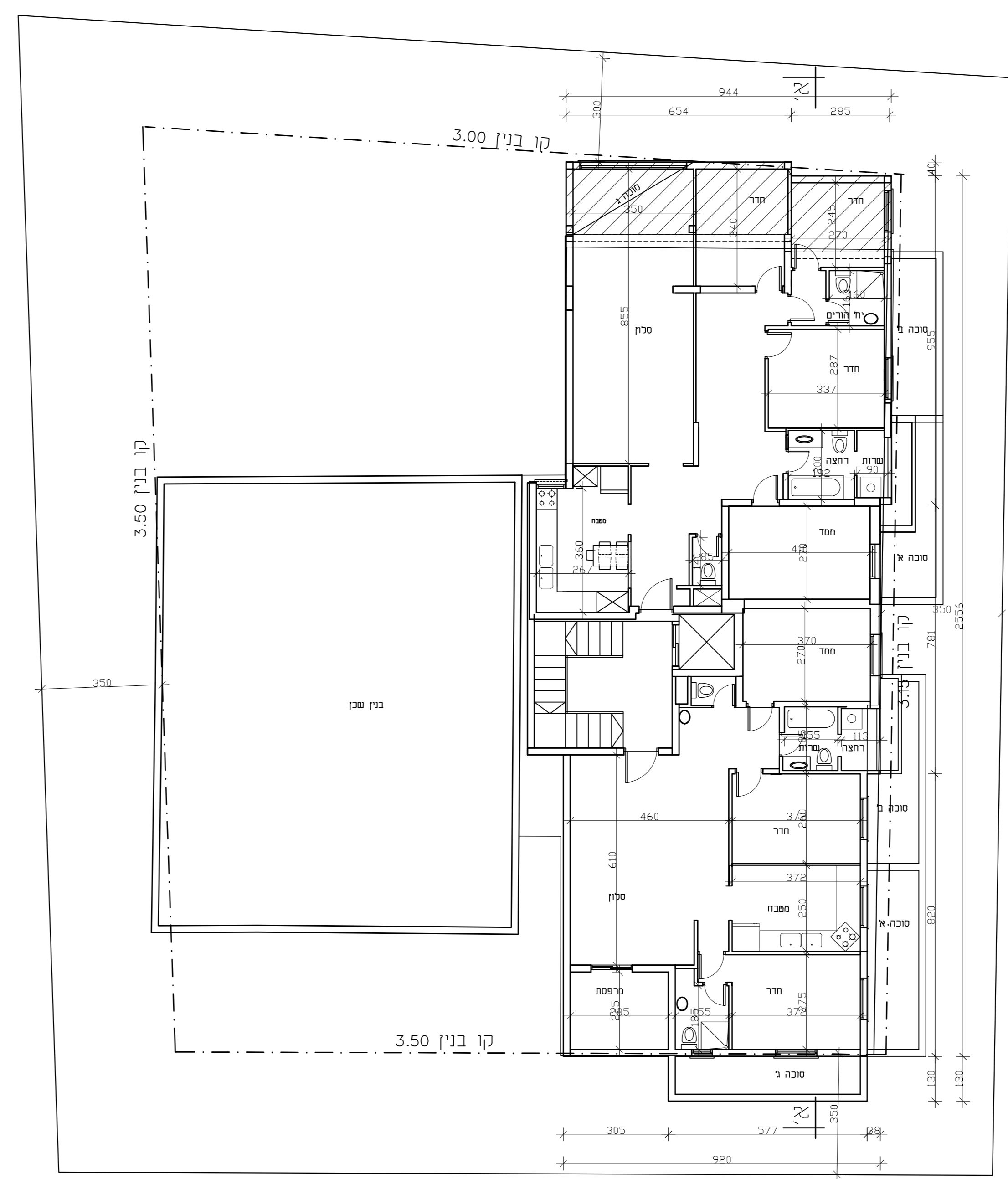
תכנית קומת מי'פוסית ק.ג.מ. 1:100
