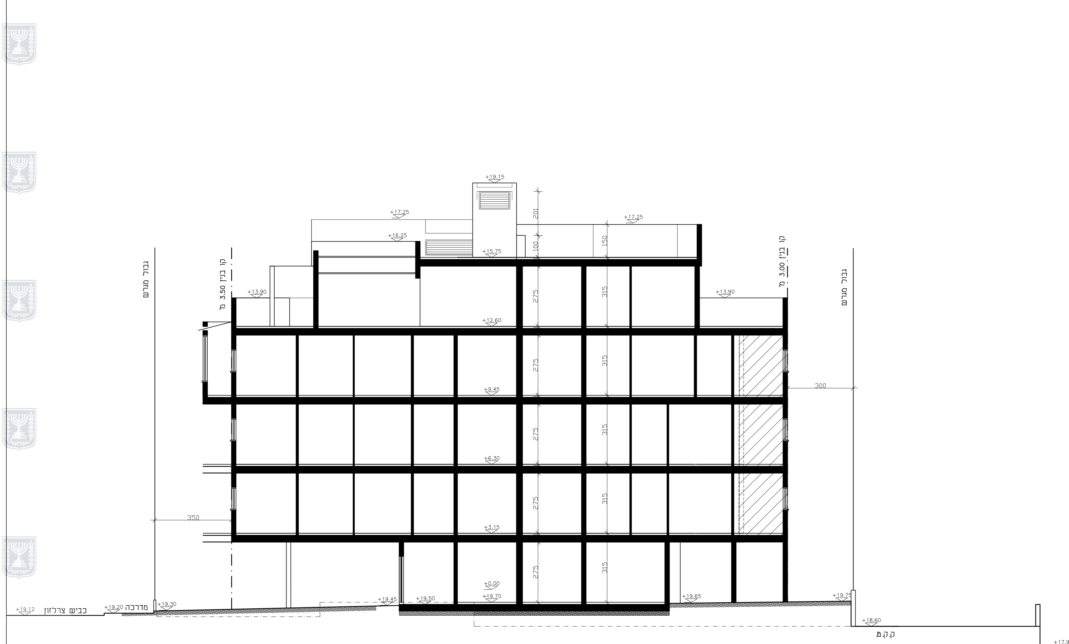
חתך א-א ק.ג.מ. 1:100
