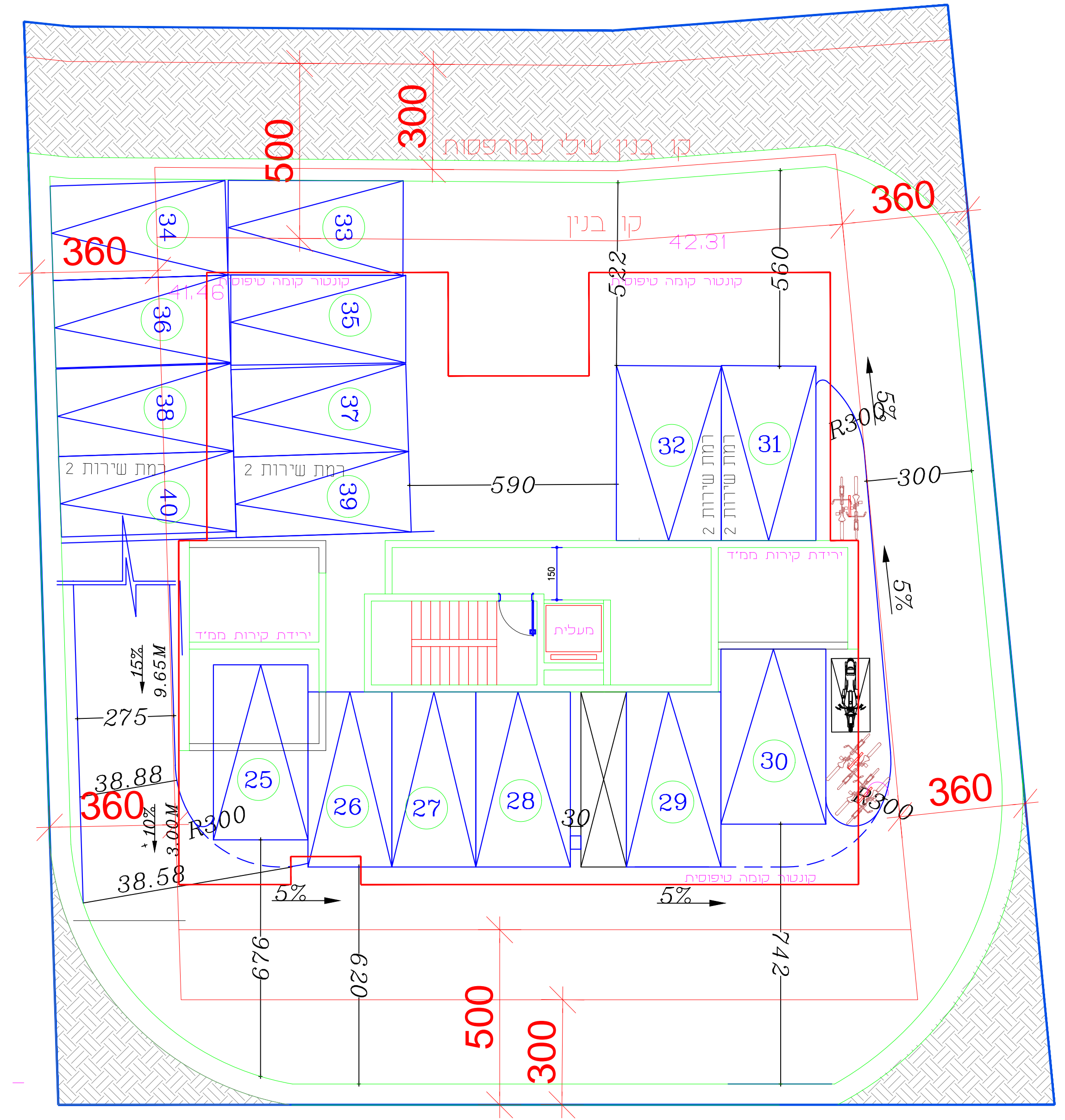
מרתף 3-
