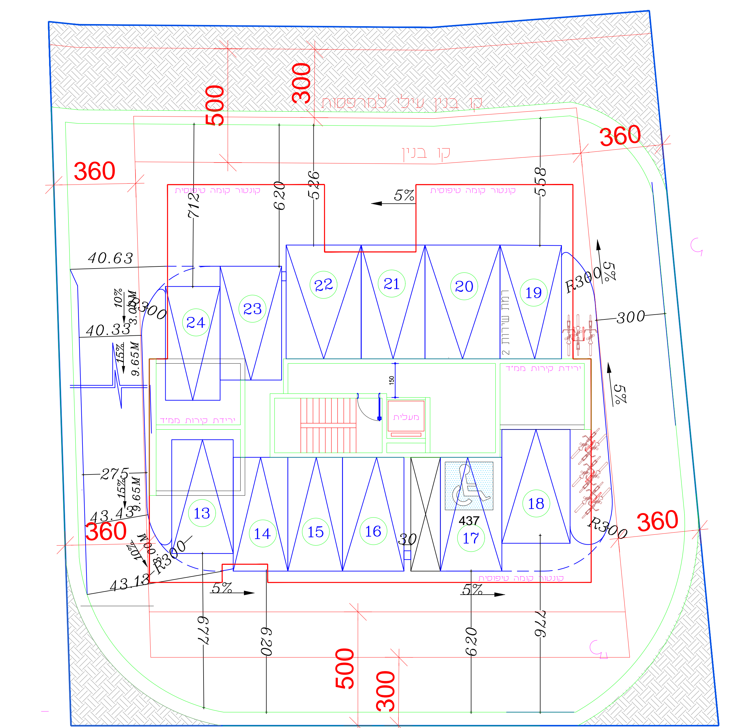
מרתף 2-
