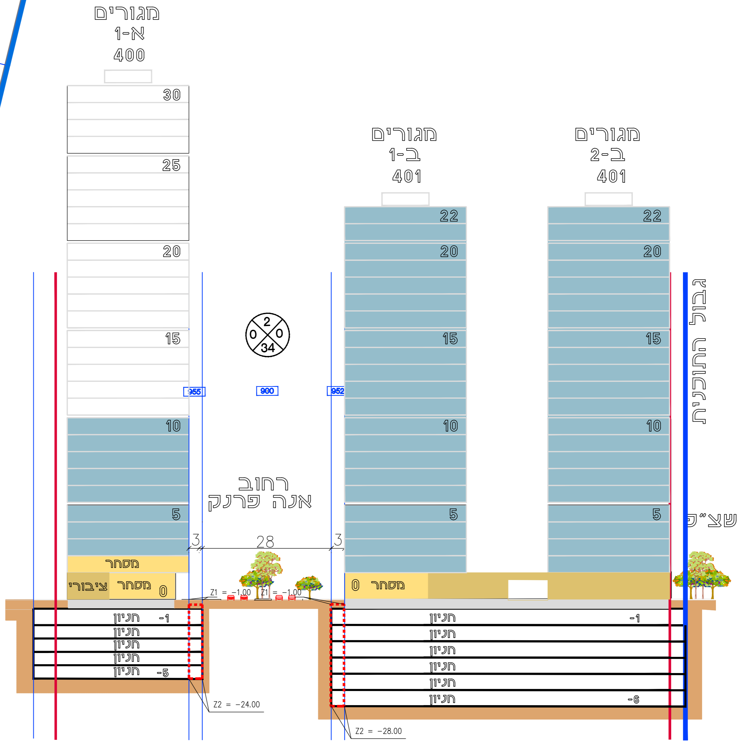
חתך עקרוני קנ"מ 1:500
