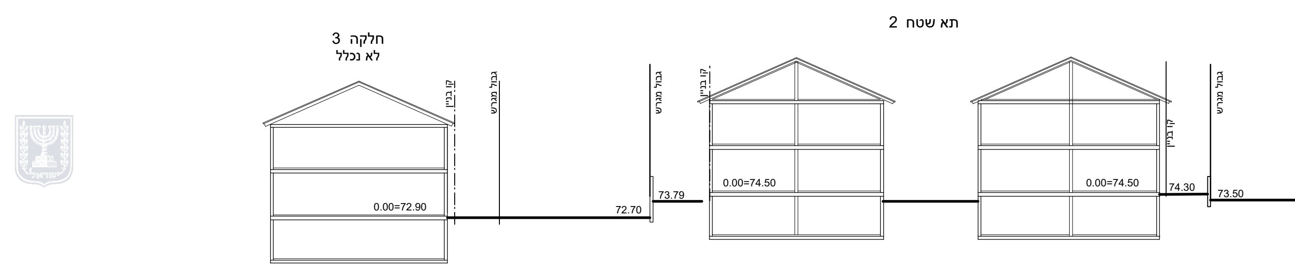
חתך 2-2 קנה מידה 1:250
