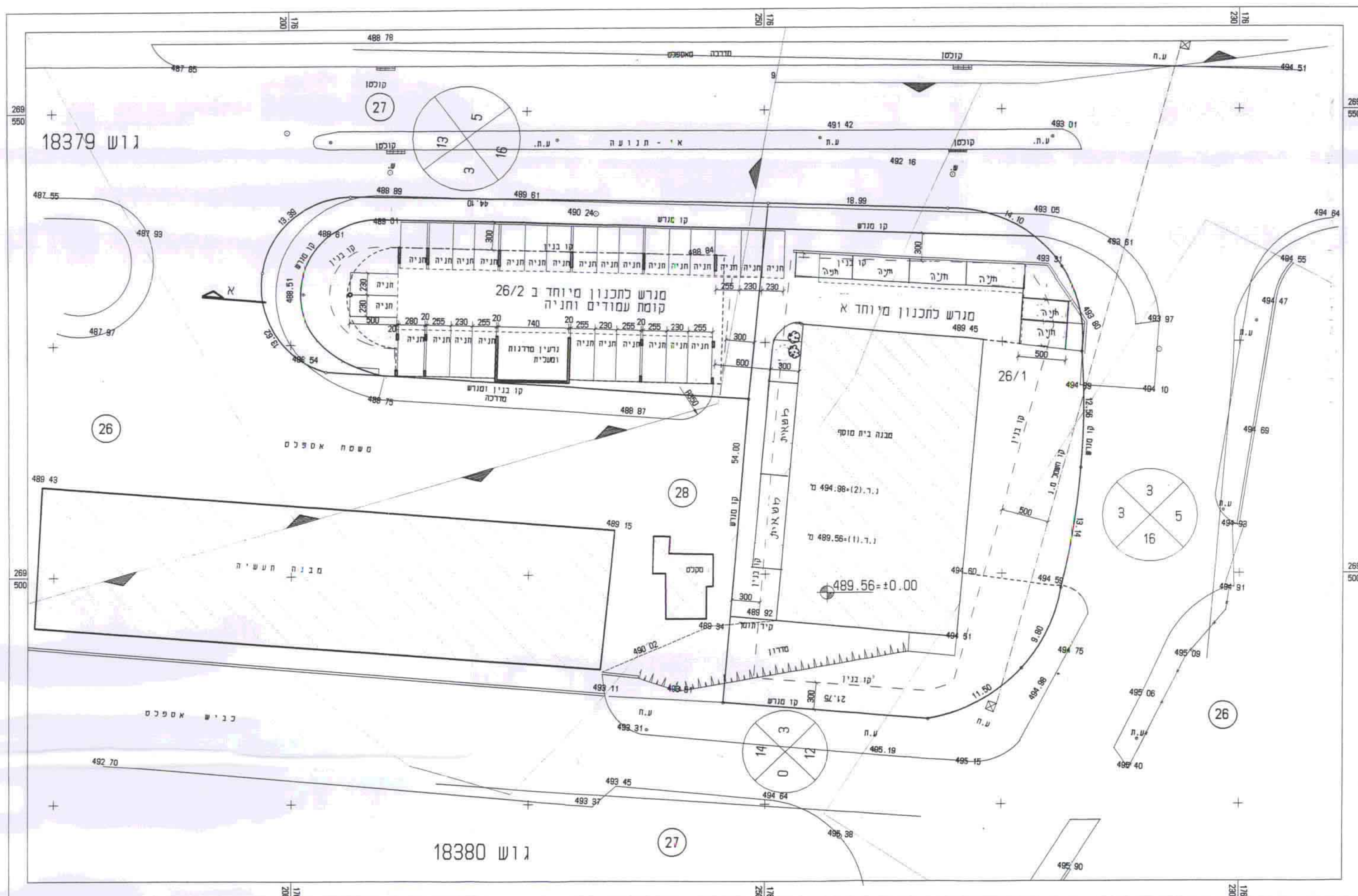
תכנית בינוי קומת קרקע
