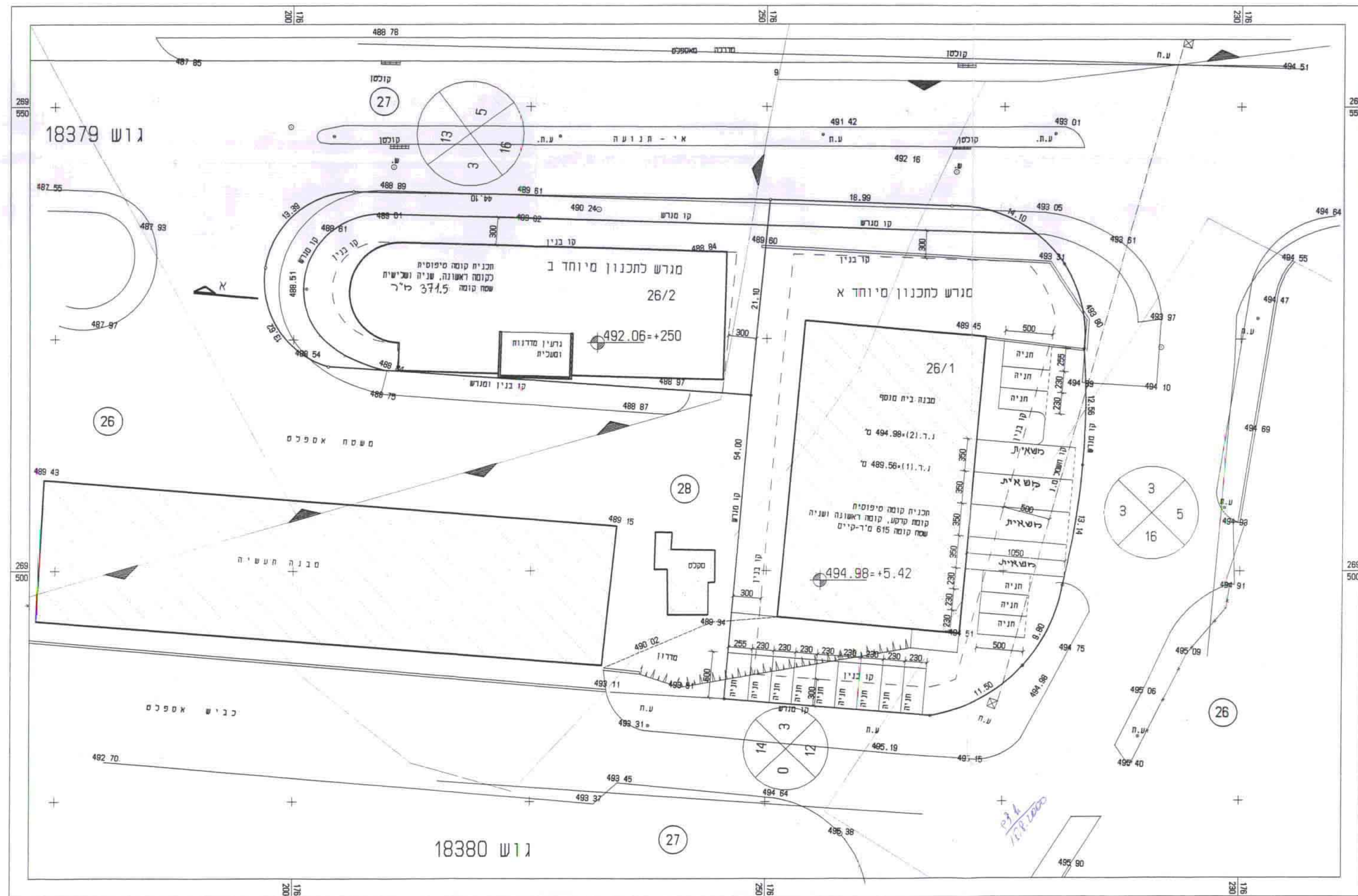
תכנית בינוי קומה ראשונה
