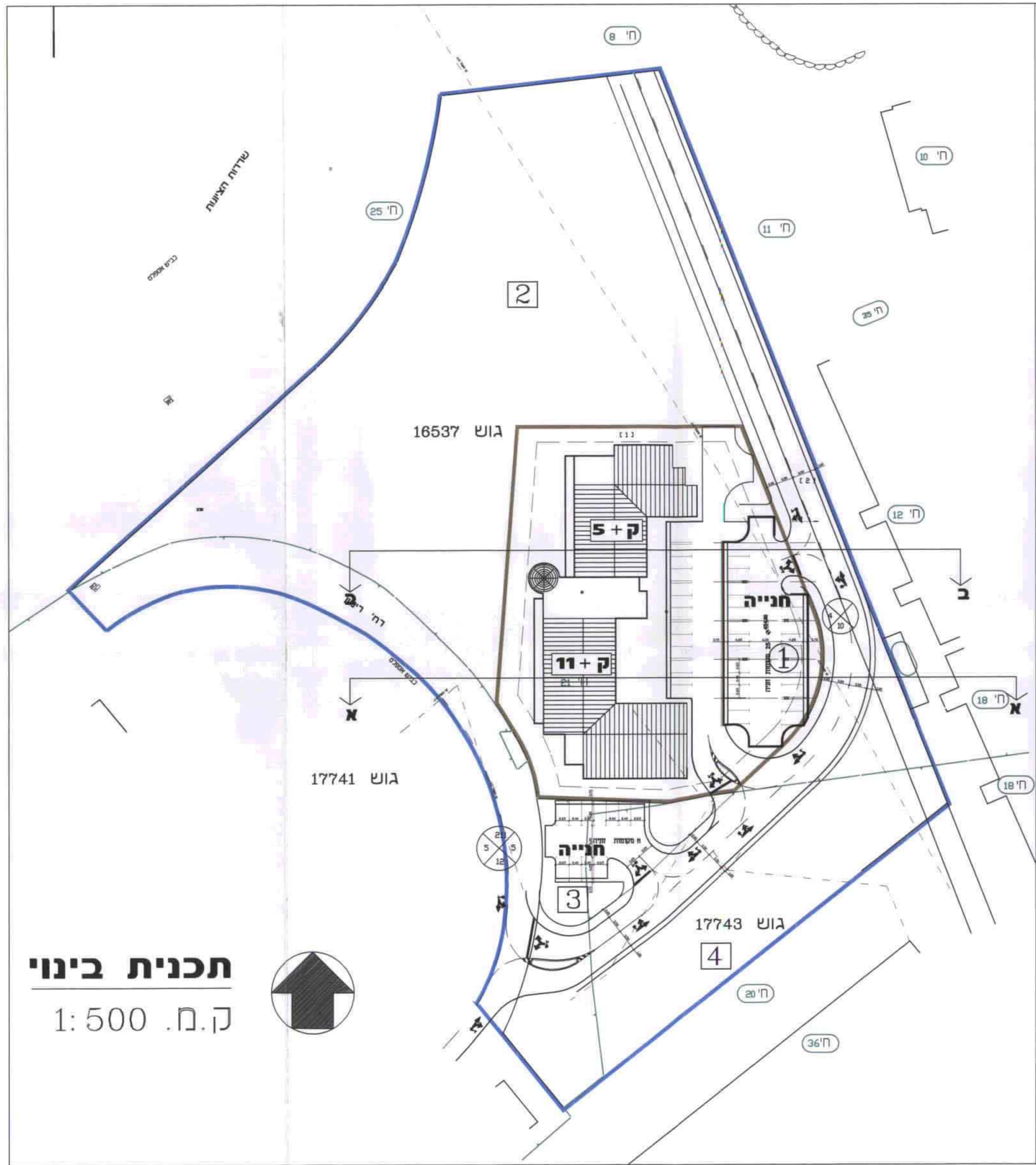
תכנית בינוי אזור משולב 1:500
