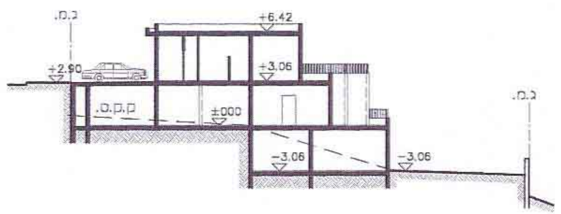
חתך אורך
