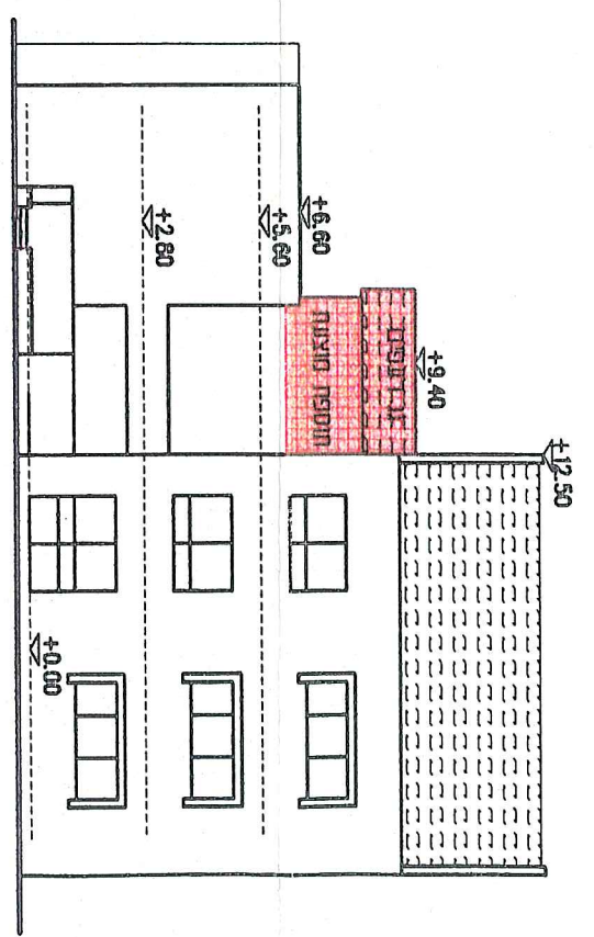
חזית קדמית
