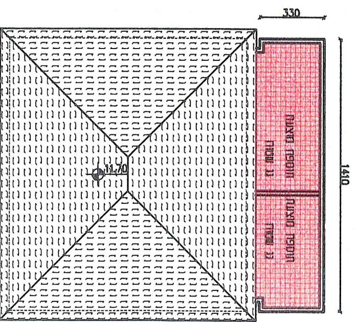
תכנית גומת
