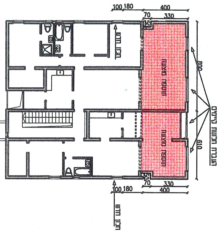
תכנית קומה טיפסית
