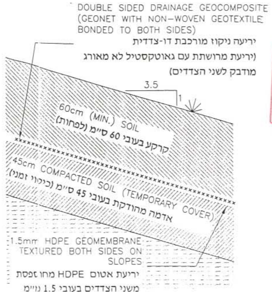
SIDE SLOPES מדרונות צדדים
