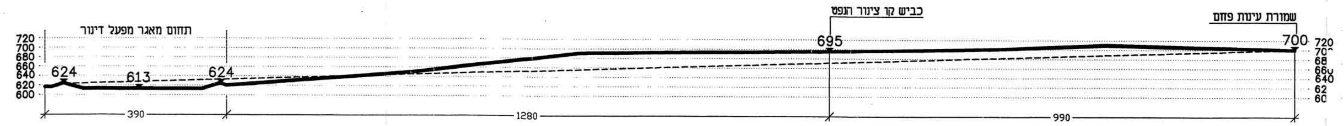
חתך ד-ד
